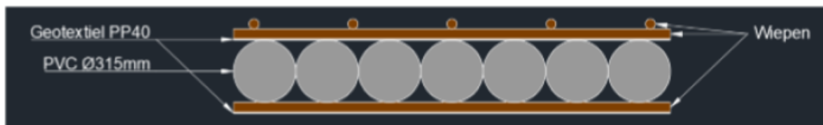
Figuur 1 | Dwarsprofiel
