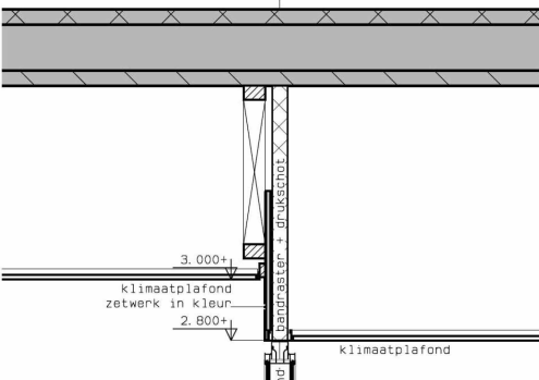
Doorsnede 4
