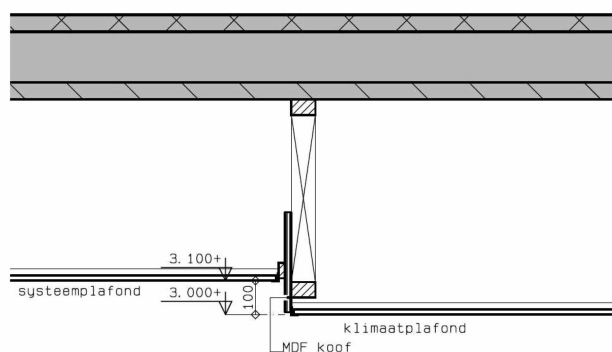
Doorsnede 5
