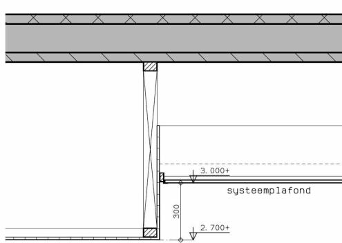
Doorsnede 3
