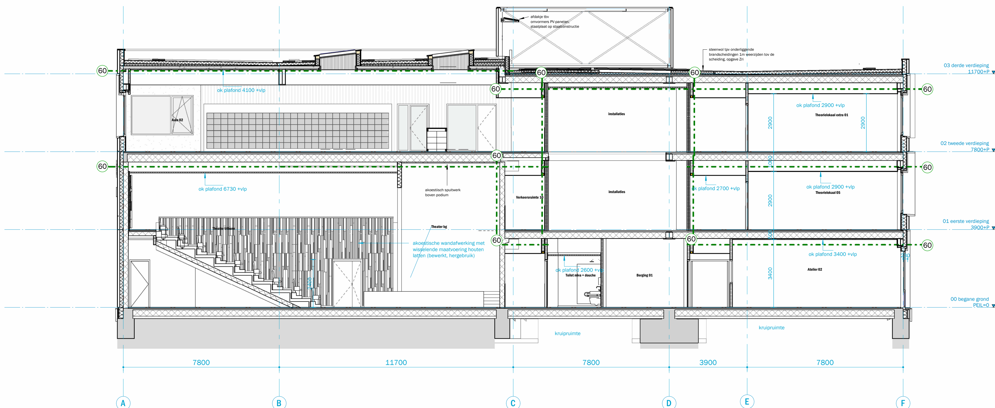
doorsnede I
