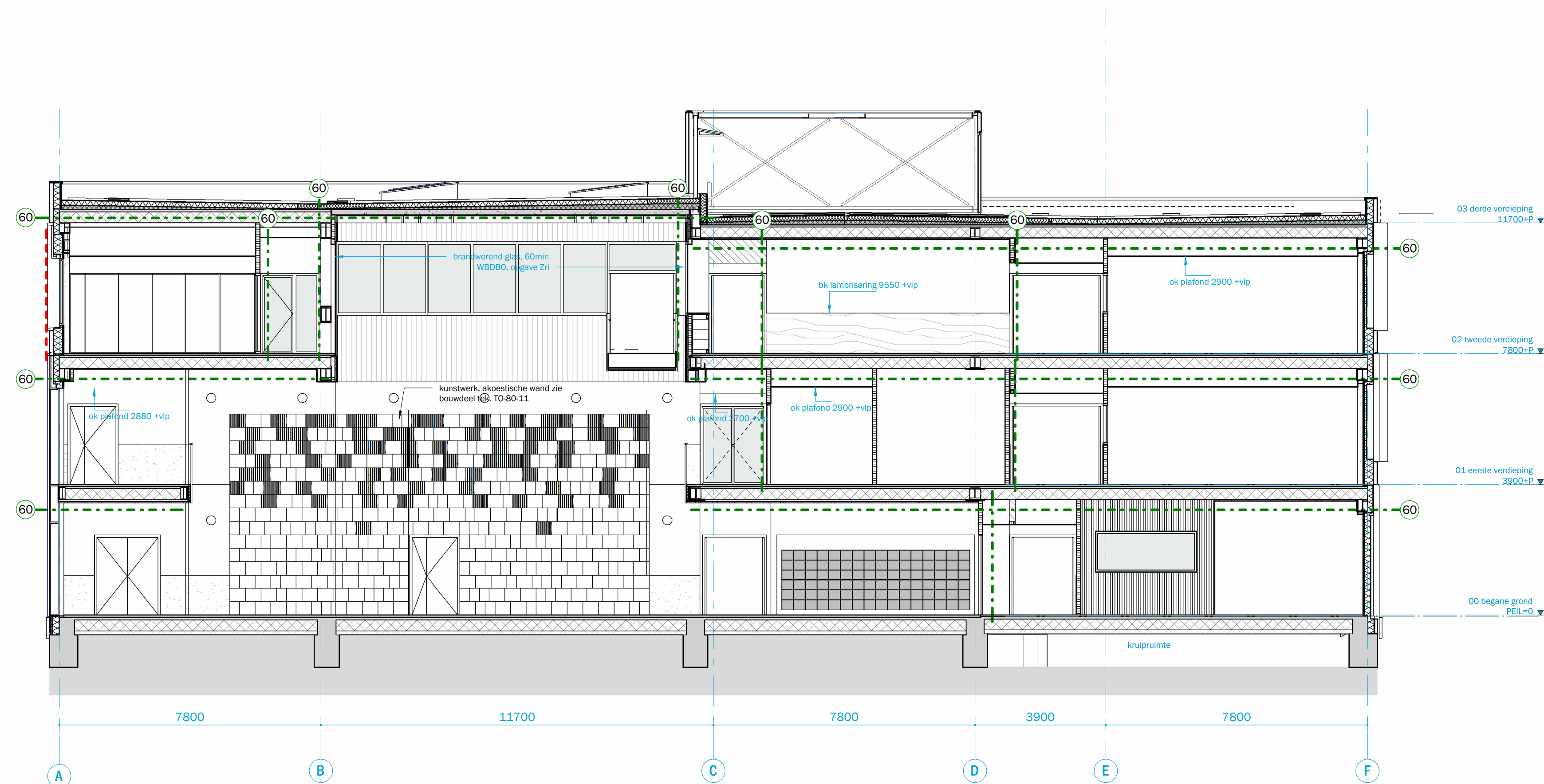
doorsnede H
