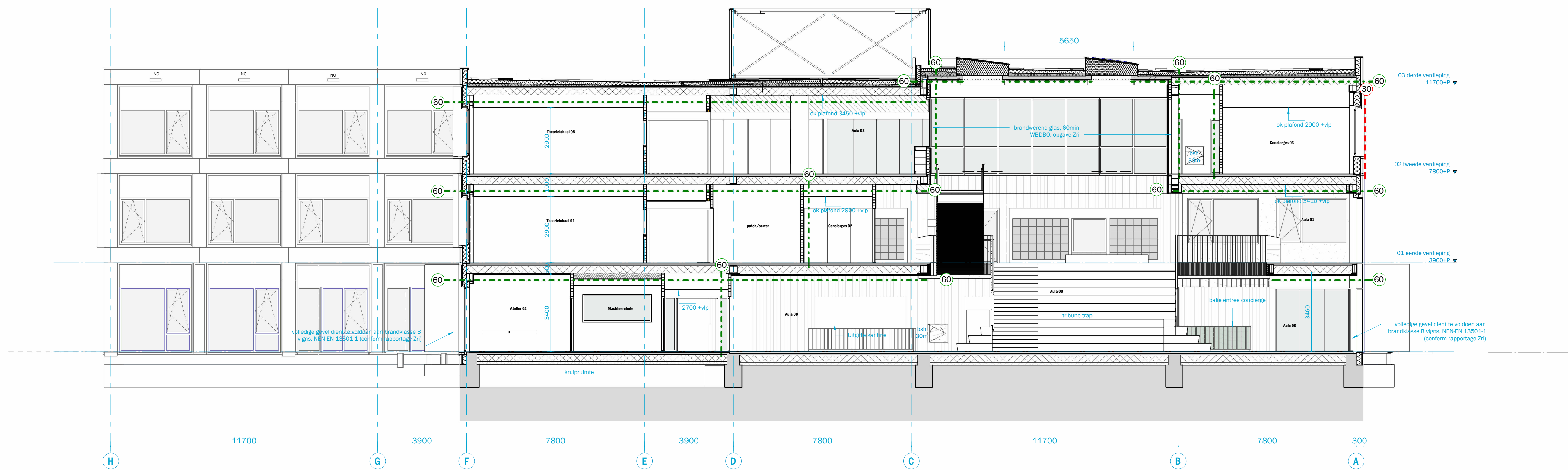
doorsnede G
