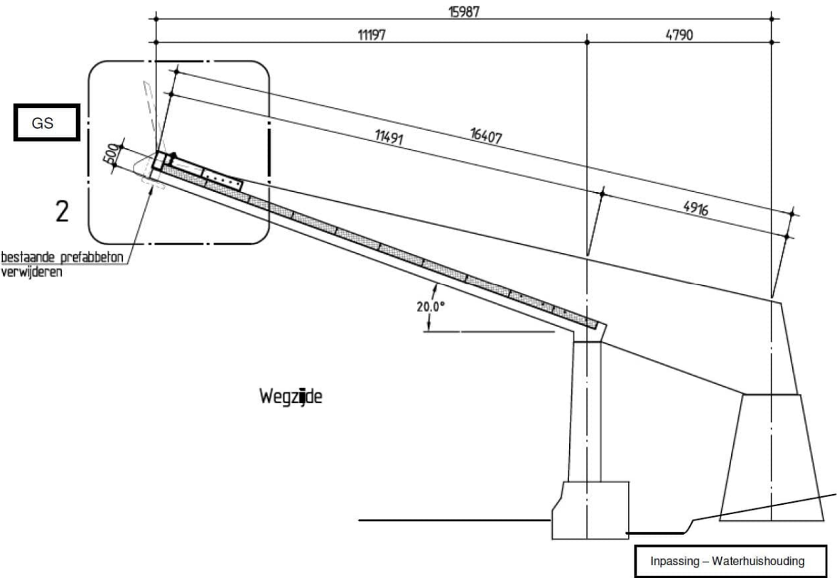
Dwarsdoorsnede luifel
