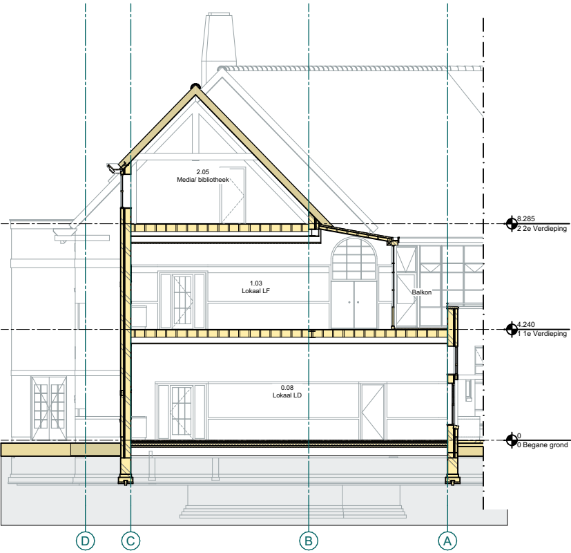
Doorsnede B-B
