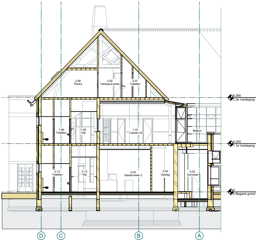
Doorsnede C-C
