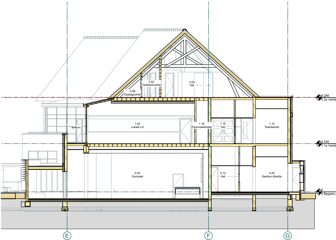
Doorsnede D-D
