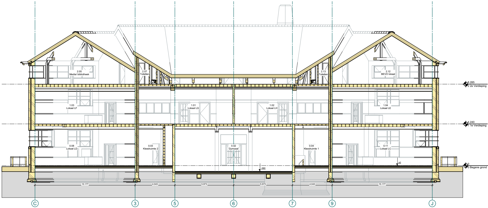
Doorsnede A-A
