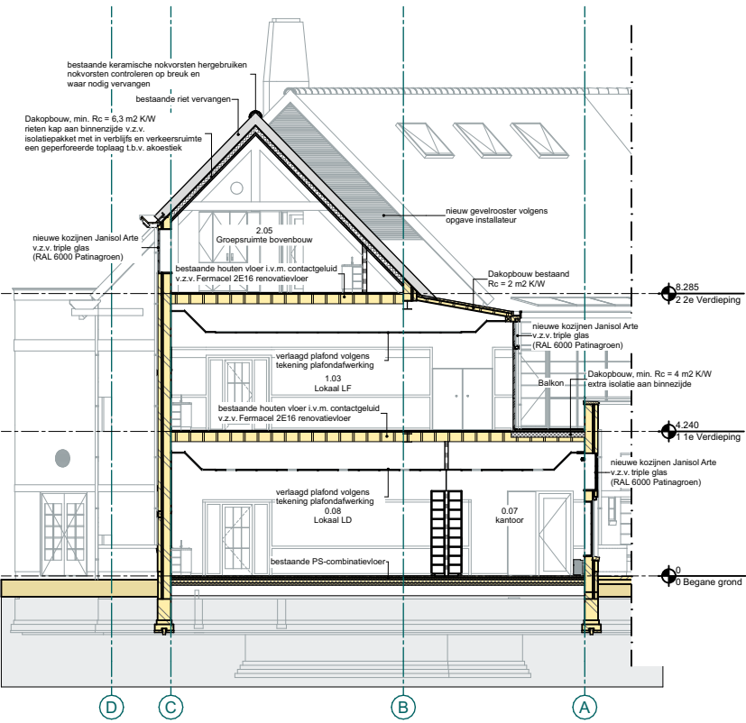
Doorsnede B-B
