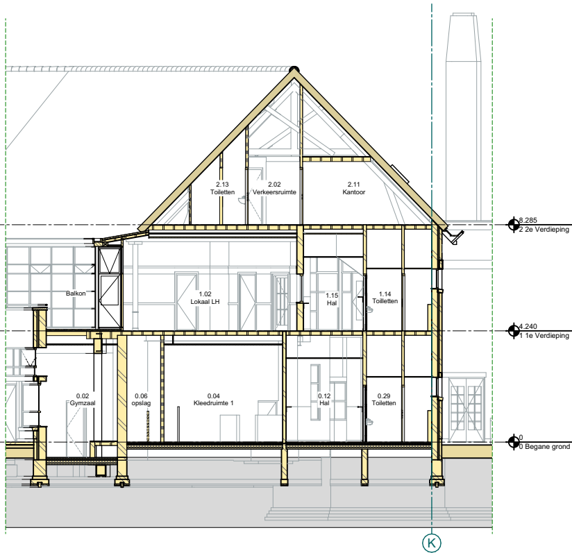
Doorsnede E-E
