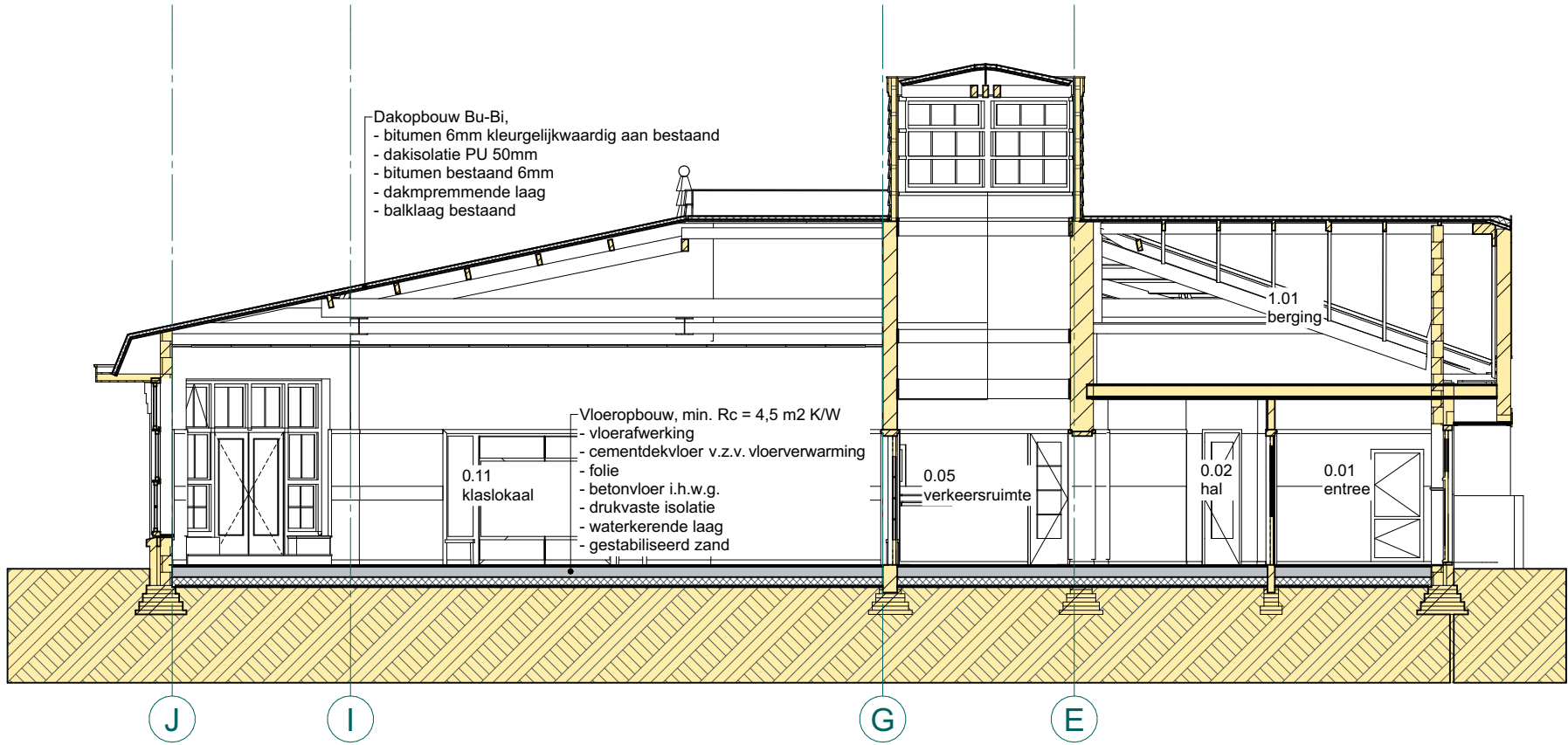
Doorsnede A-A
