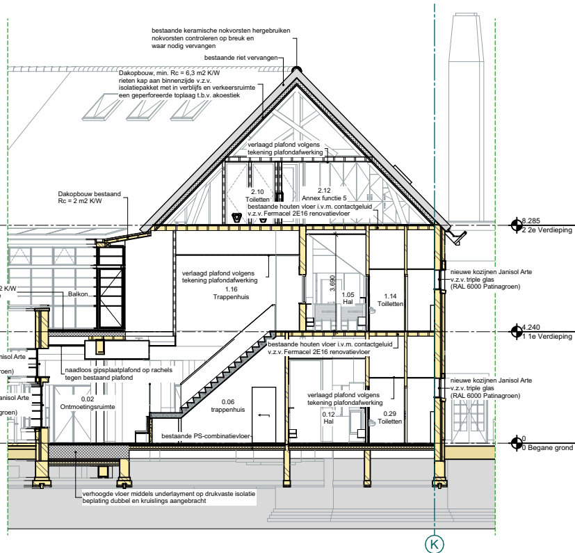
Doorsnede E-E
