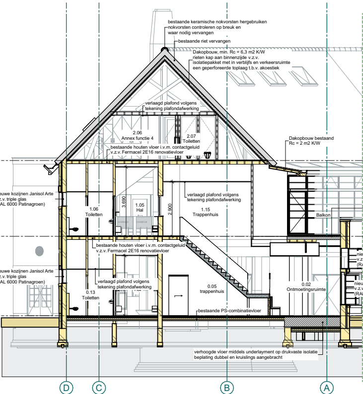
Doorsnede C-C
