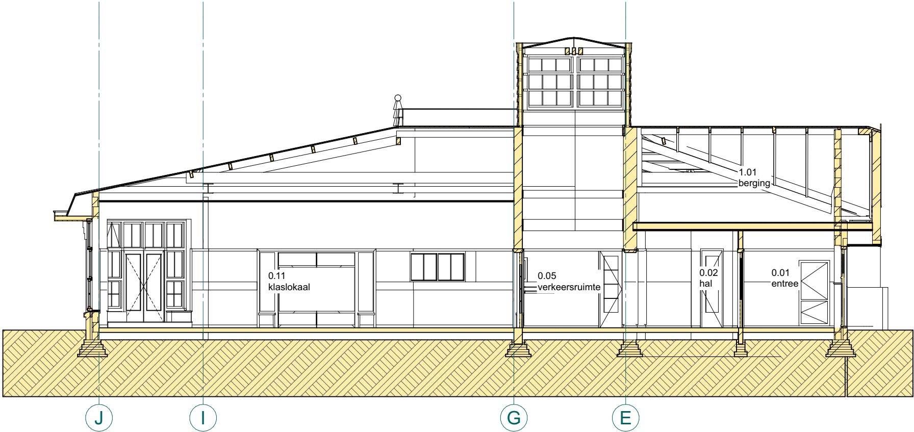
Doorsnede A-A
