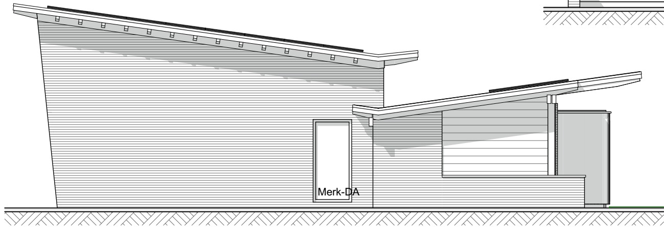
Rechtergevel
