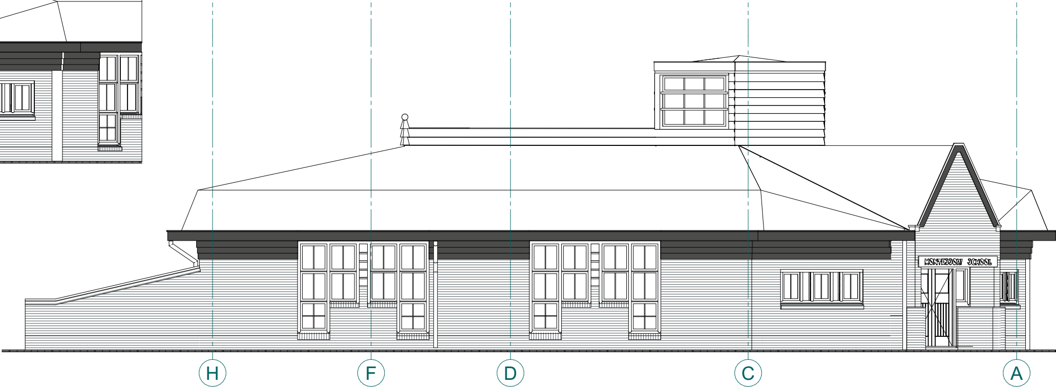
Gevel 03
