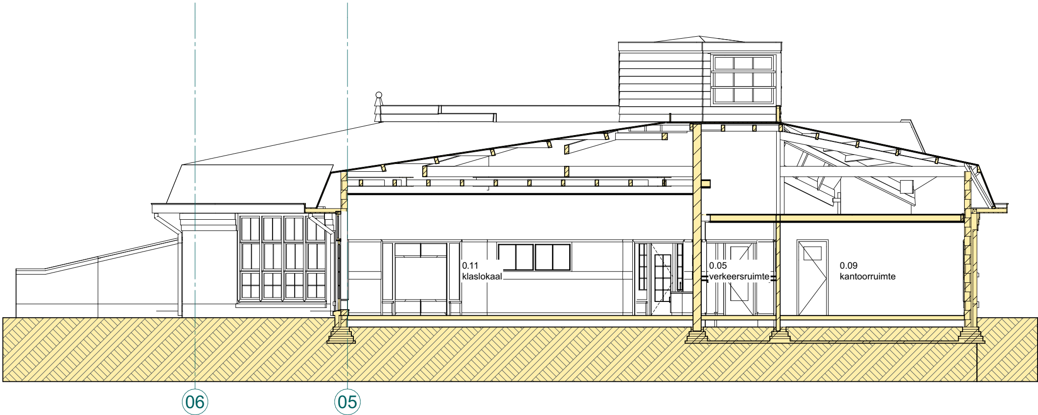
Doorsnede A-A
