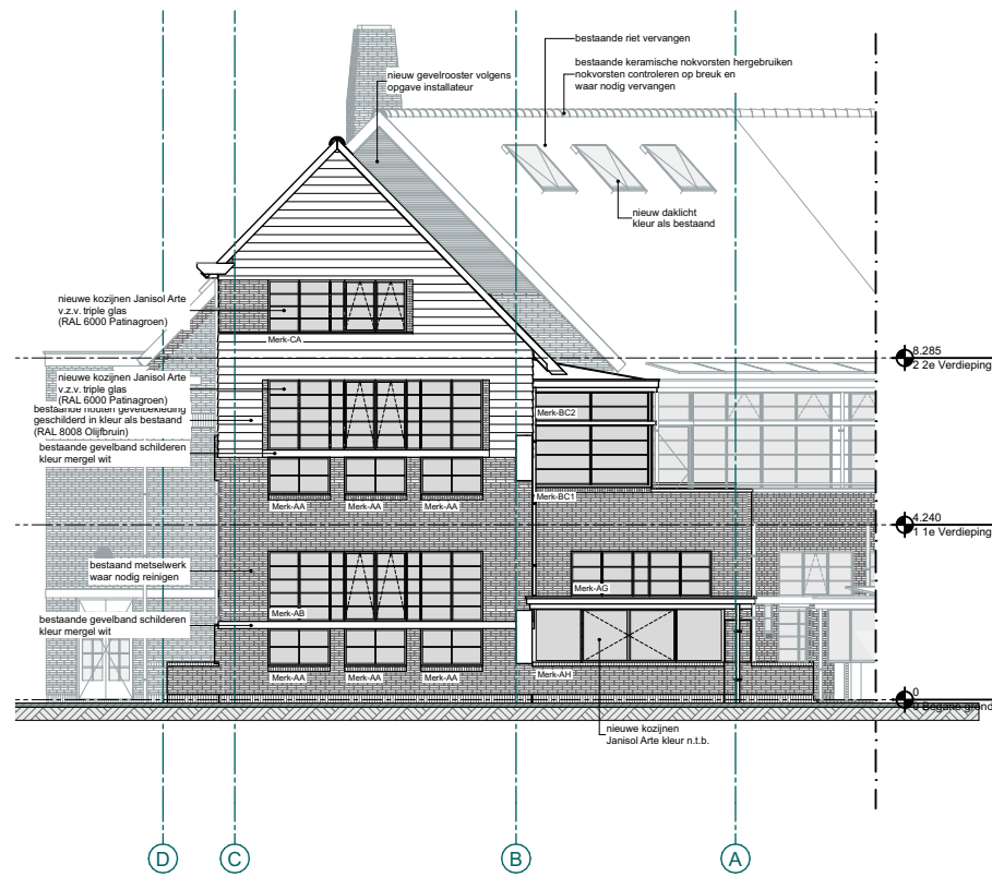
Linker zijgevel
