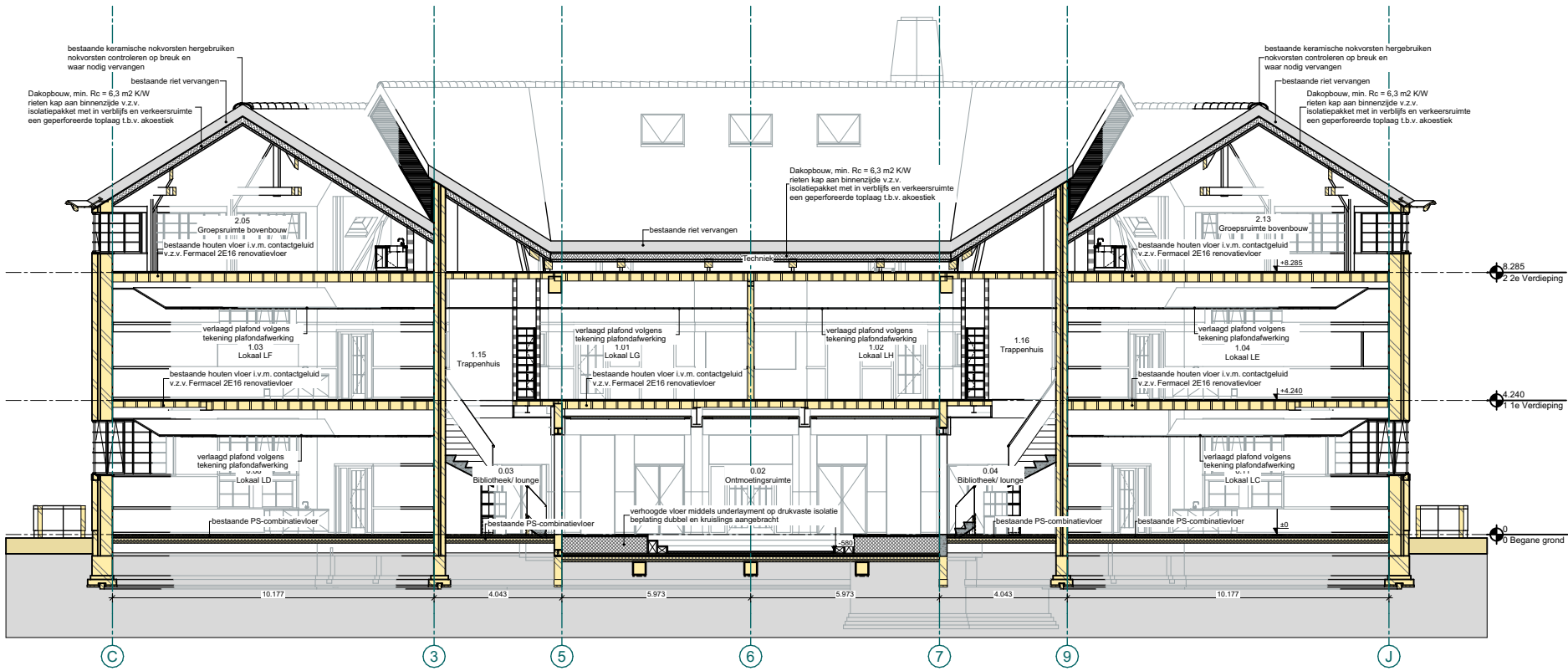
Doorsnede A-A
