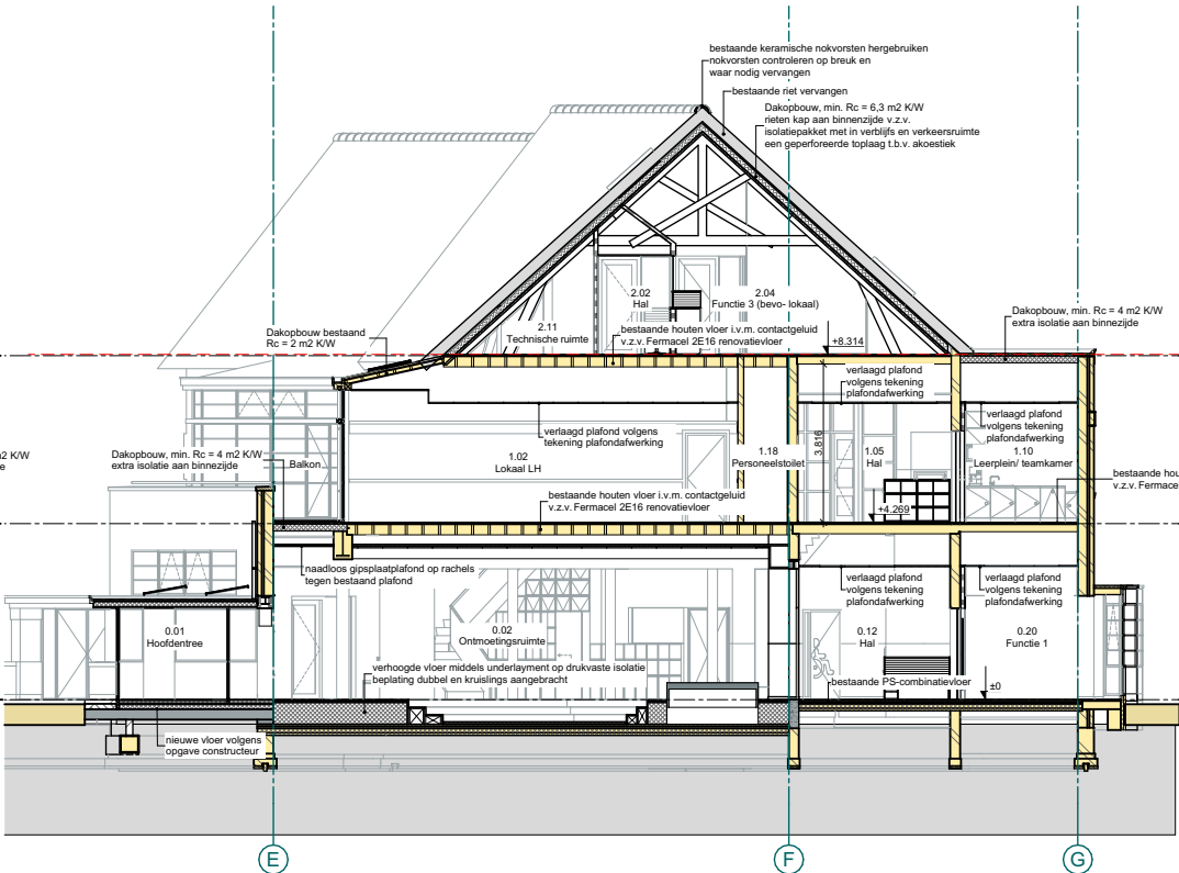
Doorsnede D-D
