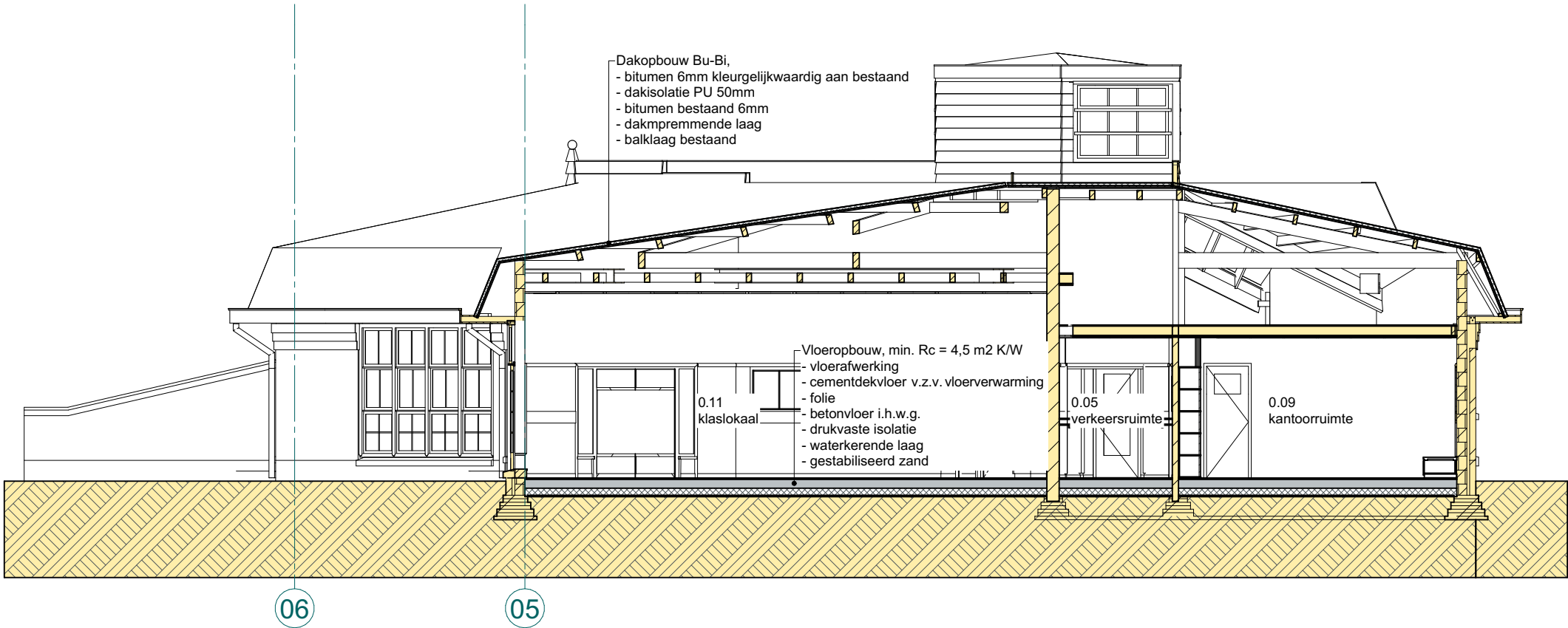
Doorsnede A-A
