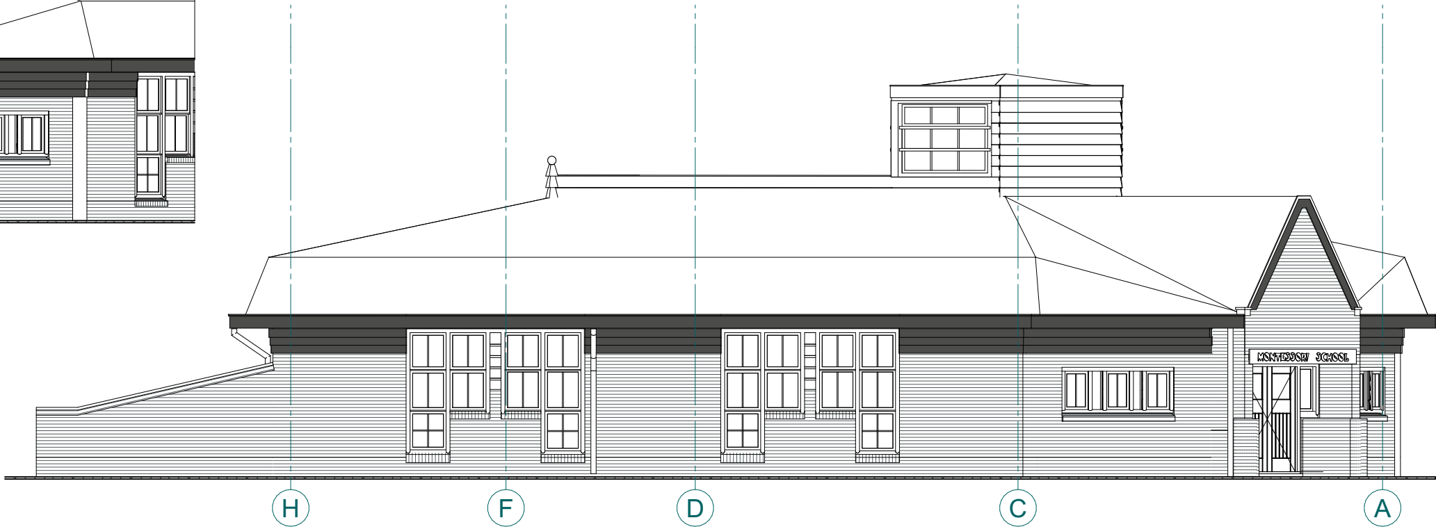
Gevel 03
