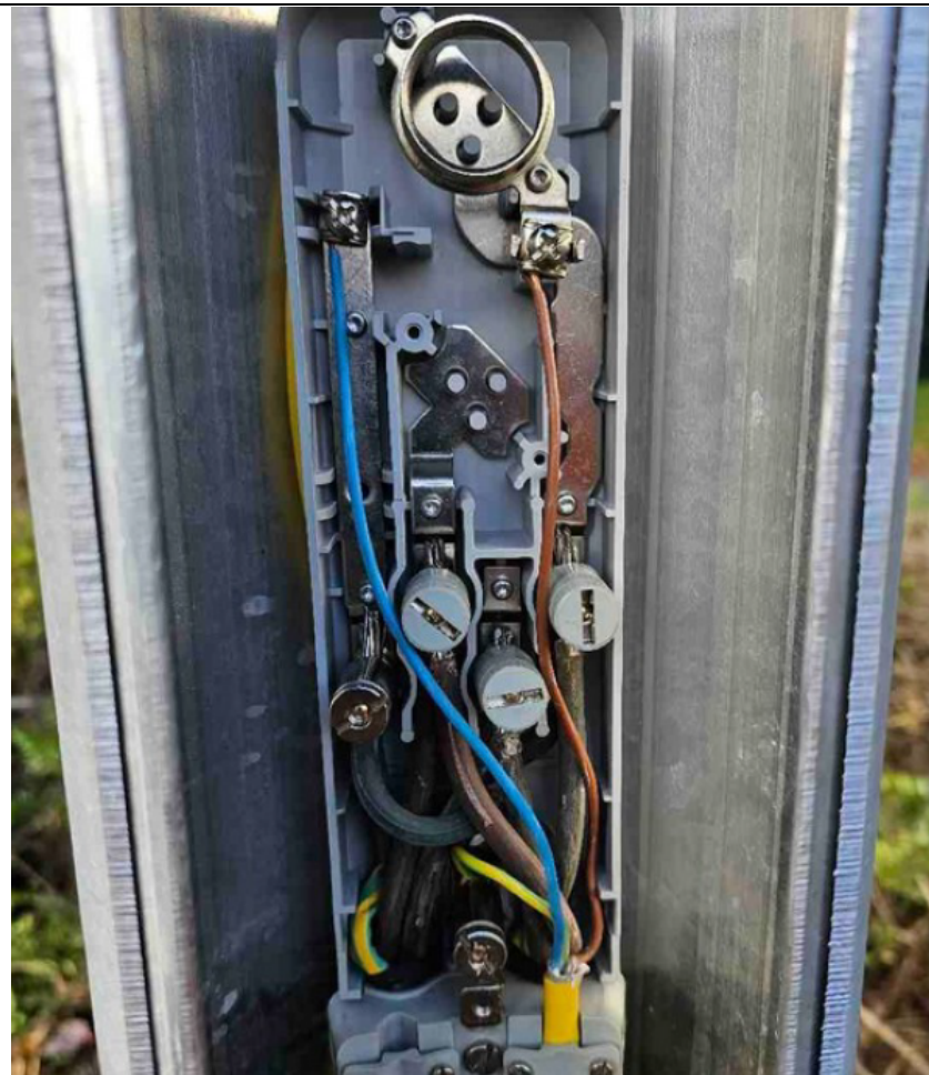
Foto nieuwe situatie, lichtmast voorzijde met lichtmastnummer leesbaar
