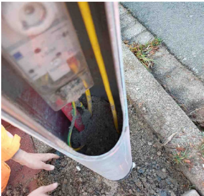
Foto nieuwe situatie, lichtmast zijkant
