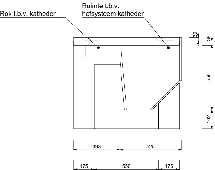
Doorsnede C
