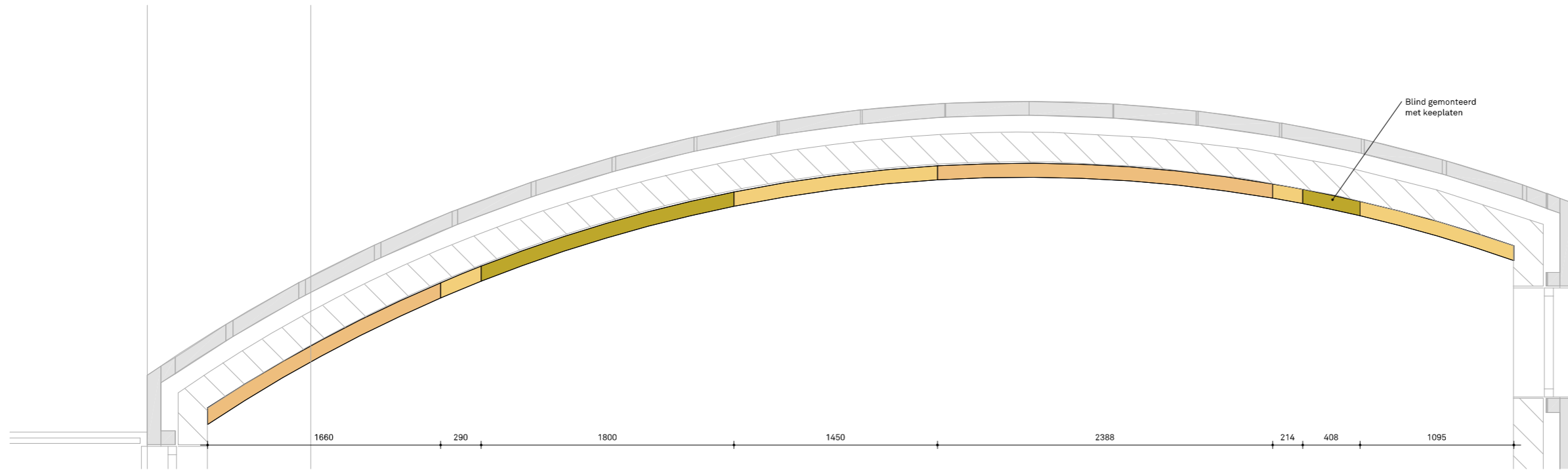
1 Bovenaanzicht 1:25
