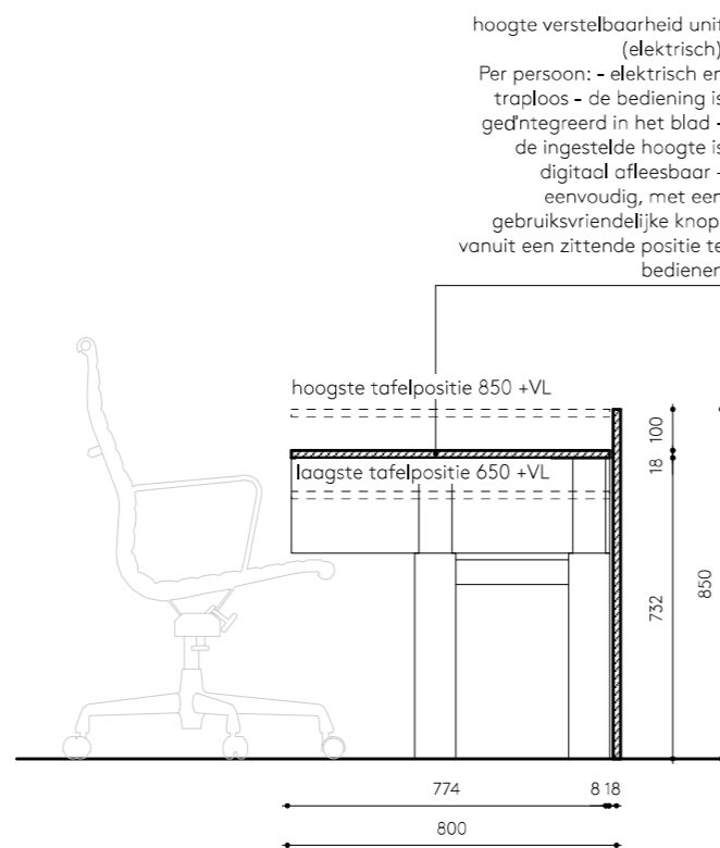
doorsnede b-b schaal: 1:20
