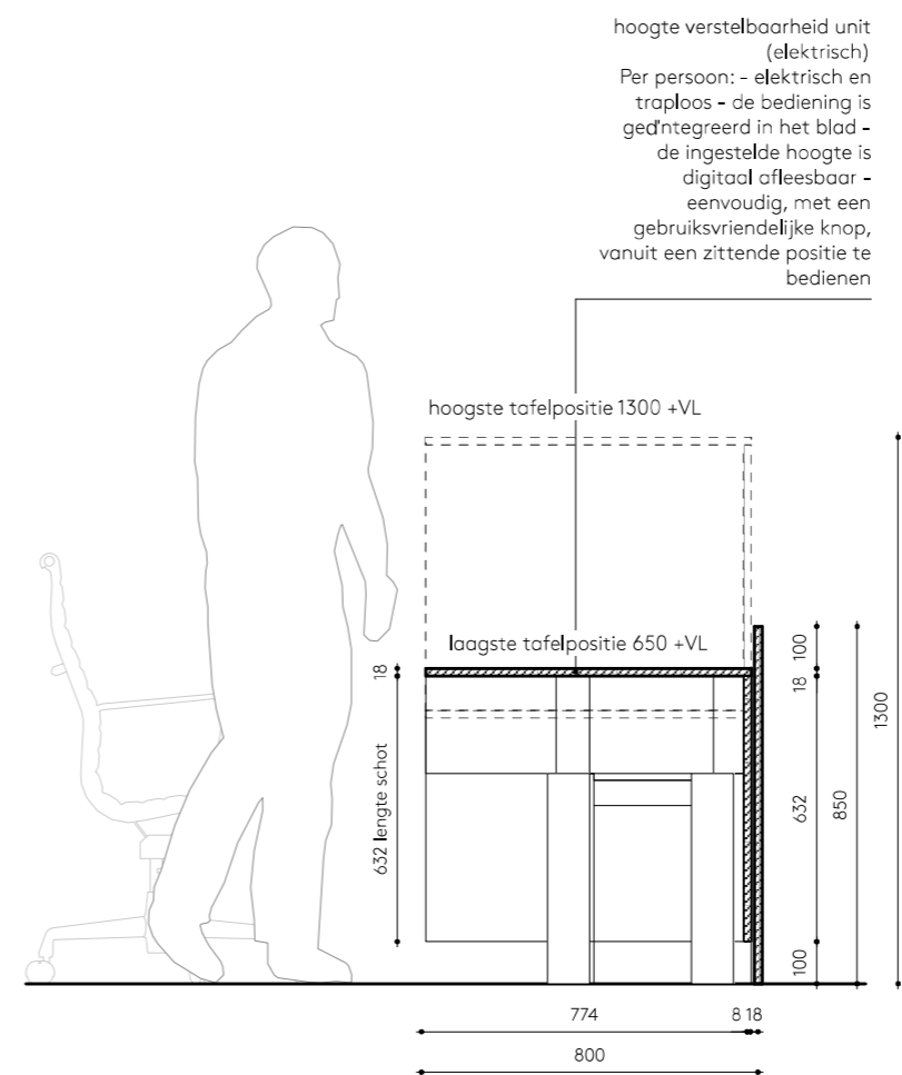
procespartij tafel advocaat schaal: 1:20
