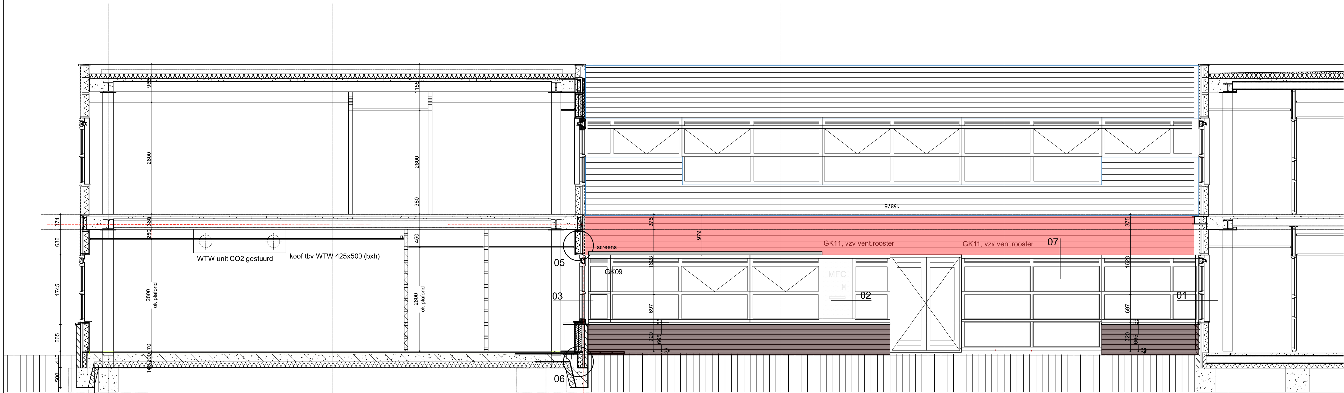
DOORSNEDE-BINNENGEVEL westzijde
