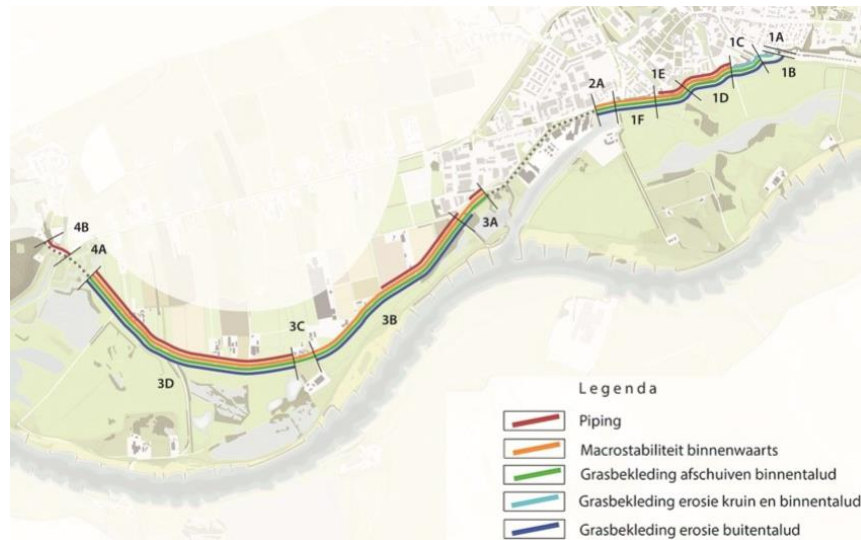
Figuur 7 Faalmechanismen Grebbedijk per dijkvak
