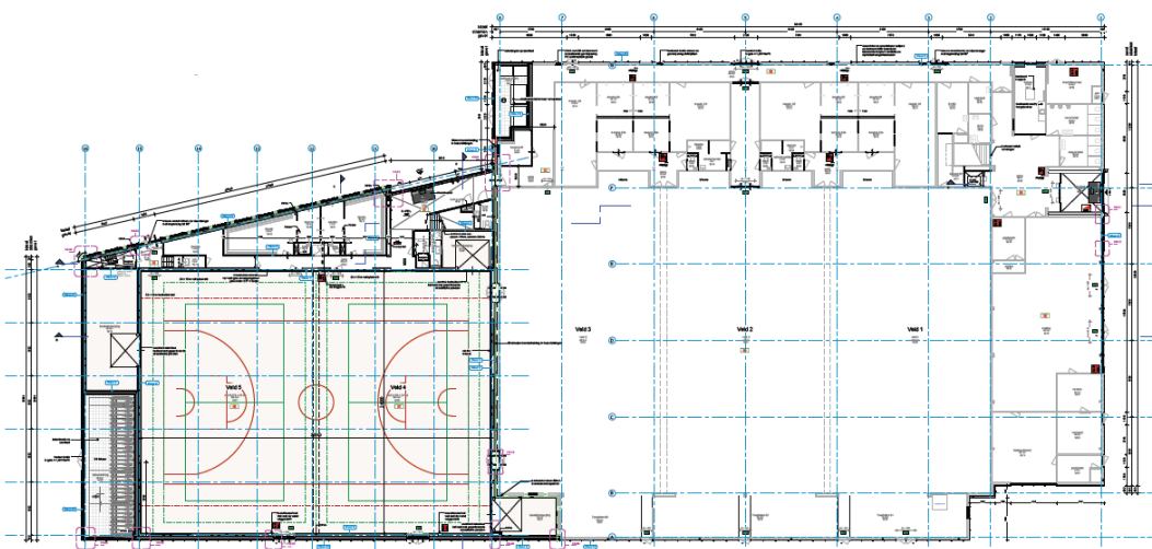
Plattegrond nieuwe situatie
