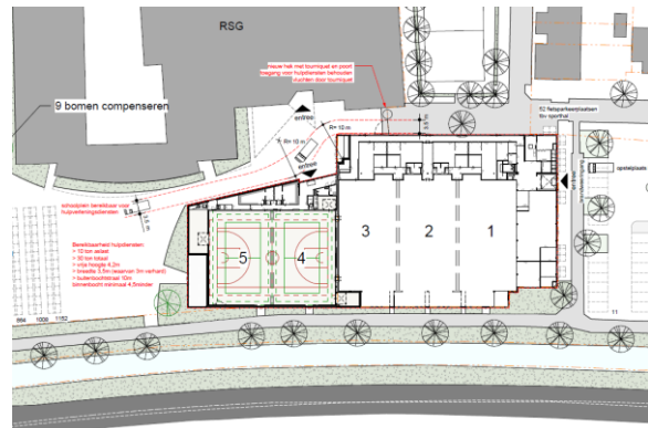
Situatie nieuwe situatie
