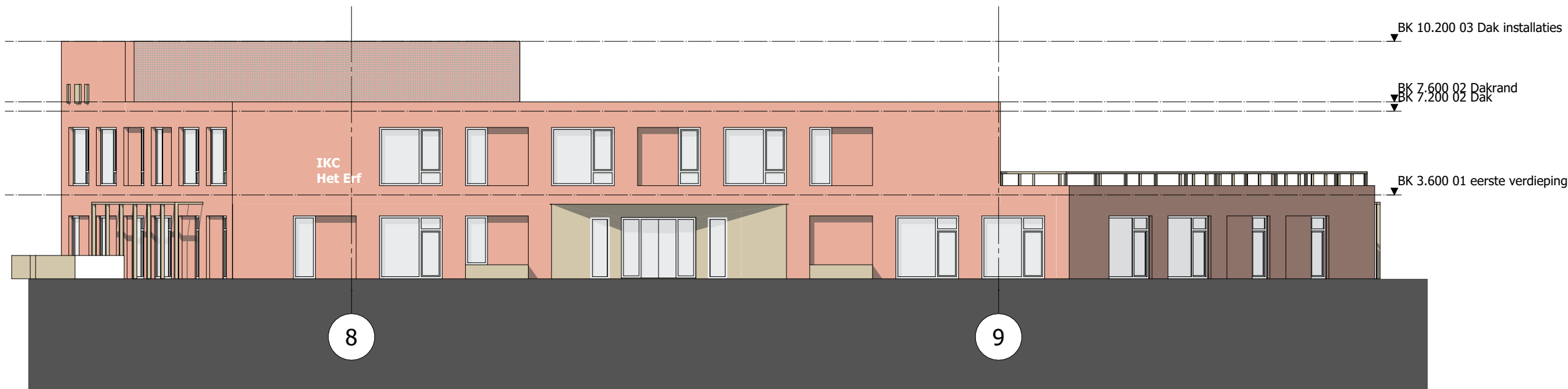
Noordgevel
