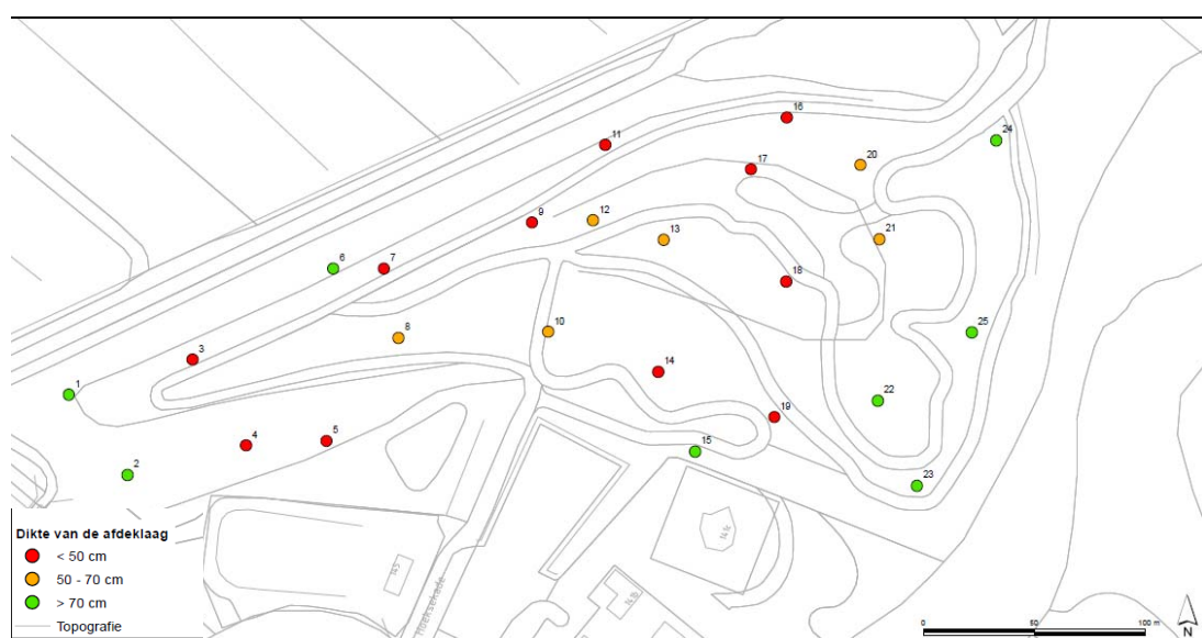
Figuur 2.2 Afdeklaagdikte in categorieën
