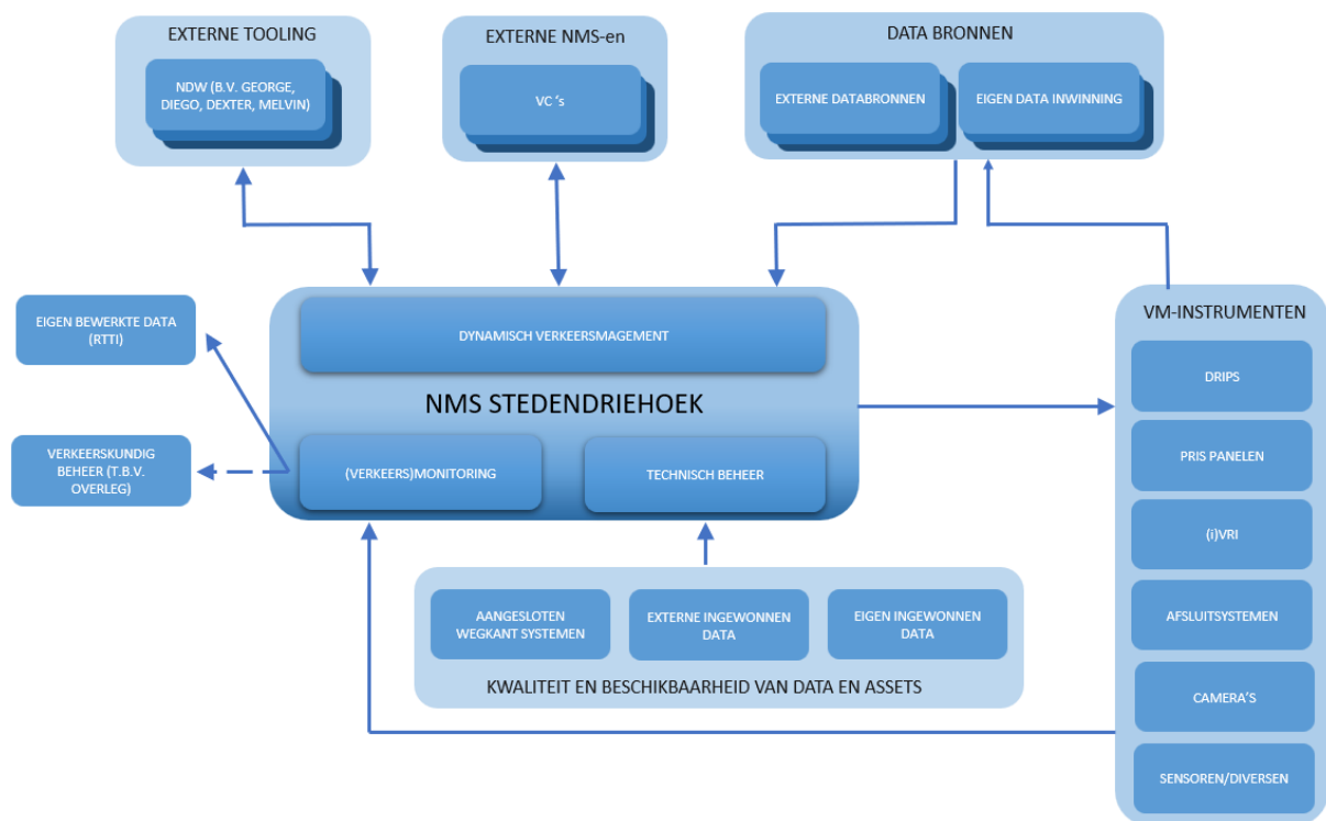
Figuur 1: Globale NMS architectuur
