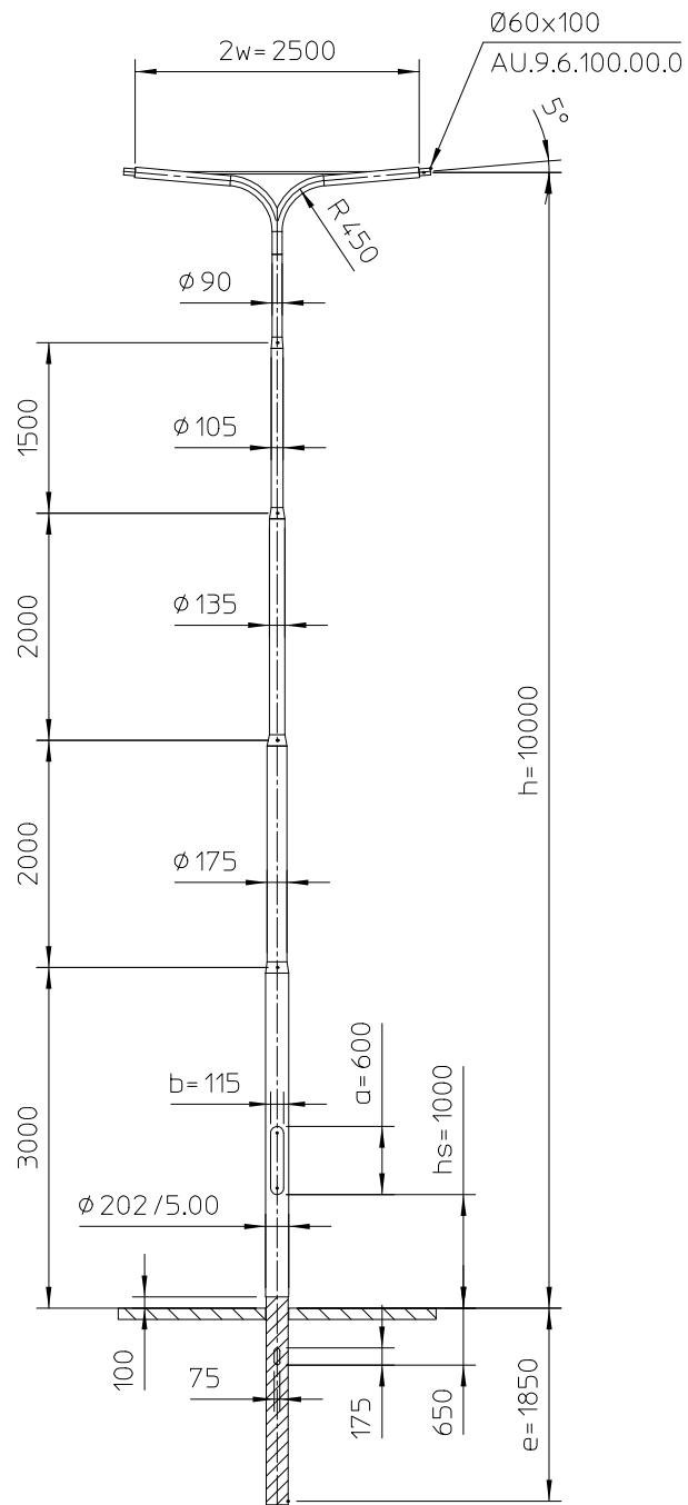
Demontabele uithouder HDPE geïsoleerd grondstuk, vlg's tekening HDPE202.2570.01
