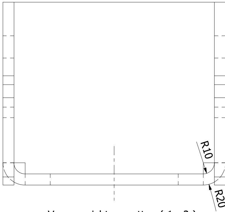
Vooraanzicht na zetten ( 1 : 2 )
