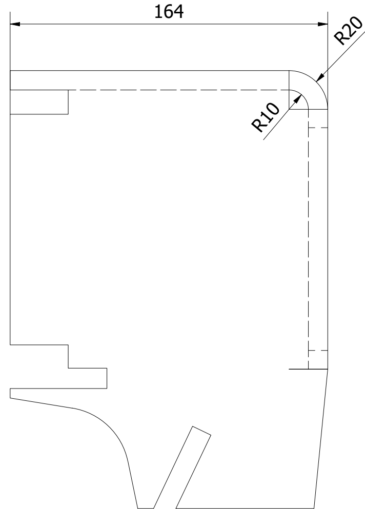
Zijaanzicht na zetten ( 1 : 2 )
