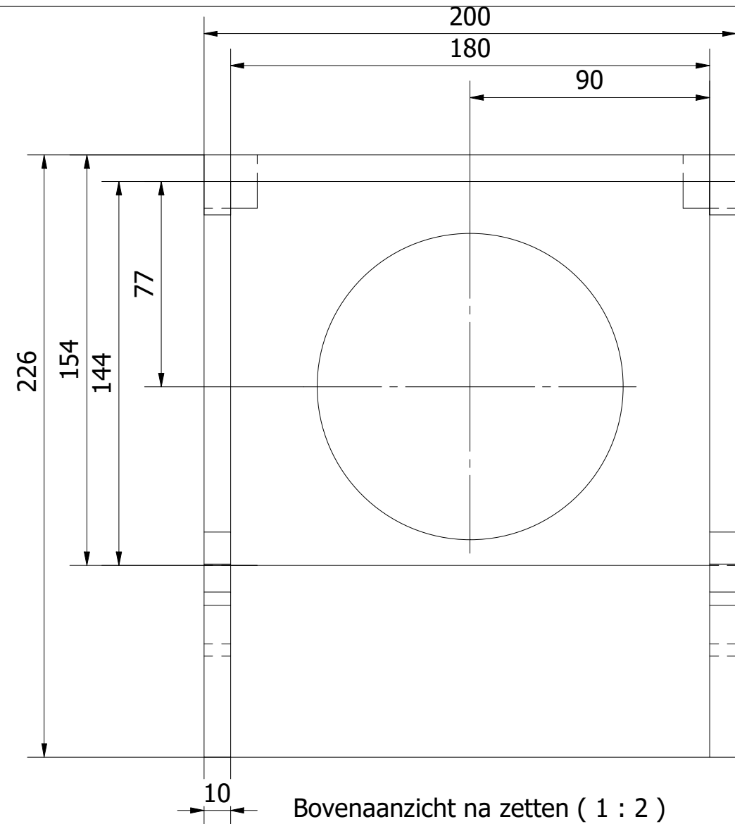
Bovenaanzicht na zetten ( 1 : 2 )
