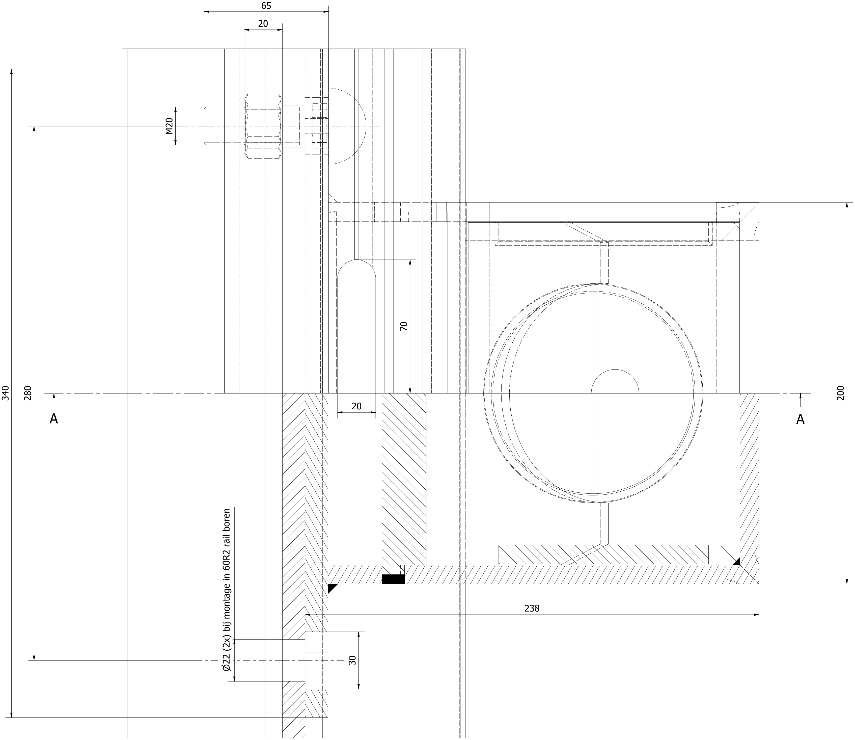
Bovenaanzicht, uitgebroken ter hoogte bolkopbouten ( 1 : 1 )
