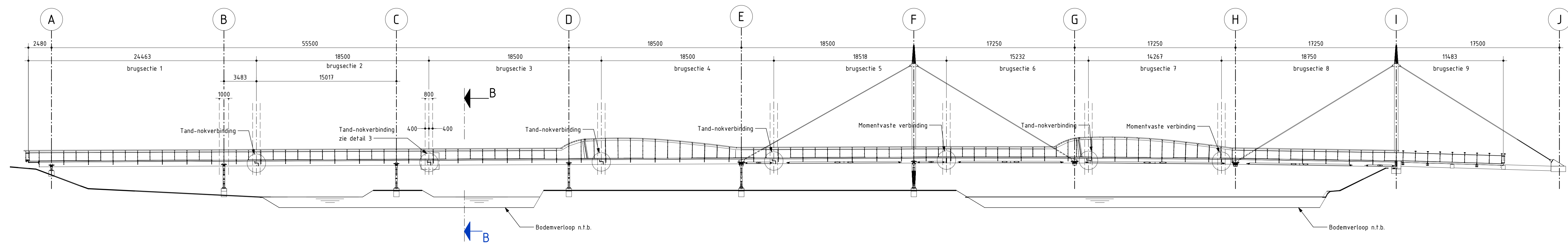
Doorsnede A-A Nieuwe situatie Schaal 1 : 200
