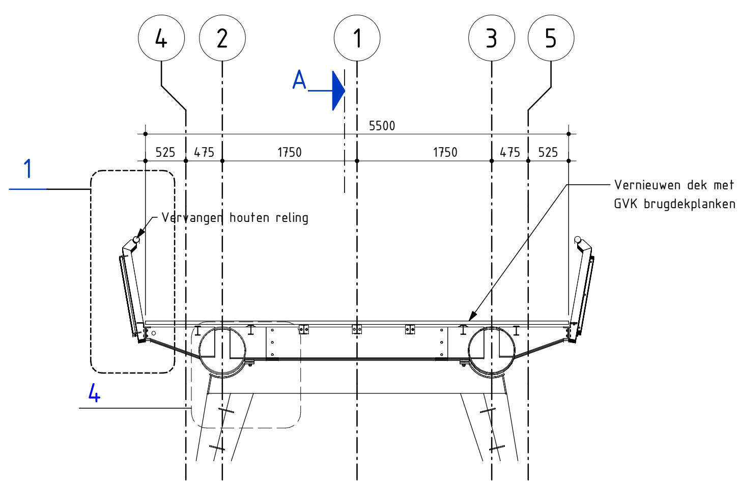
Doorsnede B-B Nieuwe situatie Schaal 1 : 50
