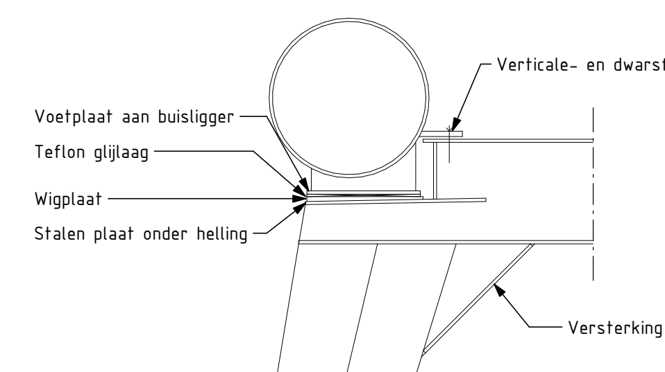
Detail 4 Herziening verbinding portaal-buislijger Schaal 1 : 20
