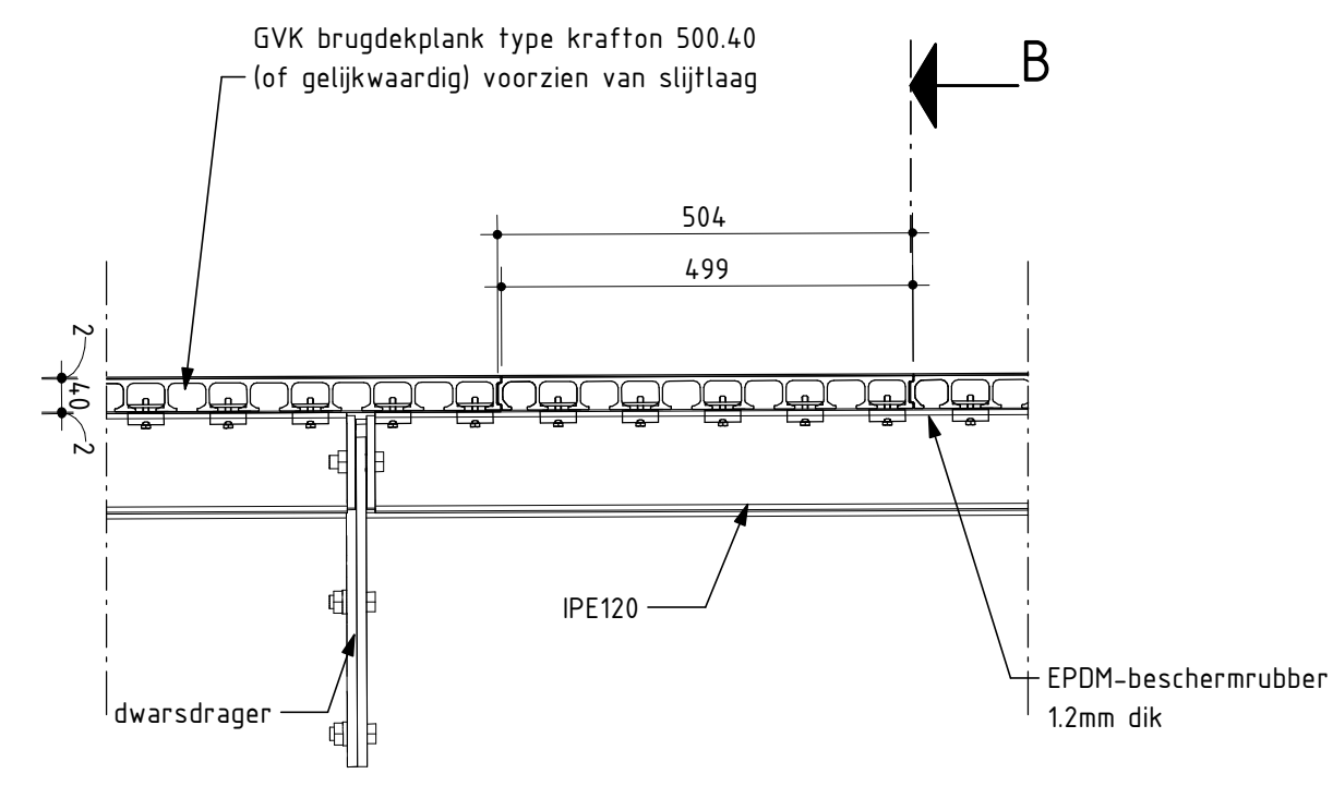
Detail 2 Brugdek (GVK) Schaal 1 : 10
