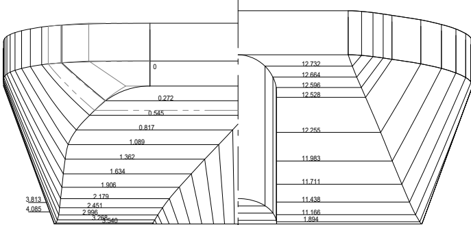
Spantenraam
