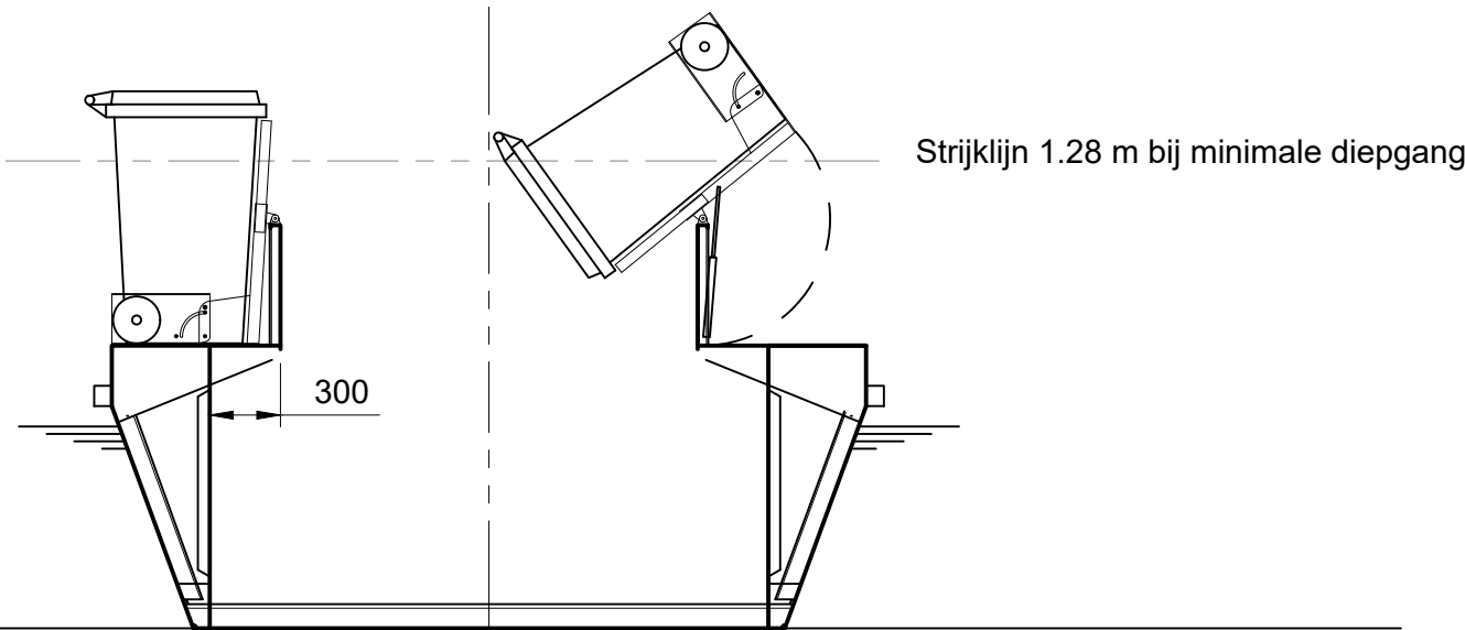
Spant 10 met zij-laders voor 240 L Kliko
