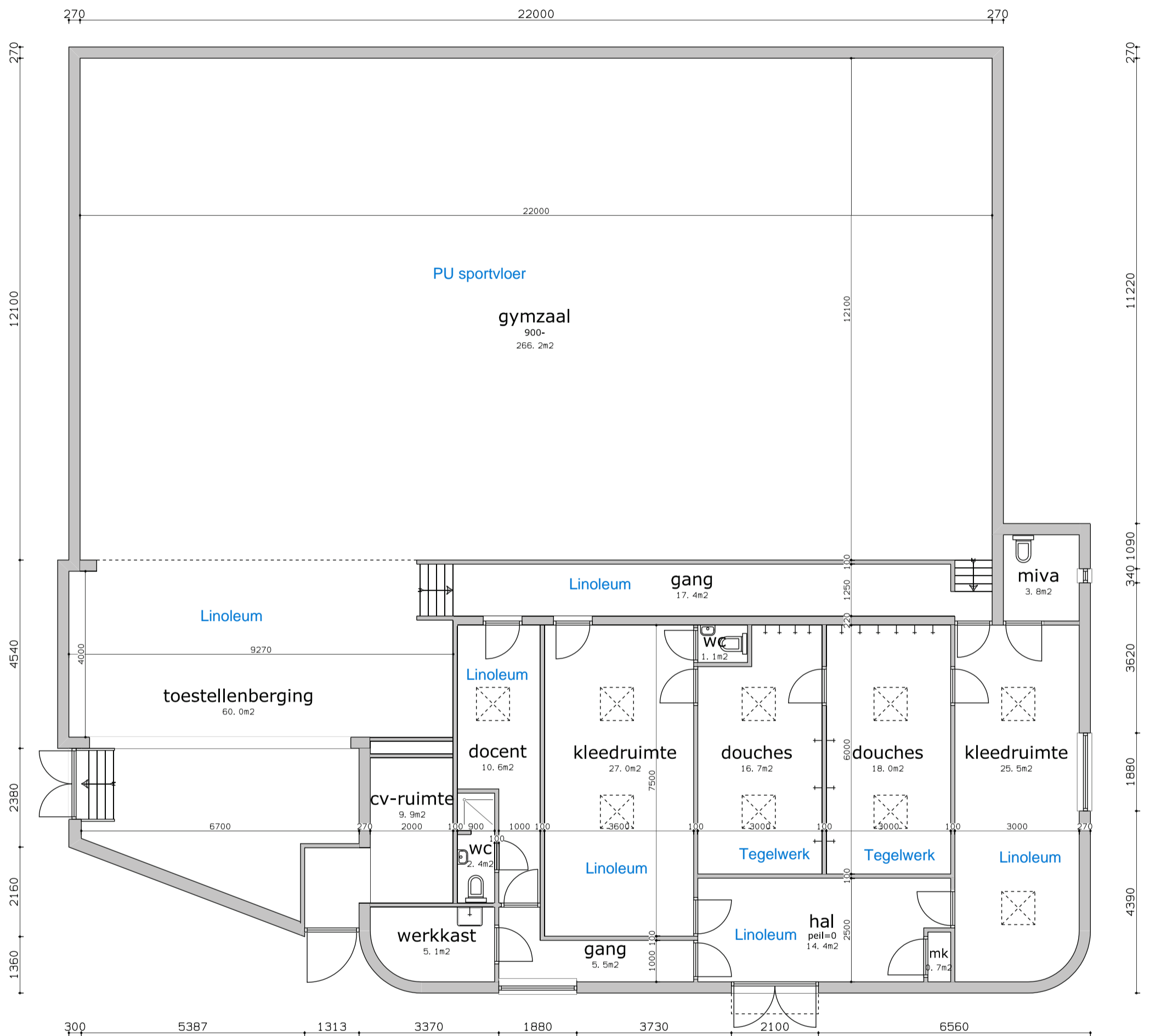
plattegrond begane grond
