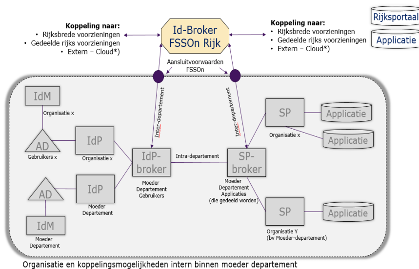
Figuur3: Schematisch overzicht van het federatief stelsel en scope van FSSOn Rijk
