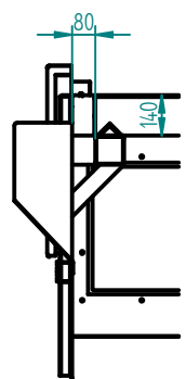
DOORSNEDE B-B
