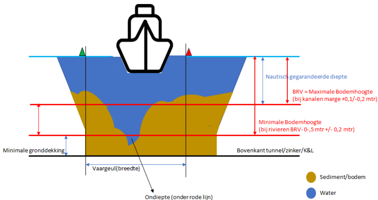
figuur 2.2. Weg te nemen sediment zie hieronder dat een resultaat oplevert dat de vaargeul op BRV-0,5 \pm 0,2 mtr zit
