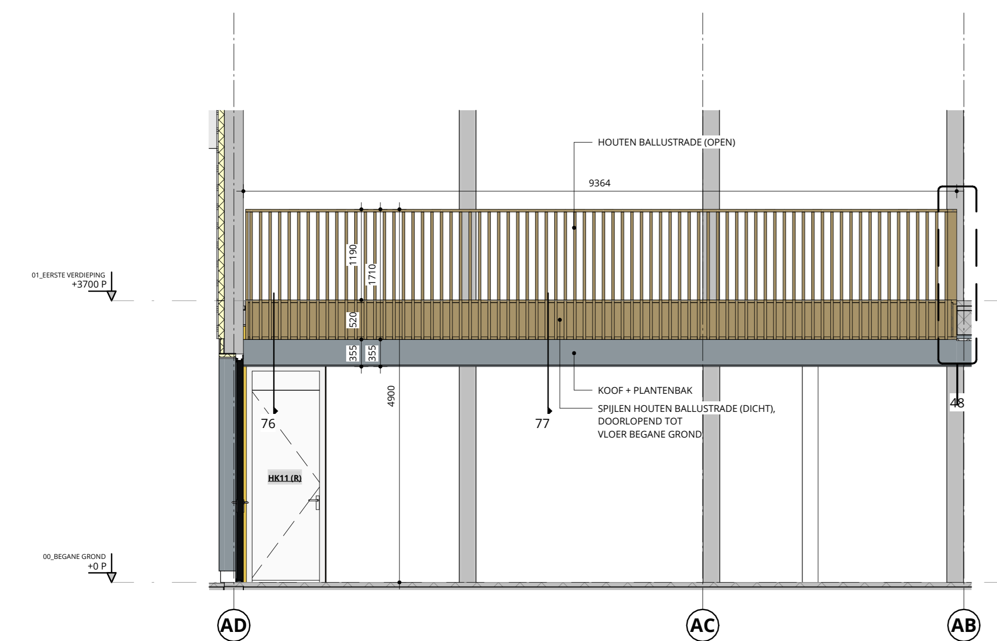
WAZ01 schaal 1:50
