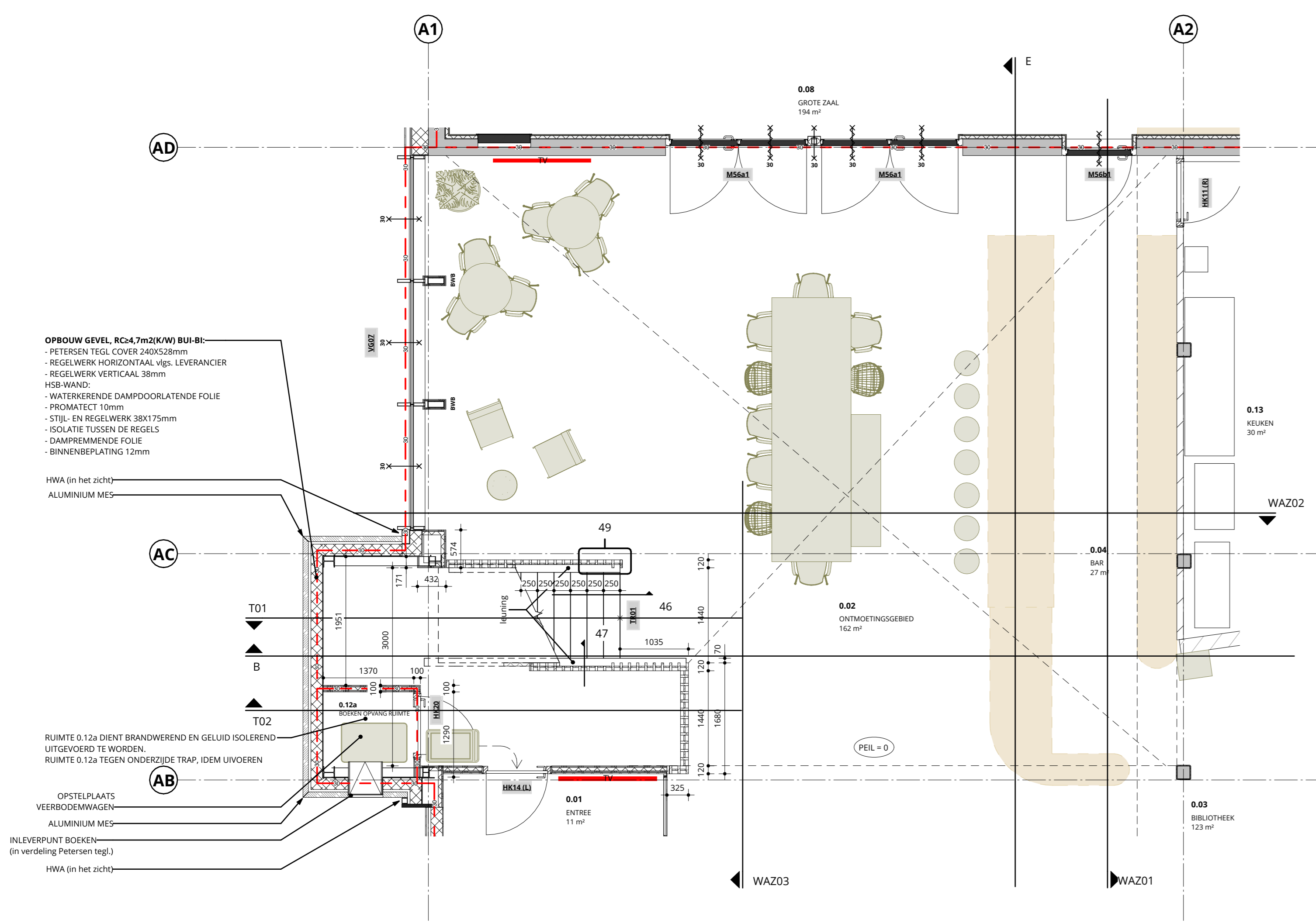
BEGANE GROND schaal 1:50
