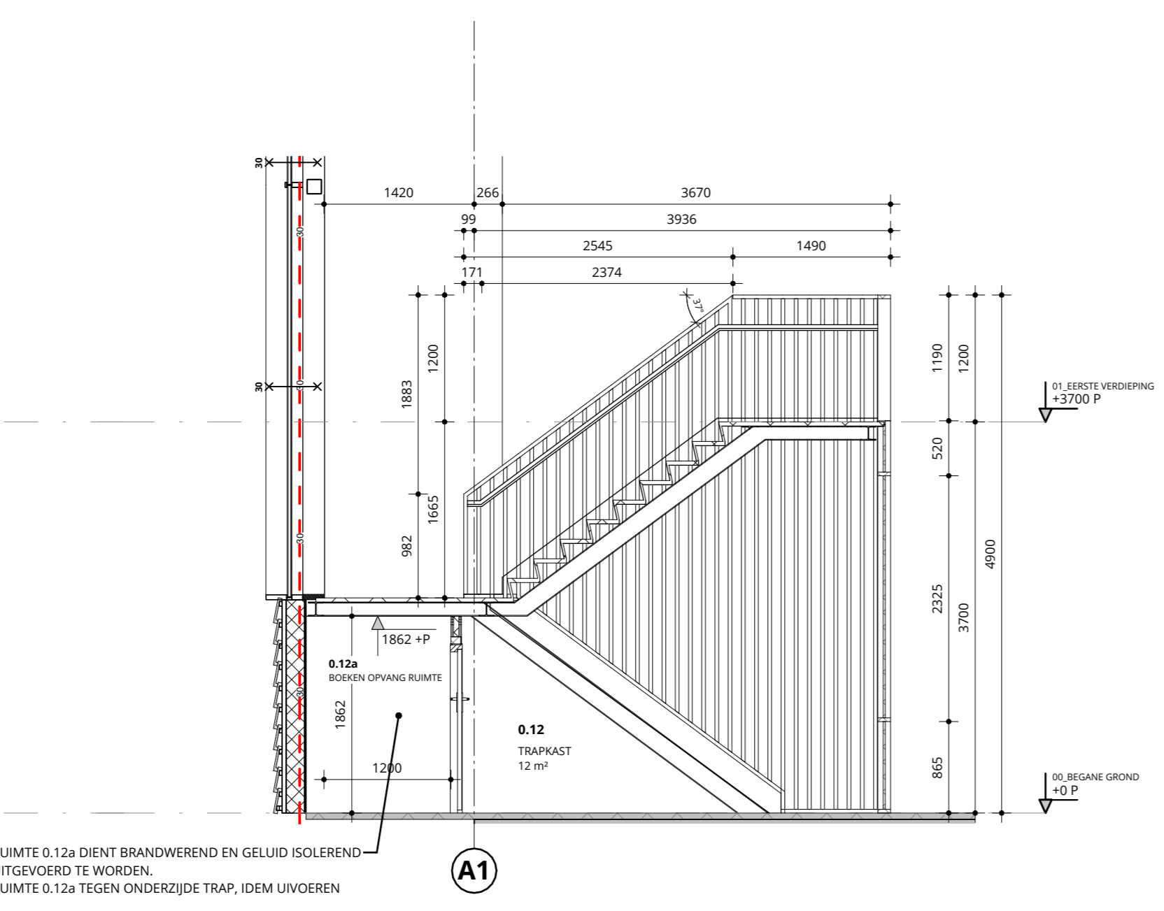
T02 schaal 1:50
