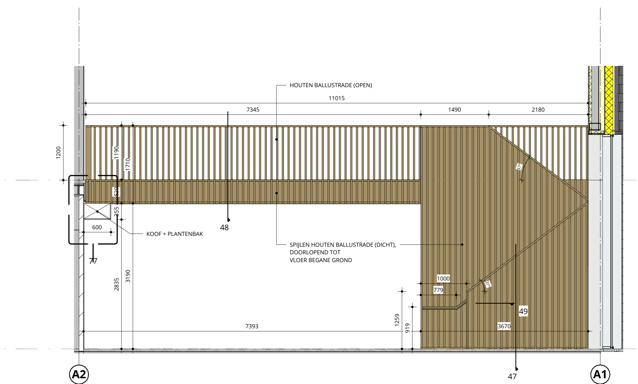
WAZ02 schaal 1:50
