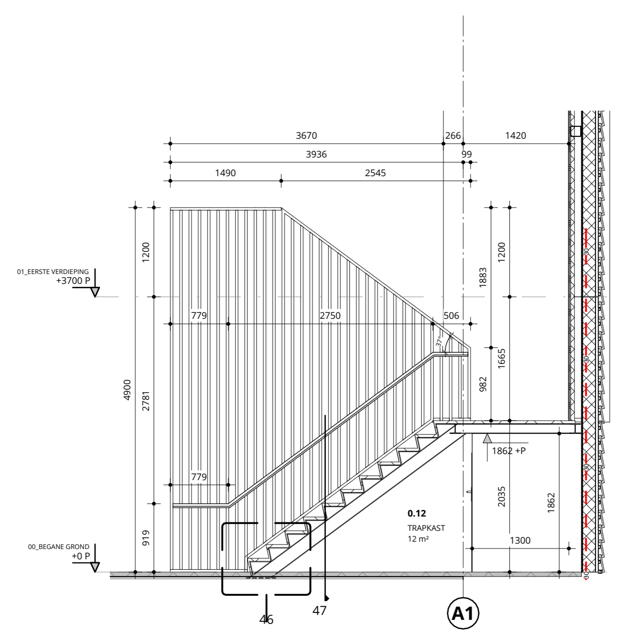
T01 schaal 1:50
