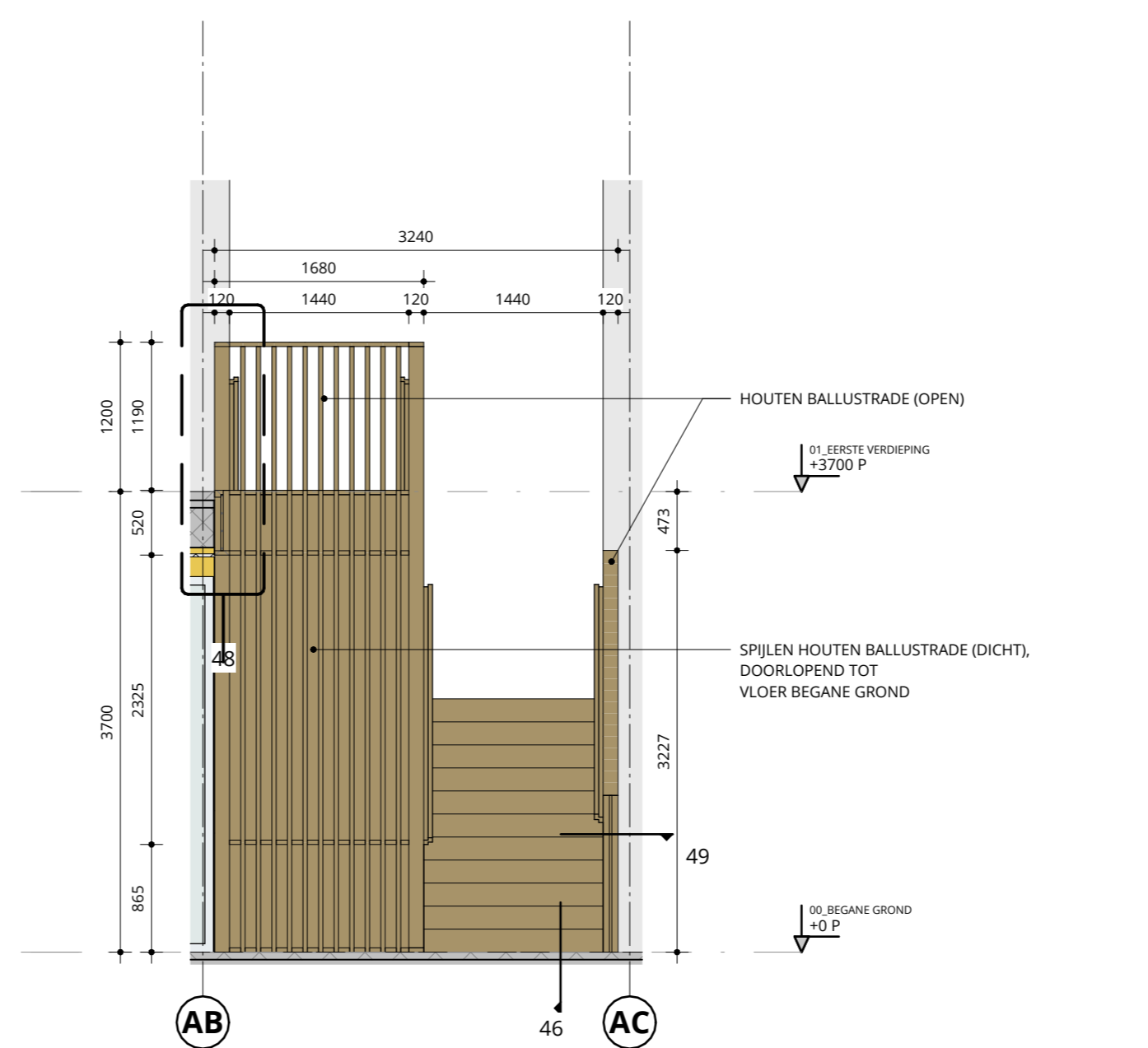
WAZ03 schaal 1:50
