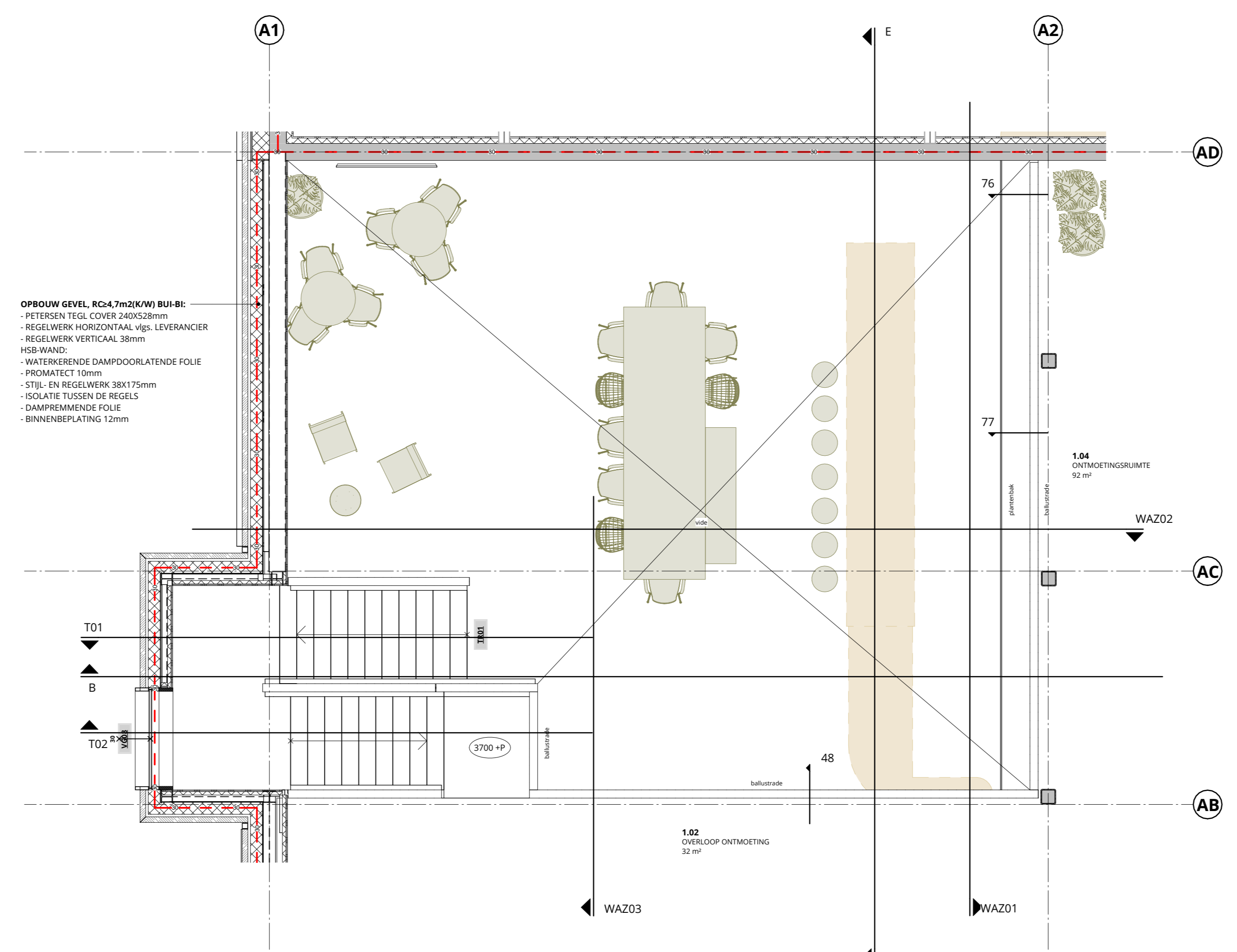
EERSTE VERDIEPING schaal 1:50
