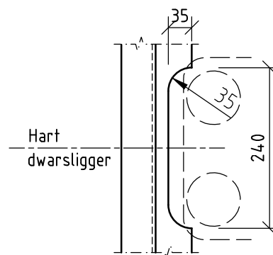
Uitsparing onderflens
