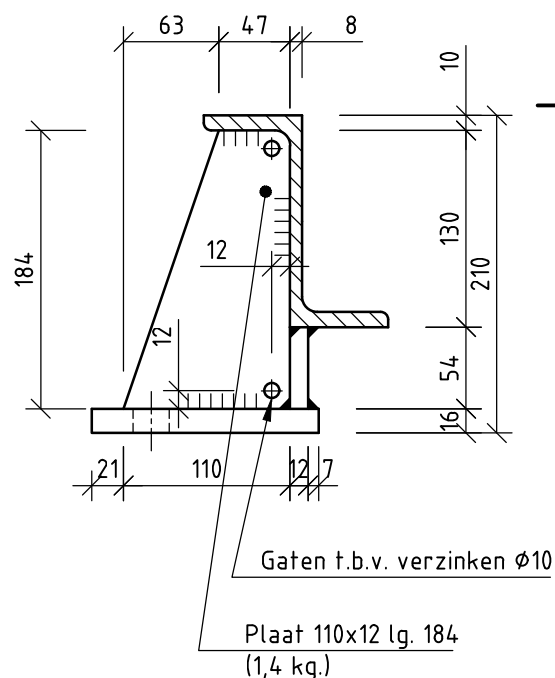
Uitsparing onderflens
