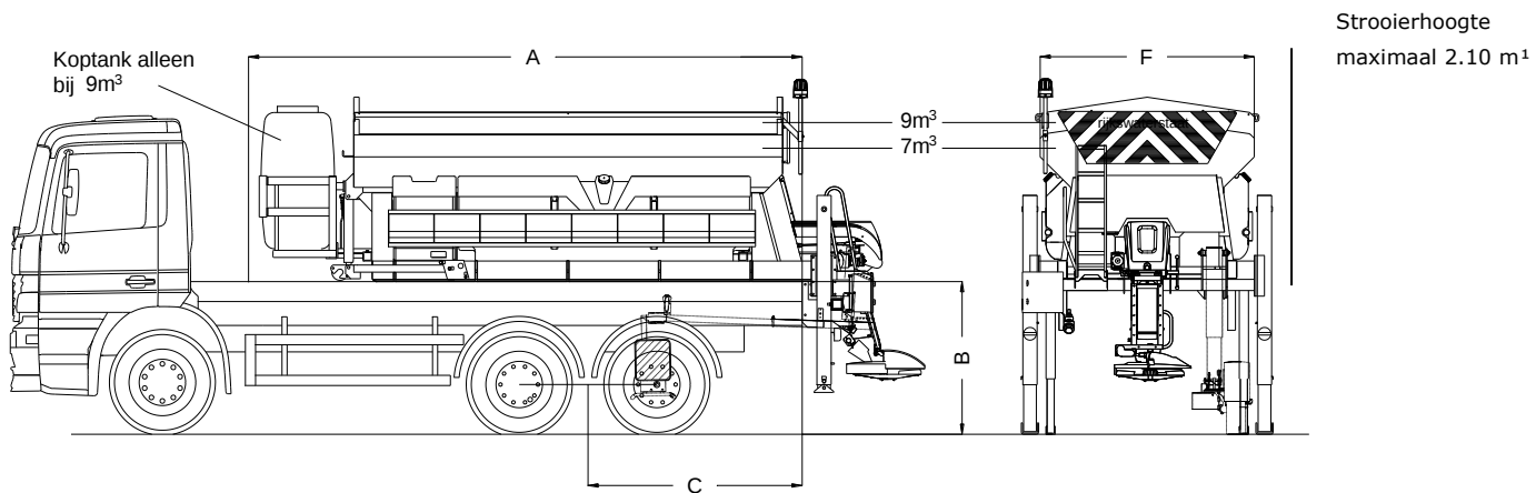
Figuur 1 : Afmetingen vrachtauto's en strooiers
