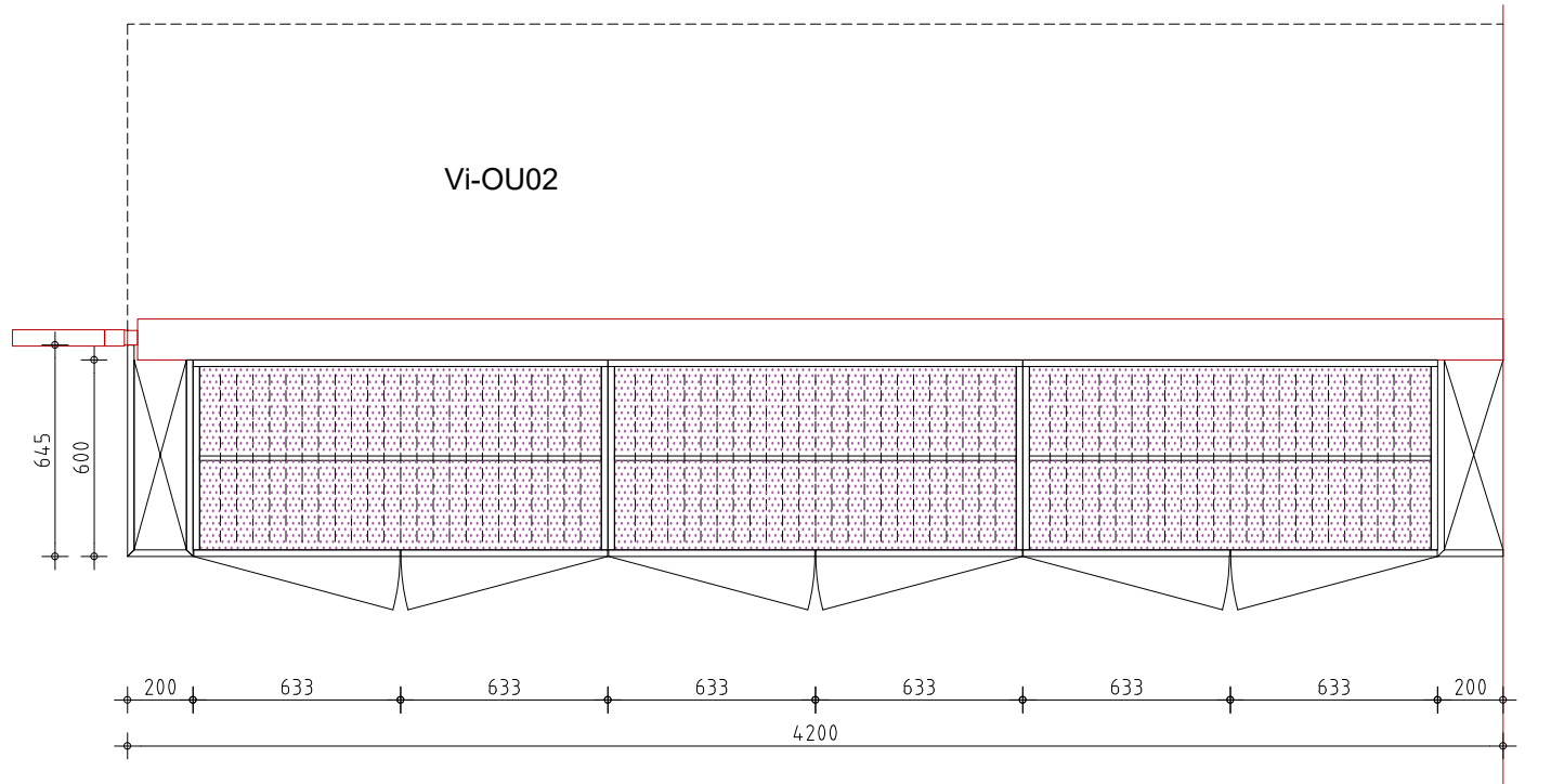
plattegrond
