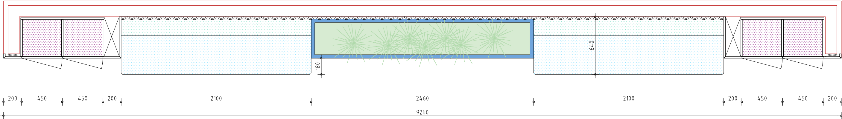
bovenaanzicht
