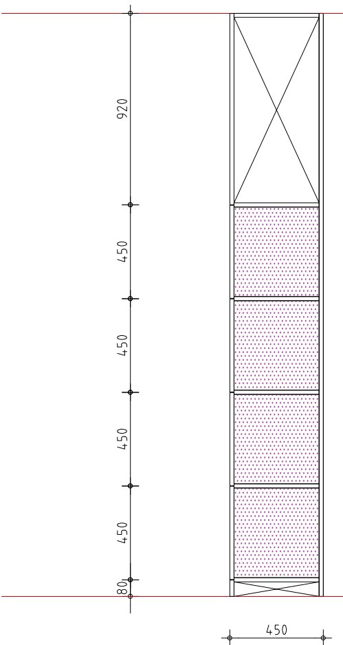
dwarsdoorsnede
