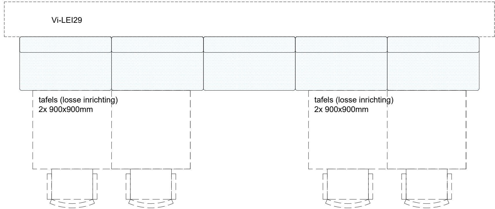
bovenaanzicht
