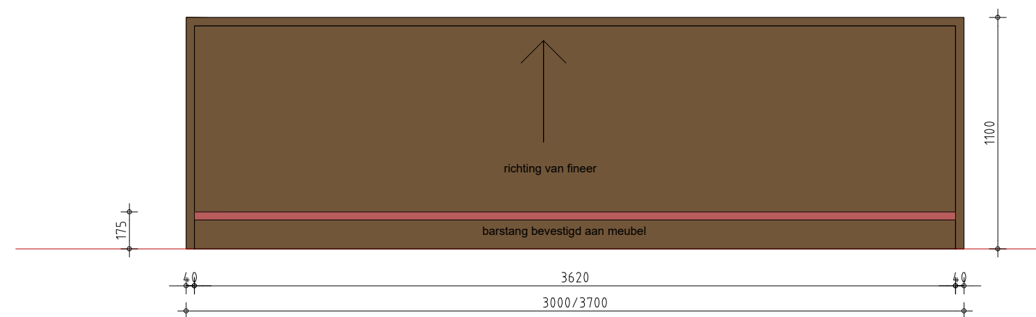
vooraanzicht
