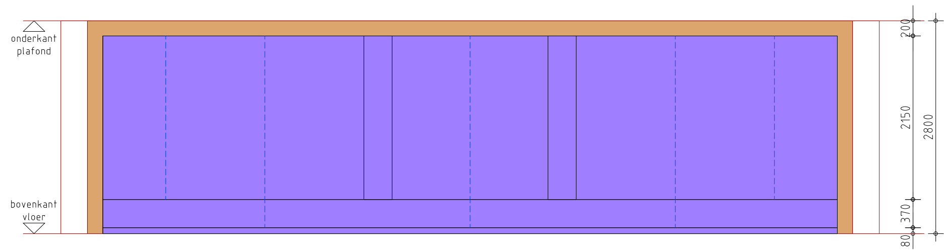
vooraanzicht
