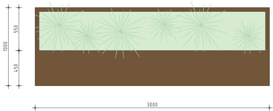
bovenaanzicht
