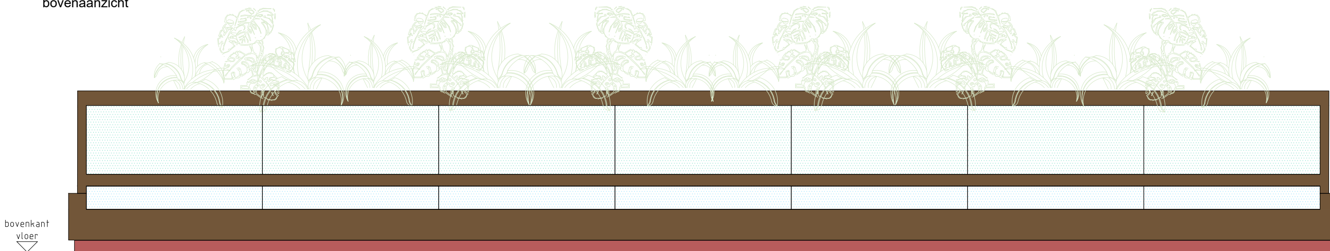
bovenaanzicht
