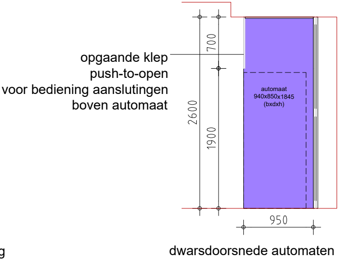
dwarsdoorsnede afvalinzameling
