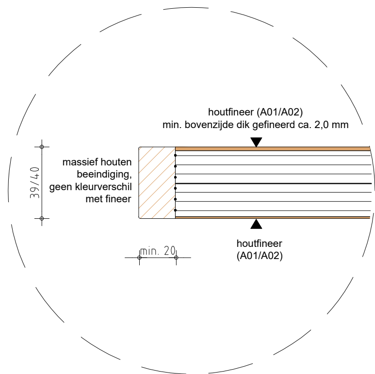
1.0 principe voor tafelbladen, staanders en planken bekleed met houtfineer
