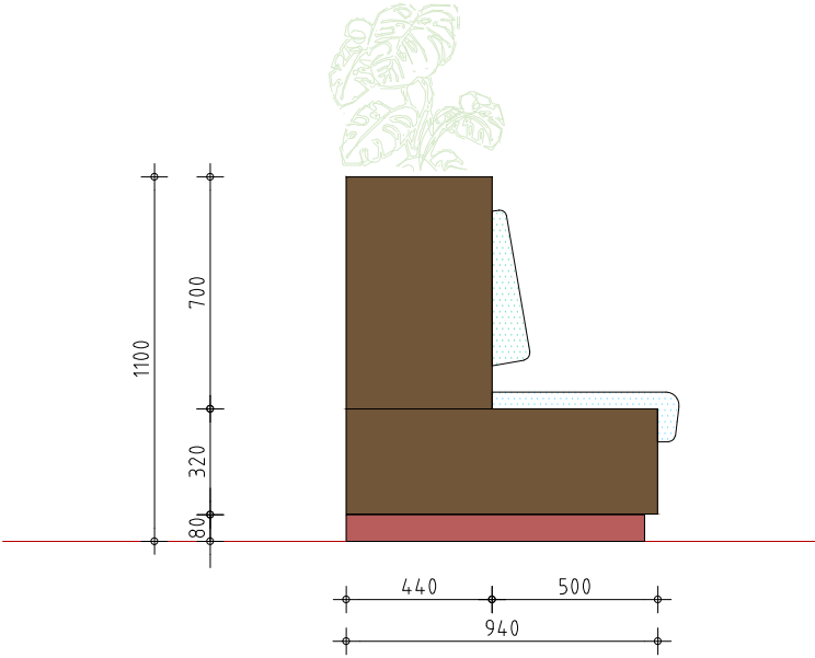
zij-aanzicht
