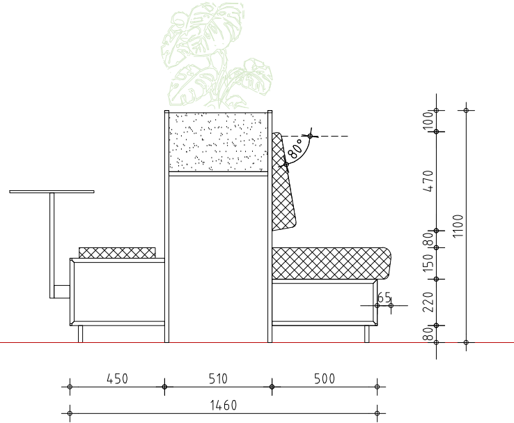
doorsnede 2
