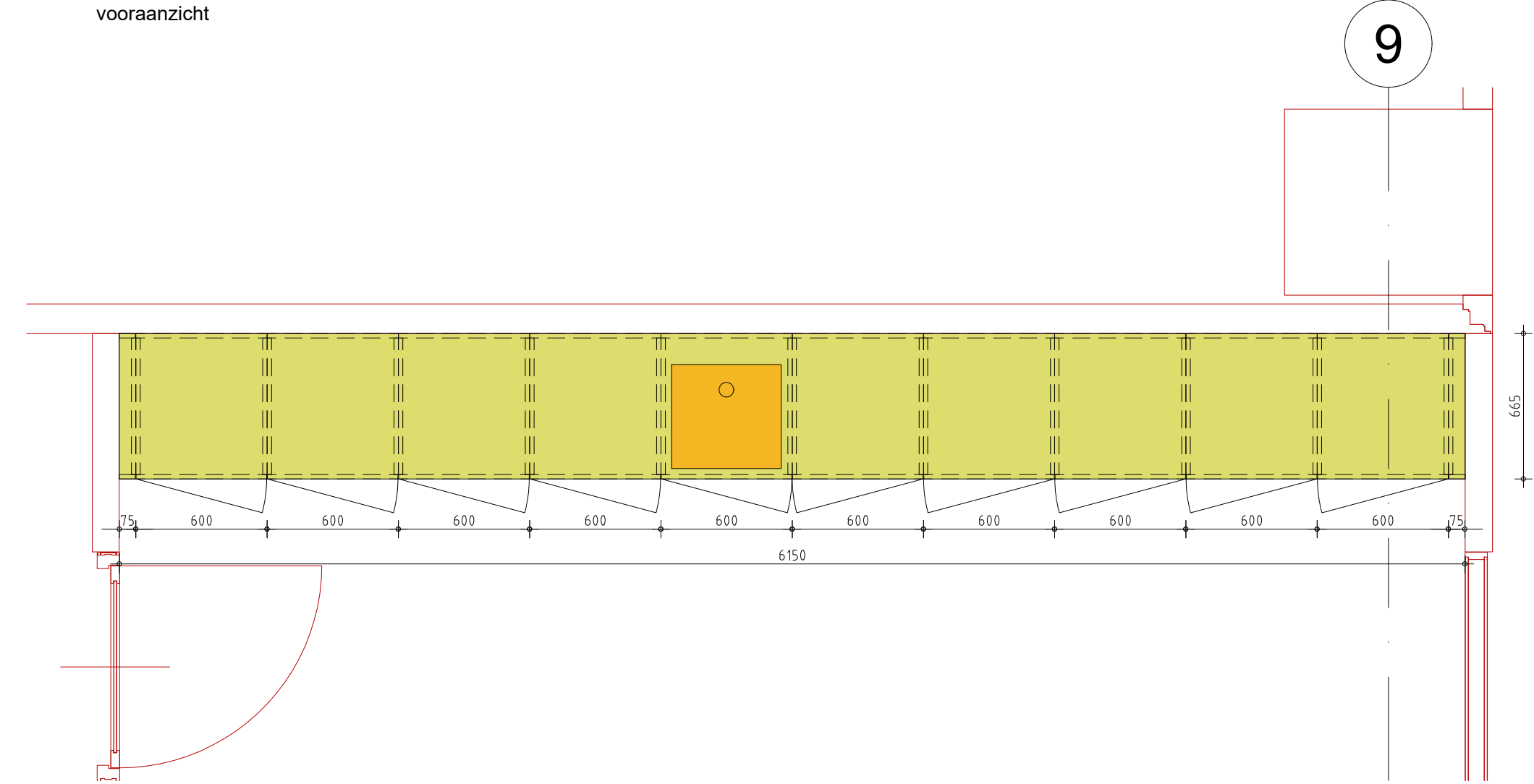
bovenaanzicht
