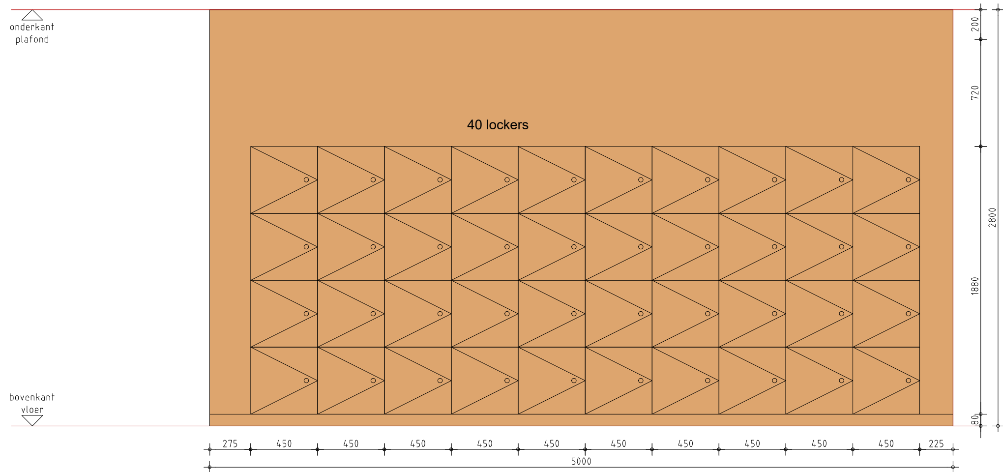
vooraanzicht
