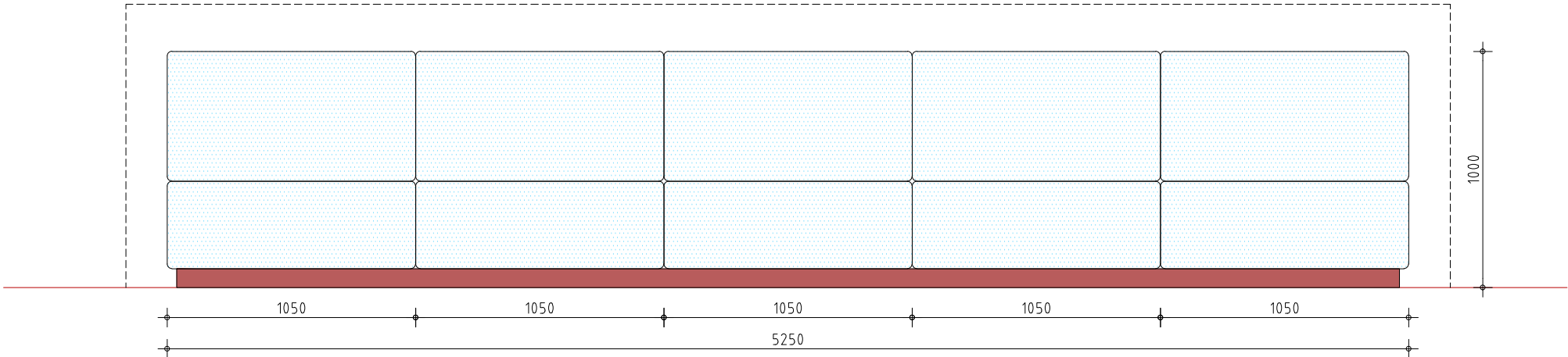
vooraanzicht
