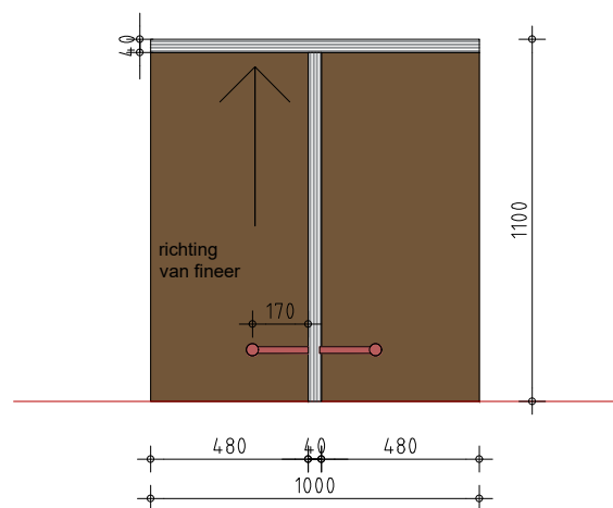
dwarsdoorsnede
