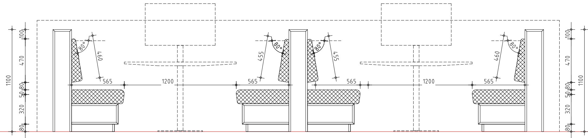
langsdoorsnede
