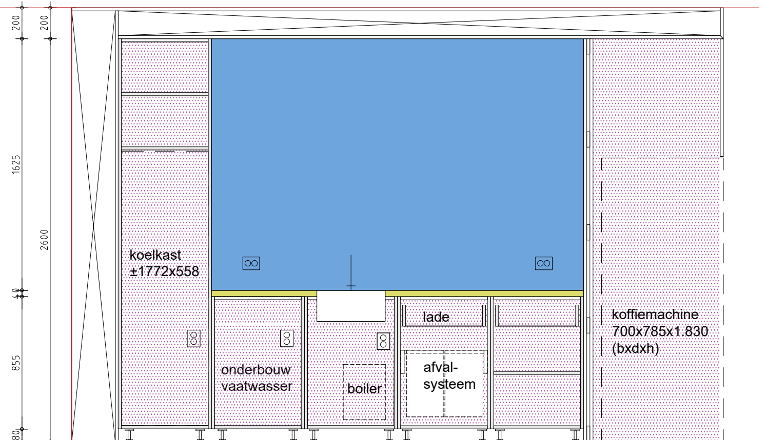
langsdoorsnede
