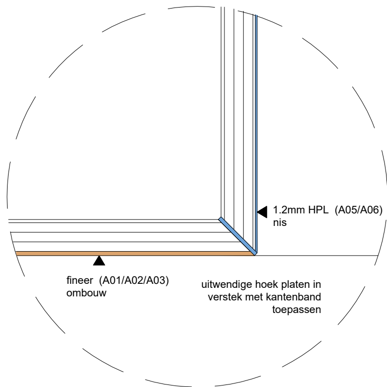
2.3 aansluiting HPL nis in fineer ombouw
