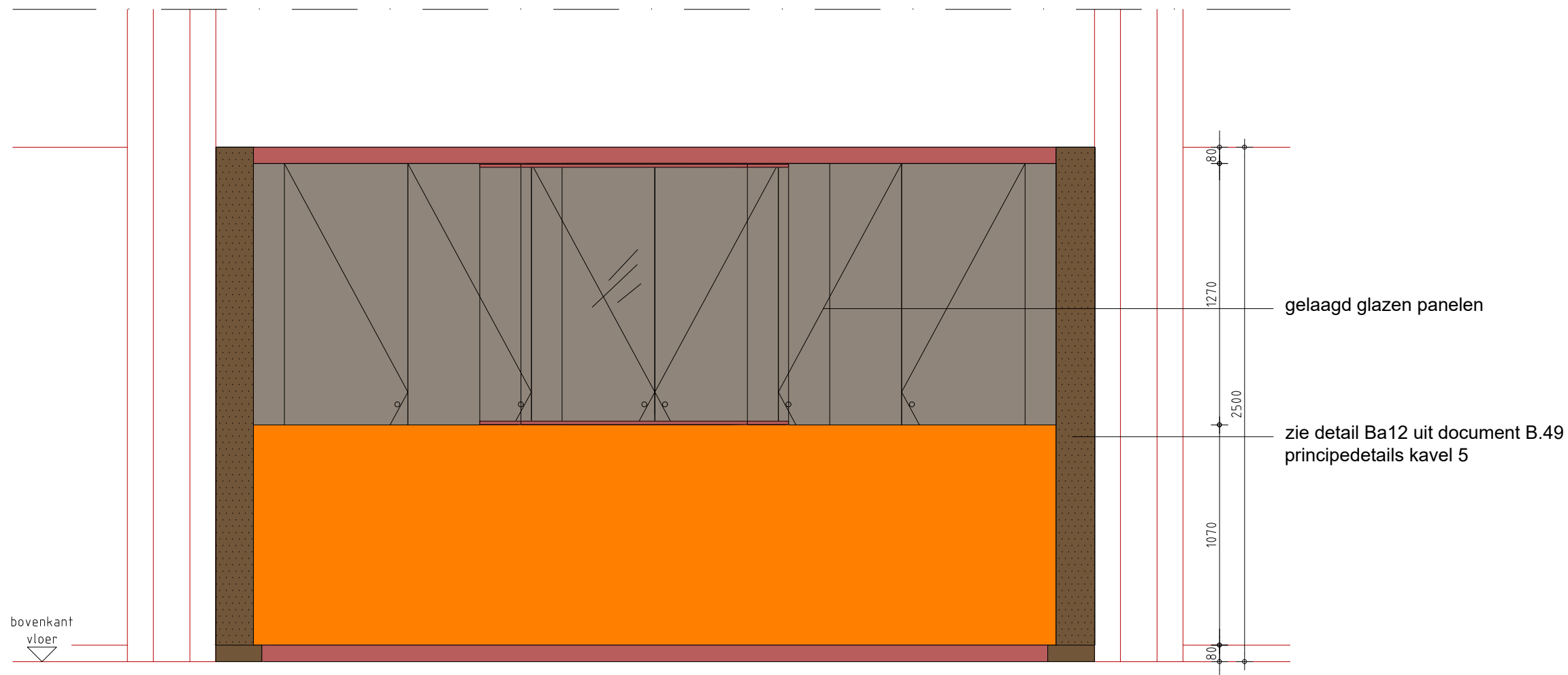
vooraanzicht
