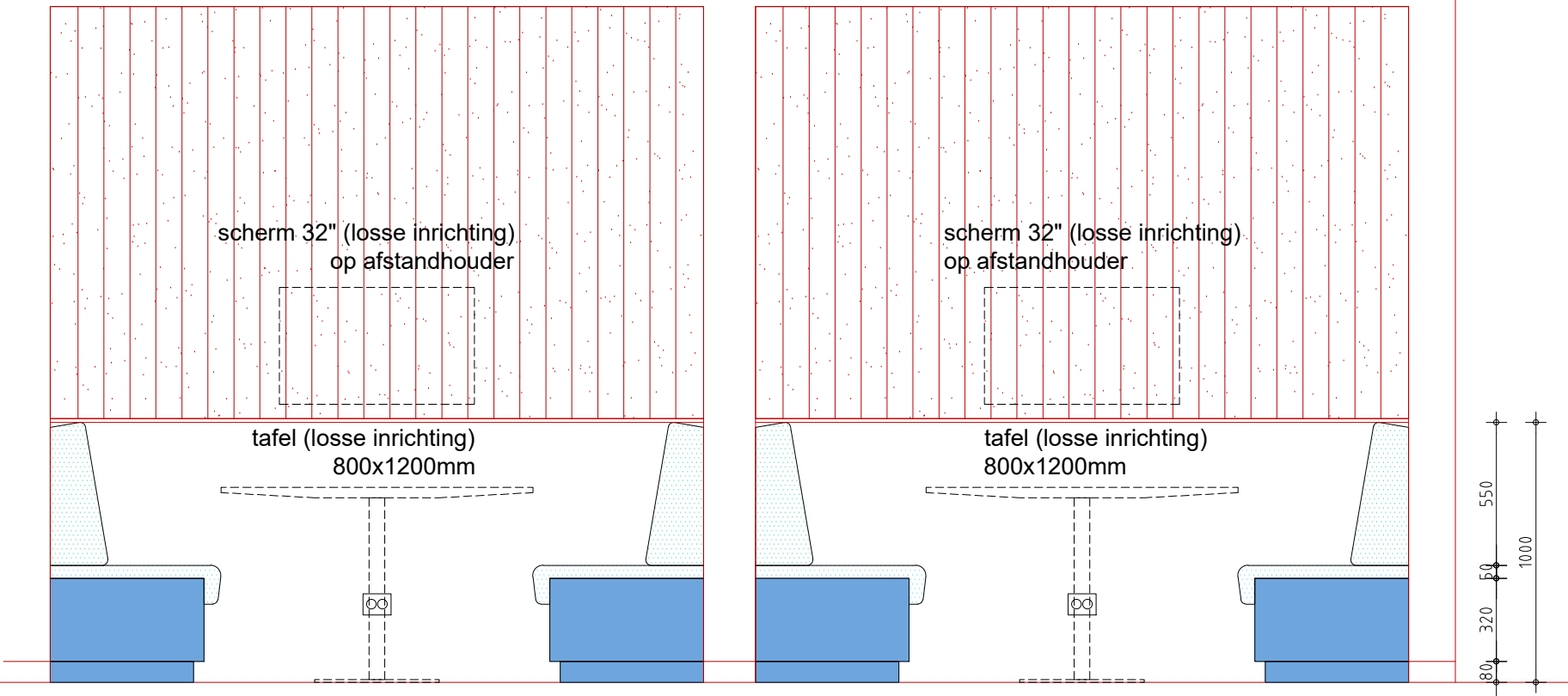
vooraanzicht
