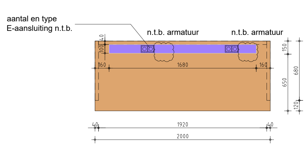
bovenaanzicht
