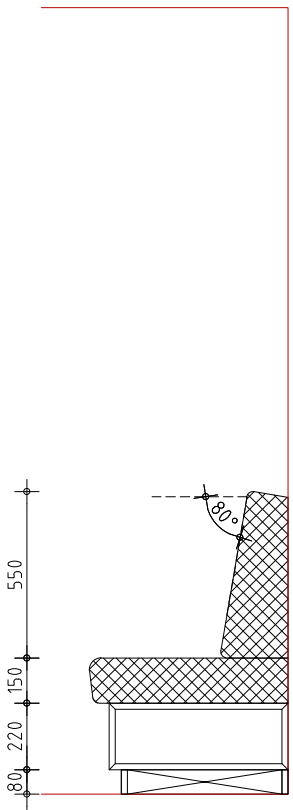
dwarsdoorsnede
