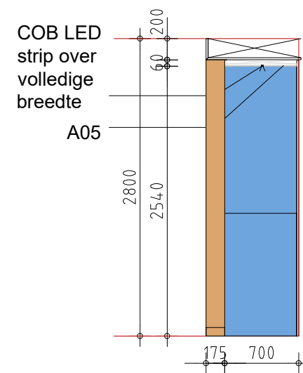
dwarsdoorsnede printernis
