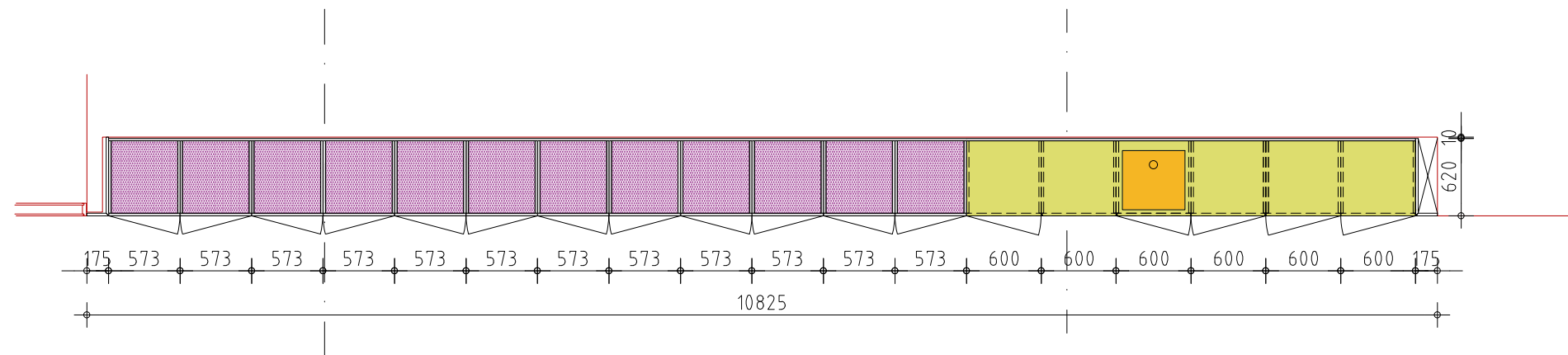
vooraanzicht
