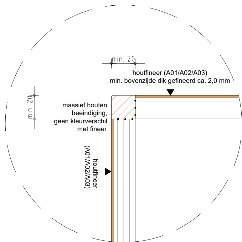
1.1 Optie 1 uitwendige hoeken in houtfineer
