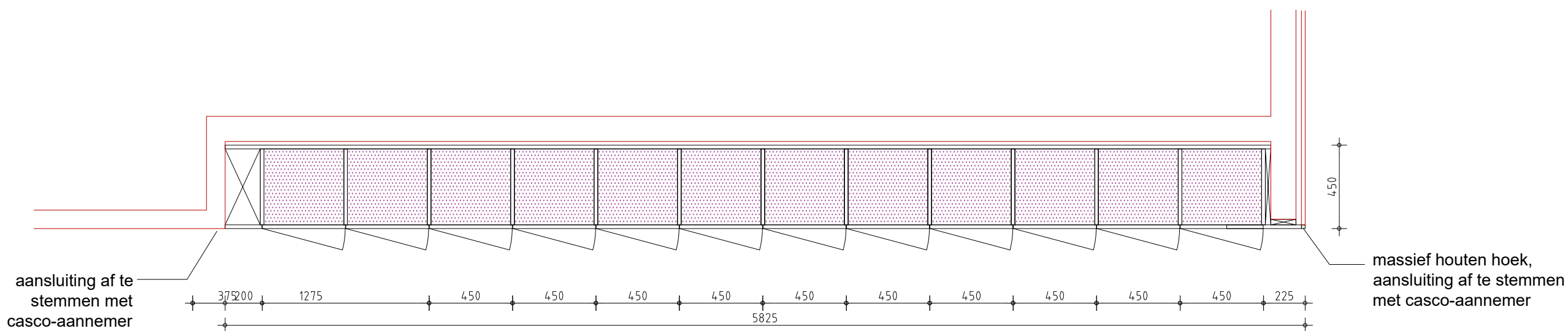
plattegrond
