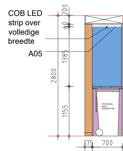
dwarsdoorsnede papierbak
