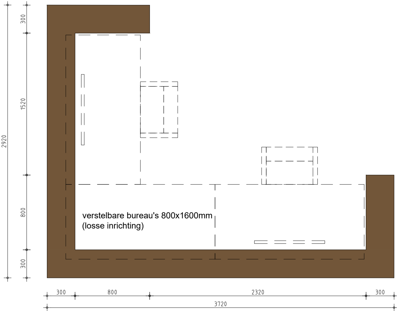
bovenaanzicht
