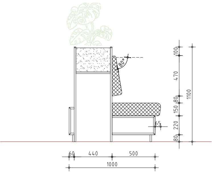
doorsnede 2
