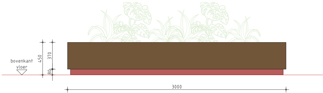
vooraanzicht
