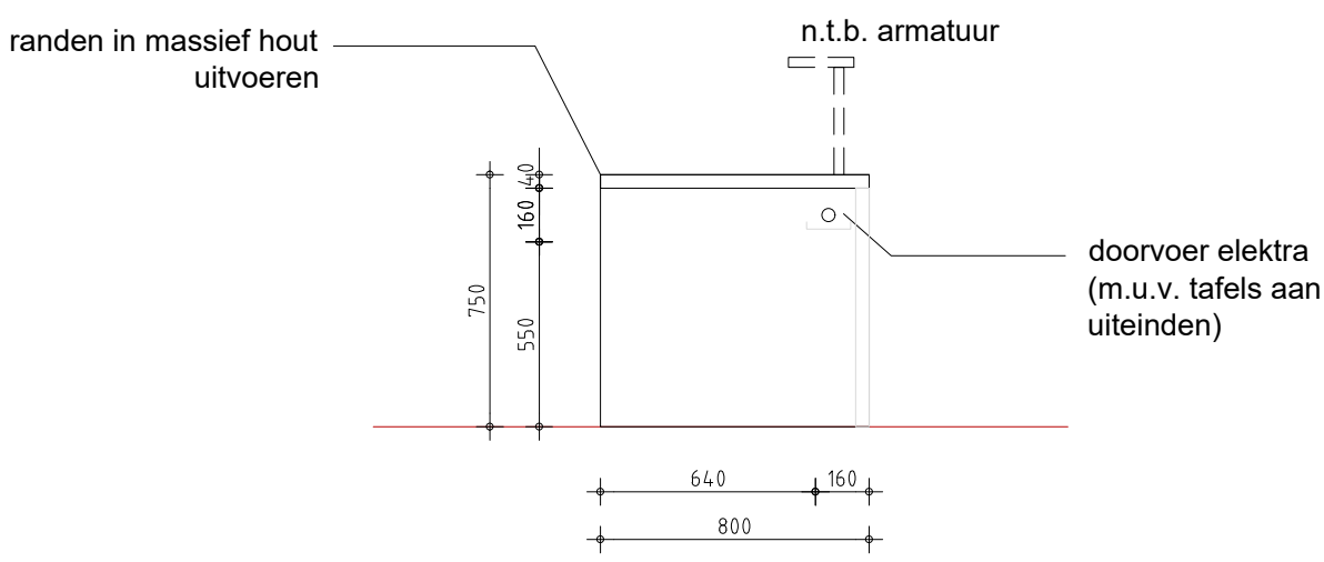
dwarsdoorsnede
