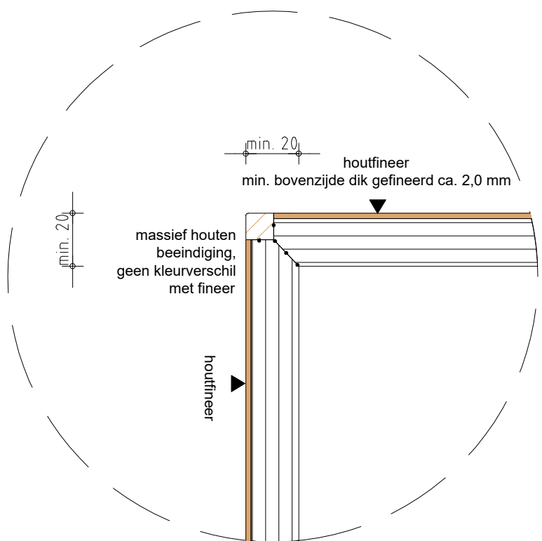
1.2 Optie 2 uitwendige hoeken in houtfineer
