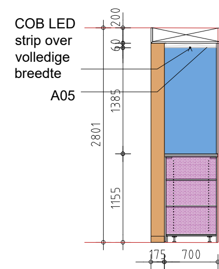
dwarsdoorsnede kast
