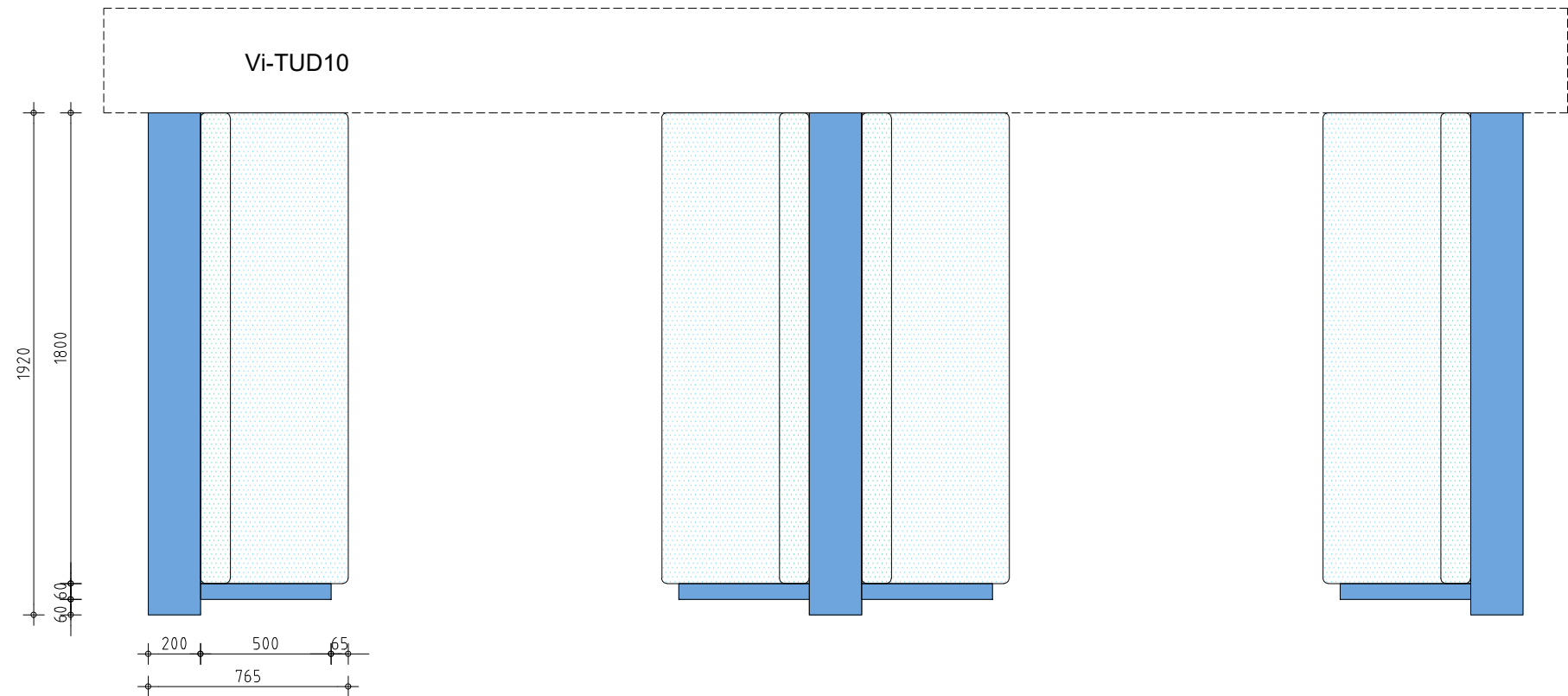
bovenaanzicht
