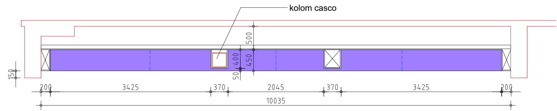
plattegrond
