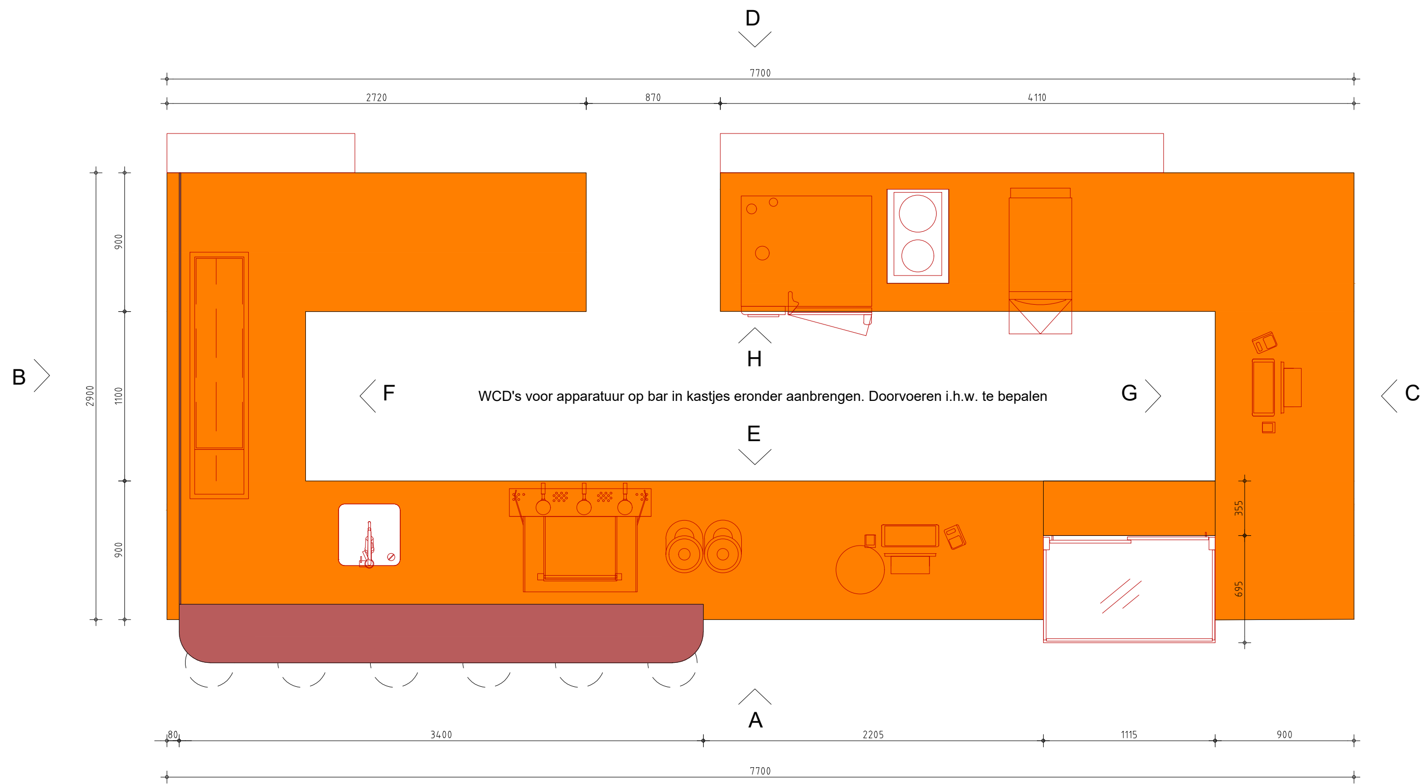
bovenaanzicht
