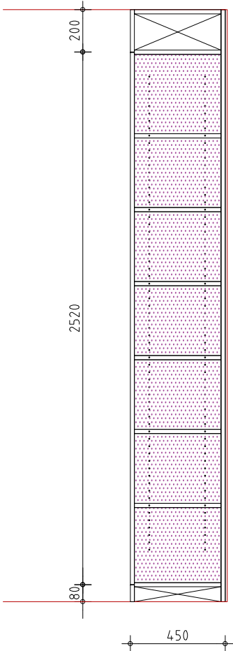
dwarsdoorsnede
