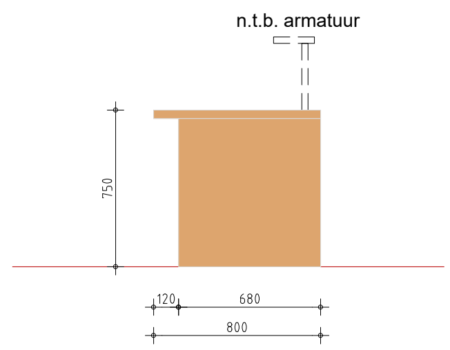
zij-aanzicht
