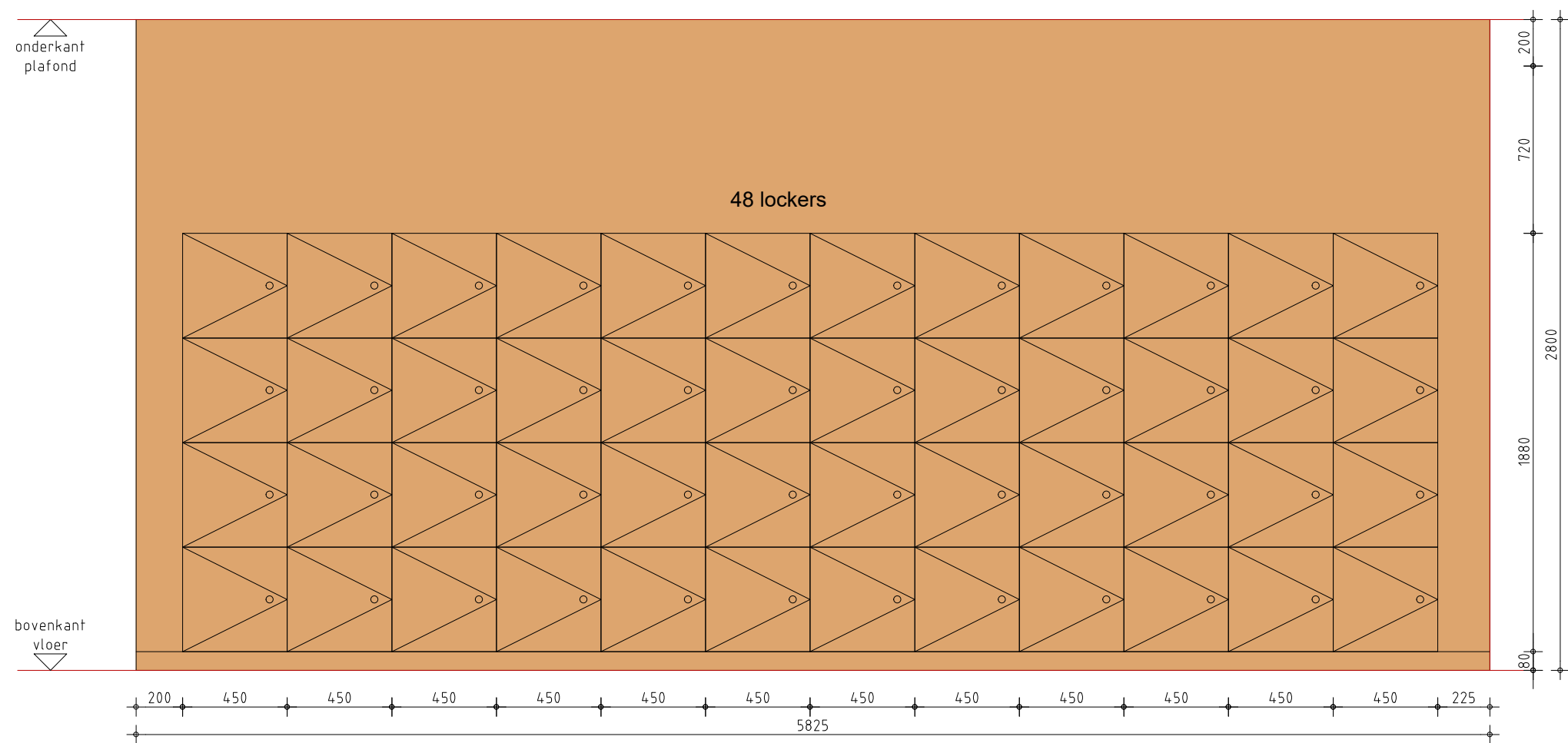
vooraanzicht
