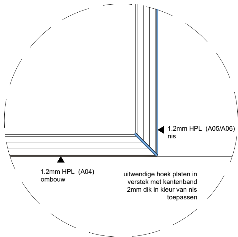
2.2 aansluiting HPL nis in HPL ombouw
