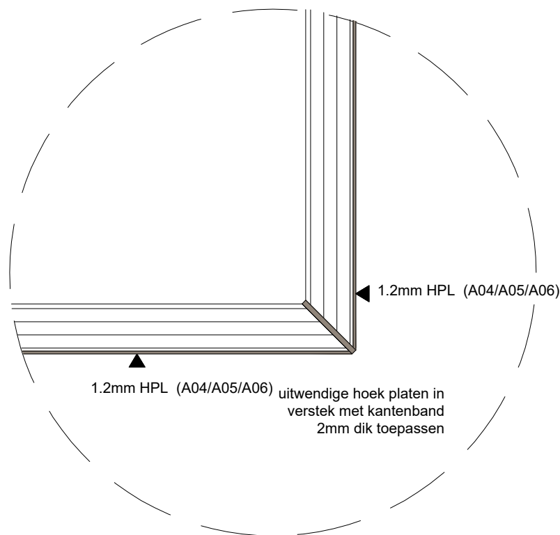
2.0 uitwendige hoeken HPL
