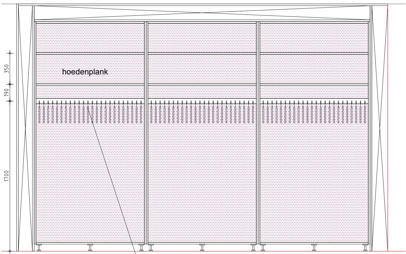
langsdoorsnede
