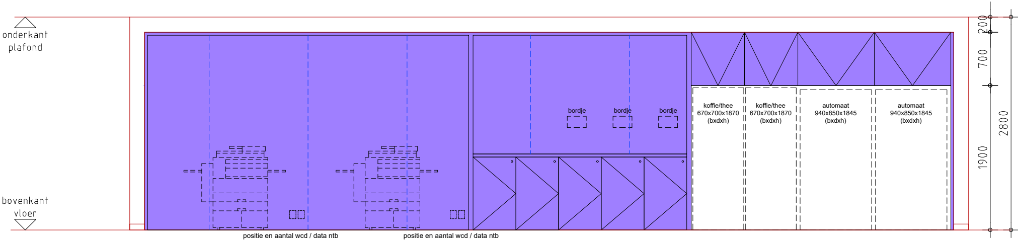
vooraanzicht
