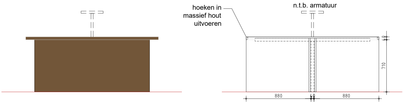
zij-aanzicht
