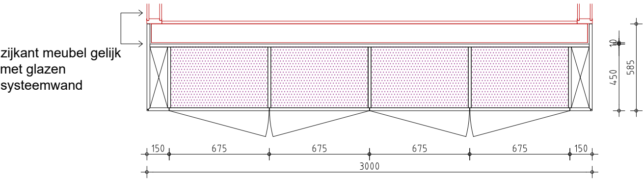
plattegrond
