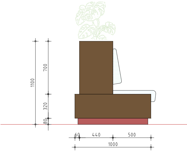
zij-aanzicht
