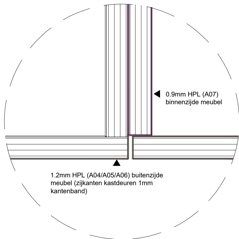
2.1 aansluiting HPL kastdeur HPL ombouw
