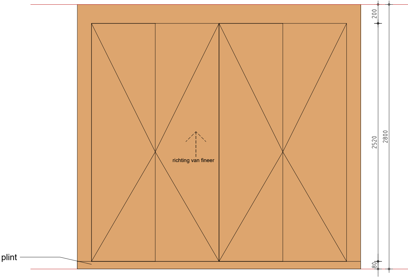
vooraanzicht
