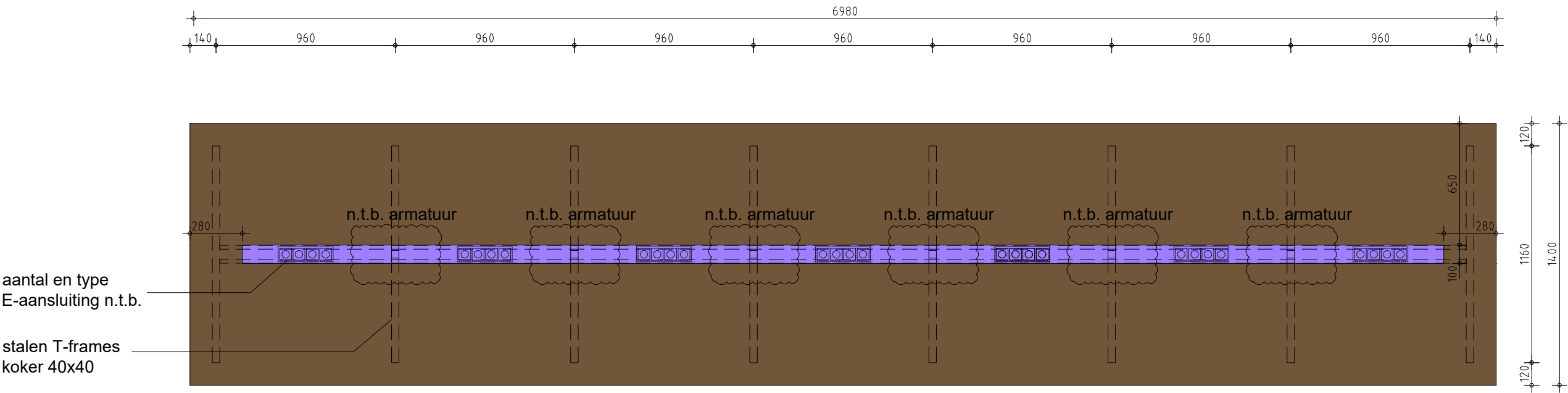
bovenaanzicht
