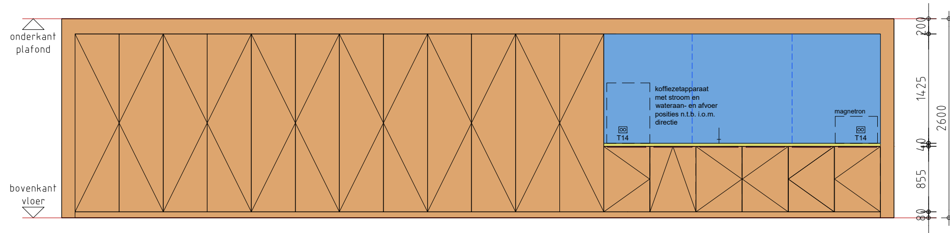
vooraanzicht
