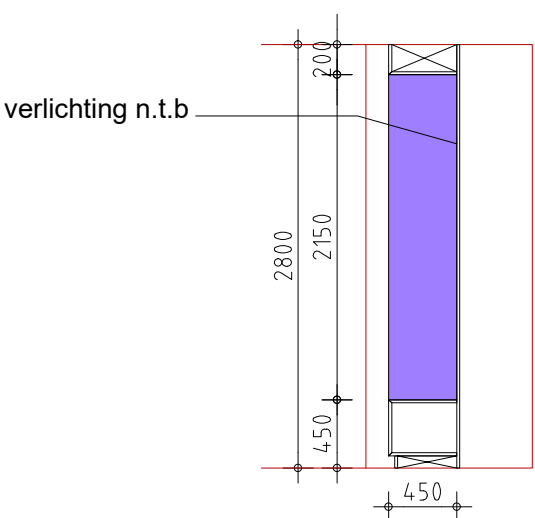
dwarsdoorsnede
