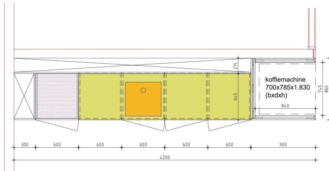
vooraanzicht
