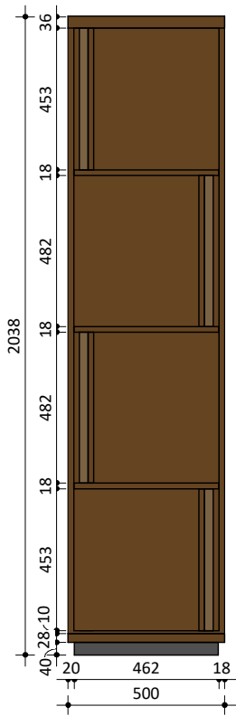
Doorsnede
