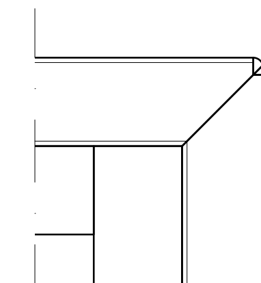
detail 'bilverstek'
