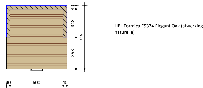
Dwarsdoorsnede
