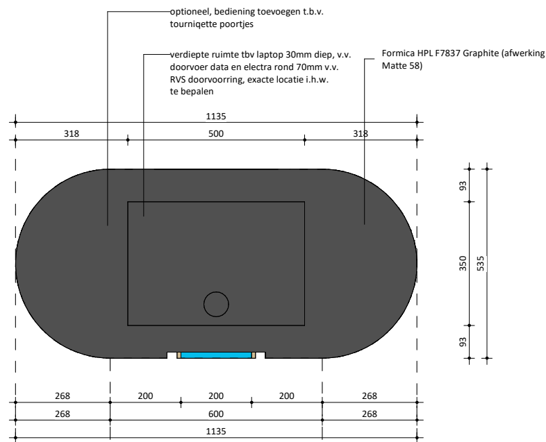
Bovenaanzicht
