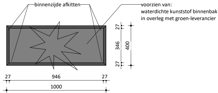
Bovenaanzicht
