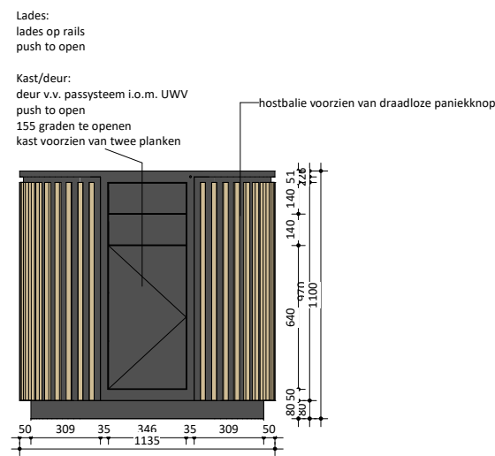
Achteraanzicht
