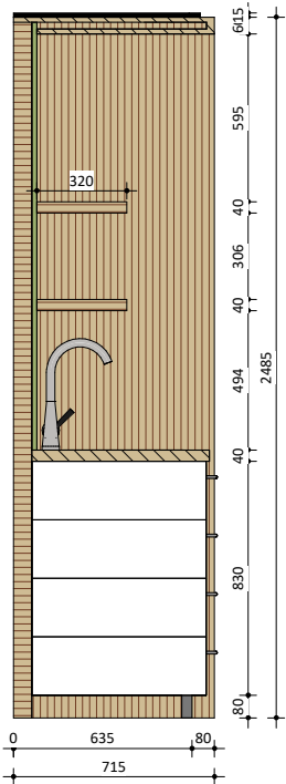
Doorsnede
