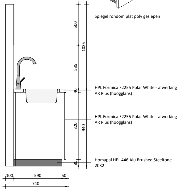
Doorsnede
