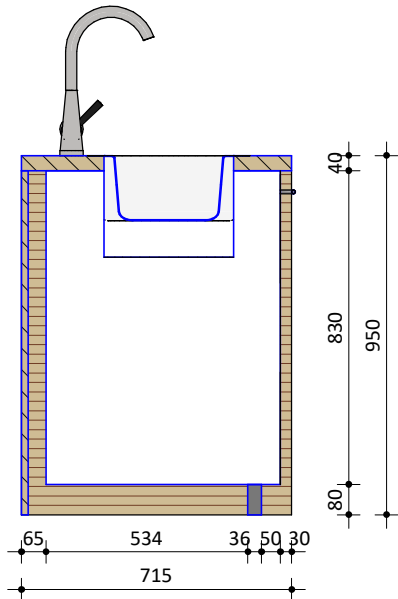
Doorsnede
