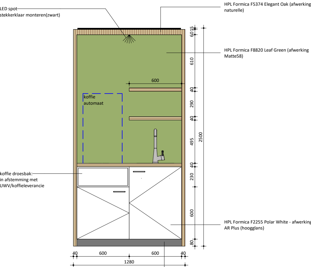
Vooraanzicht
