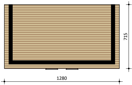
Bovenaanzicht
