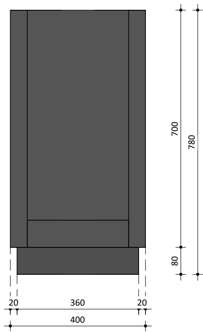
Doorsnede A
