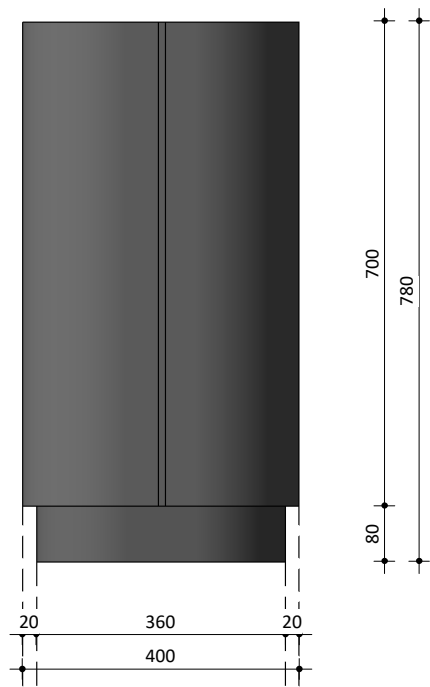
Rechter zijaanzicht
