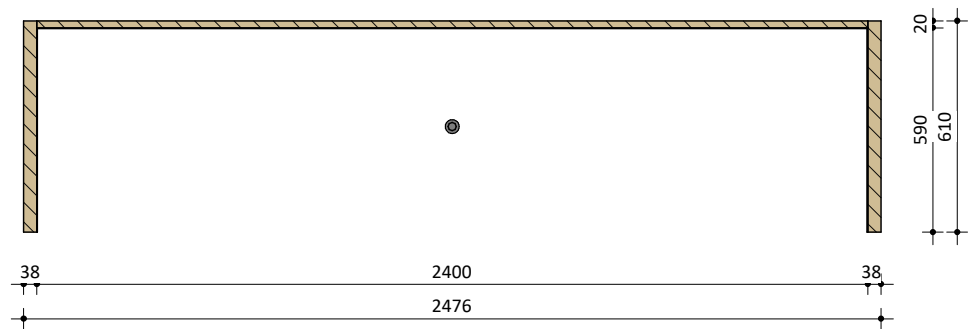
Plattegrond
