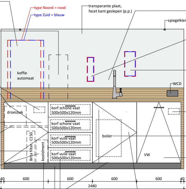
Vooraanzicht
