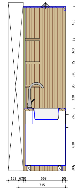
Doorsnede
