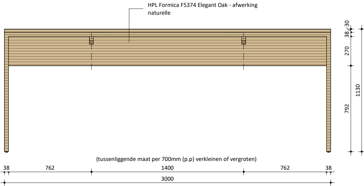
Vooraanzicht
