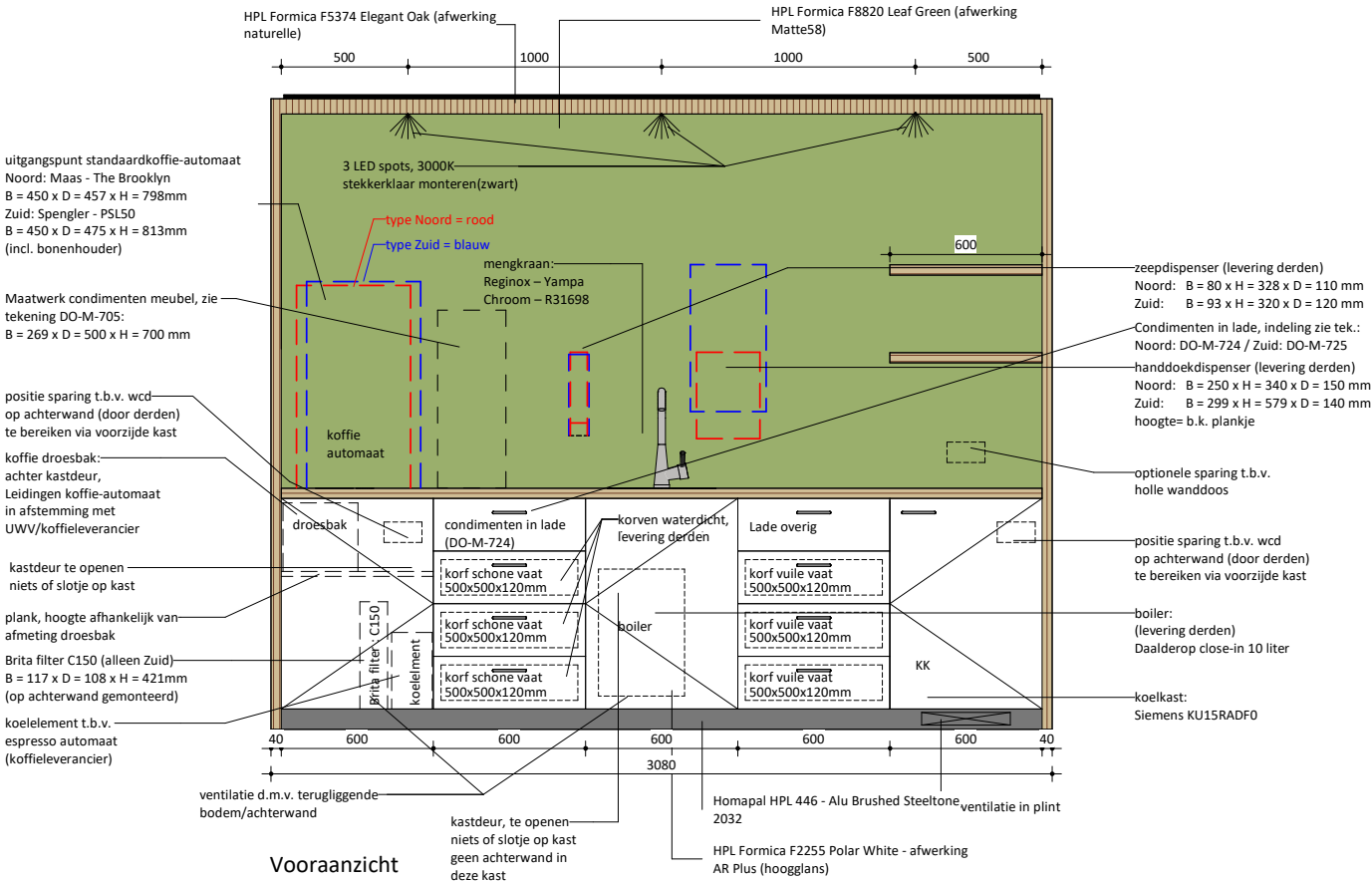
Vooraanzicht
