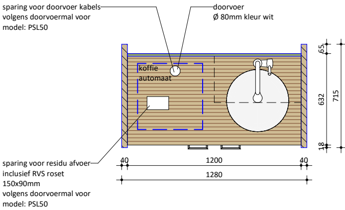
Plattegrond
