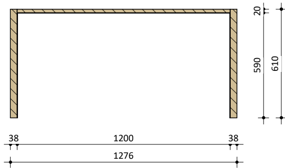
Plattegrond
