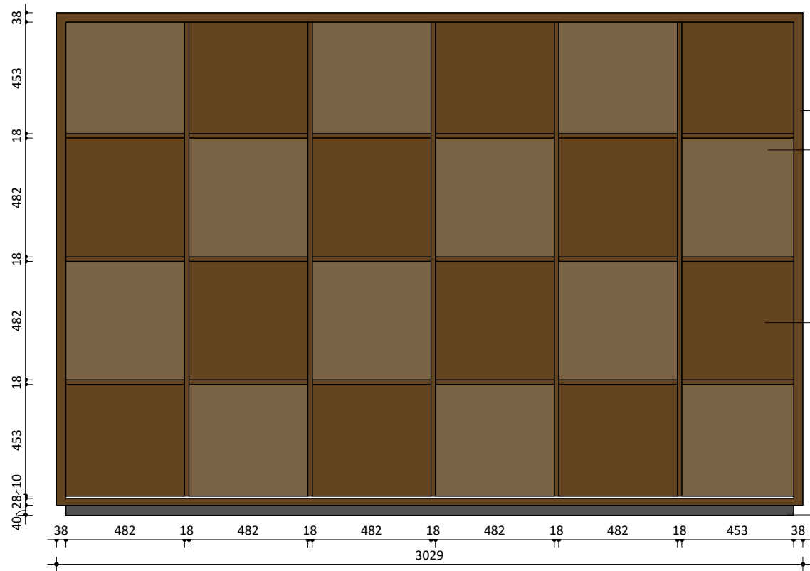
Vooraanzicht
