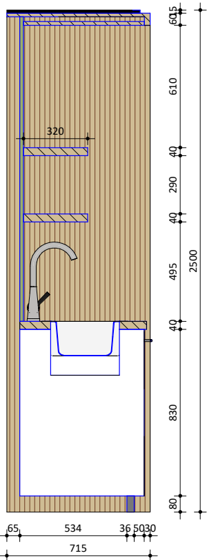
Doorsnede
