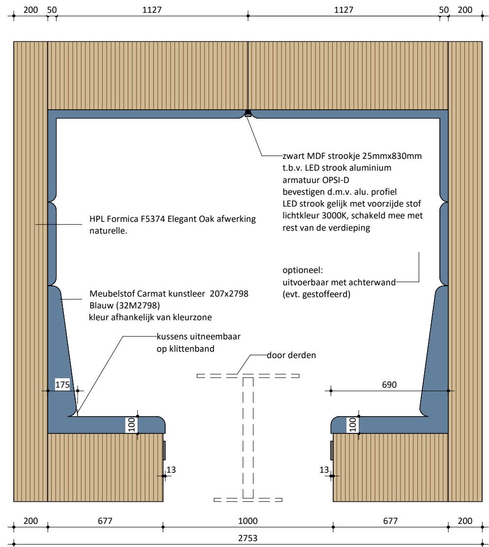
Vooraanzicht
