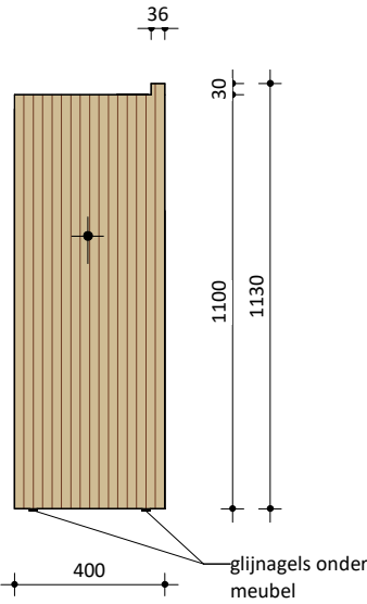
Rechter zijaanzicht
