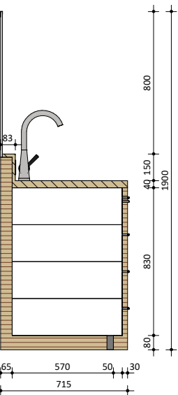
Doorsnede
