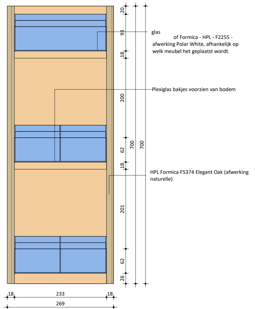
Vooraanzicht
