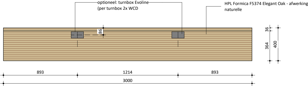
Bovenaanzicht
