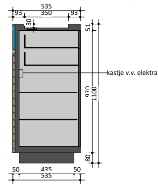
Doorsnede A
