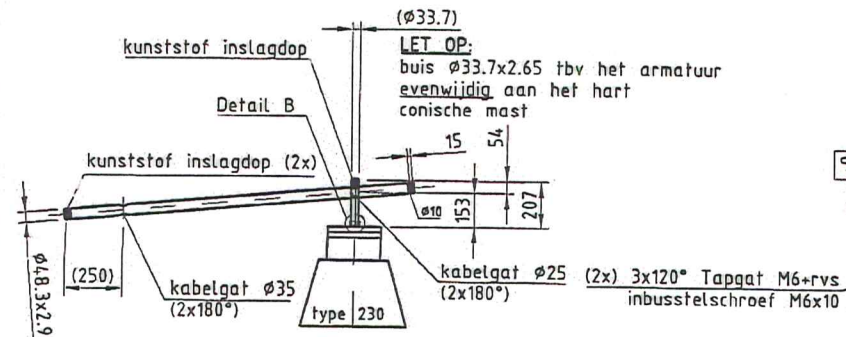
DETAIL UITLEGGER
