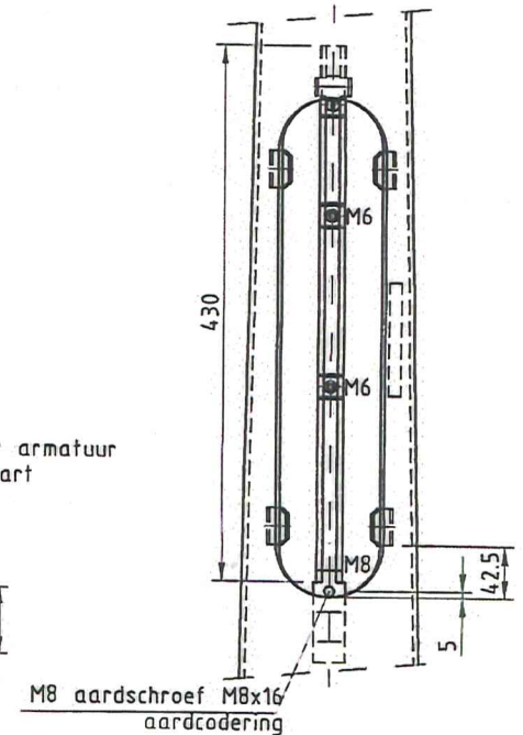
DETAIL BINNENWERK
