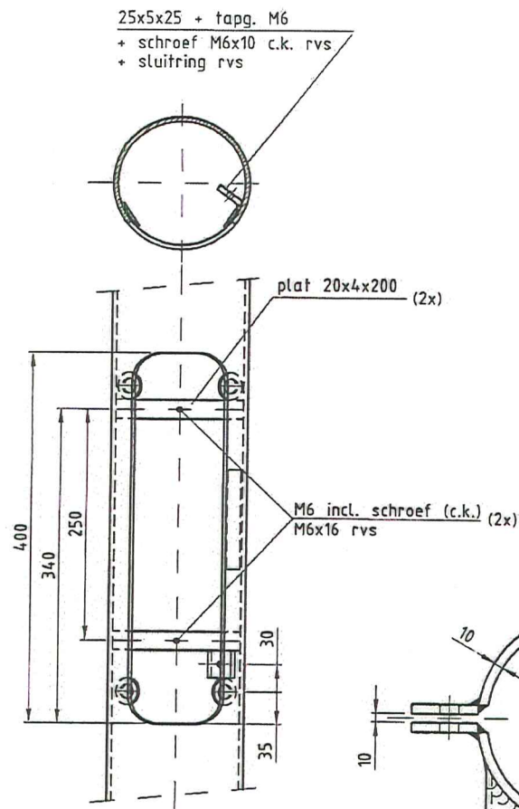
DETAIL BINNENWERK
