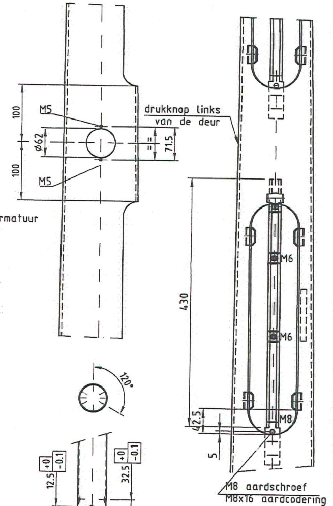
DETAIL BINNENWERK
