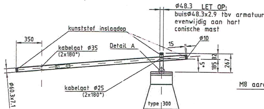
DETAIL UITLEGGER
