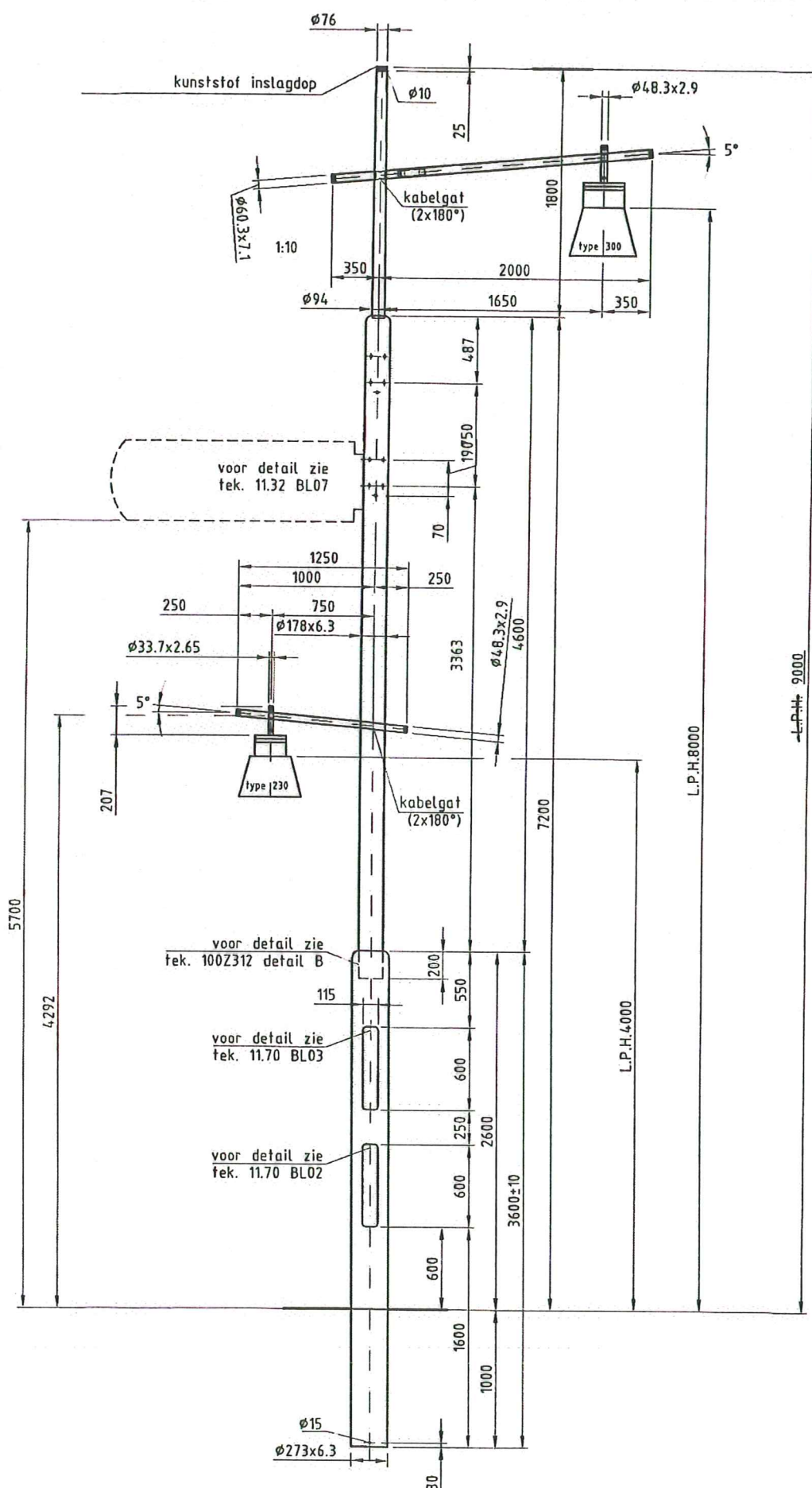
DETAIL VERLOOP
