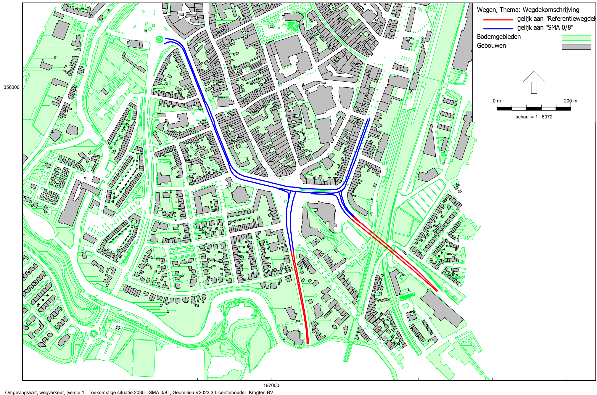
Figuur 20: Grafische weergave rekenmodel wegdektype variant bronmaatregel SMA 0/8
