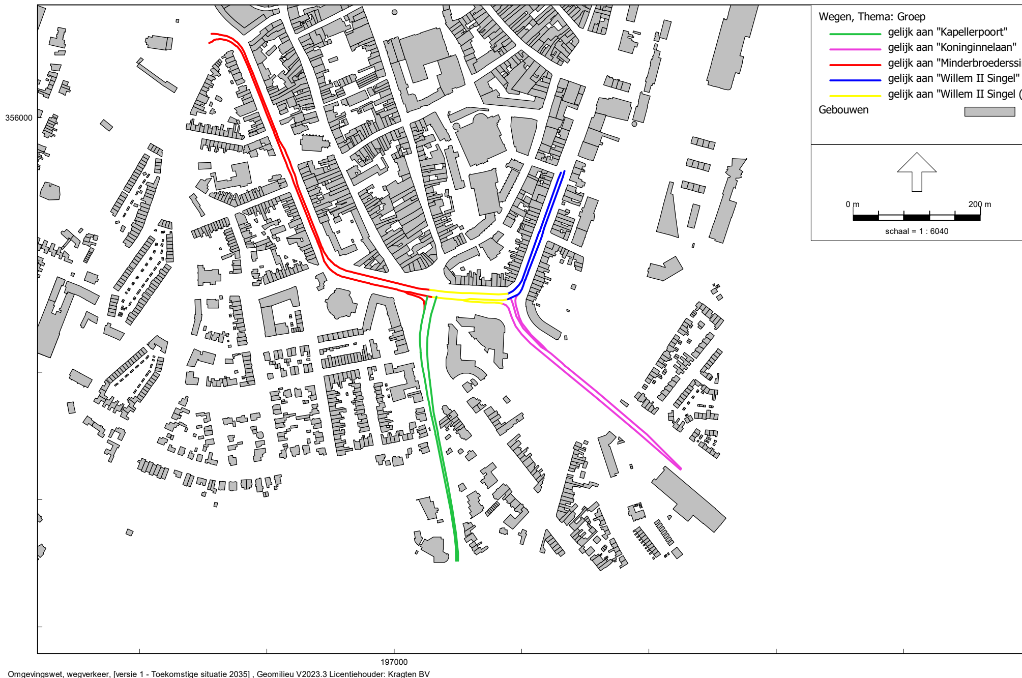
Figuur 22: Grafische weergave rekenmodel wegvakken
