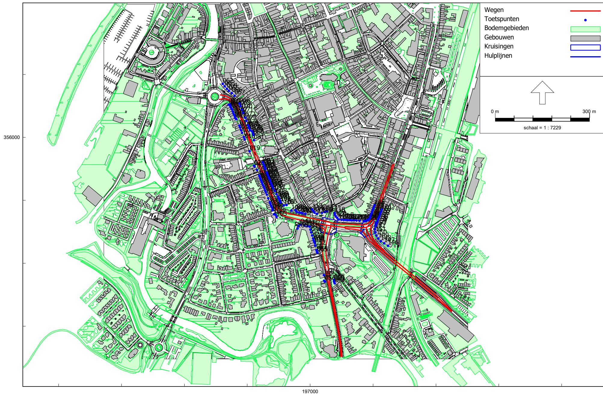
Figuur 1: Grafische weergave rekenmodel huidige situatie 2024
