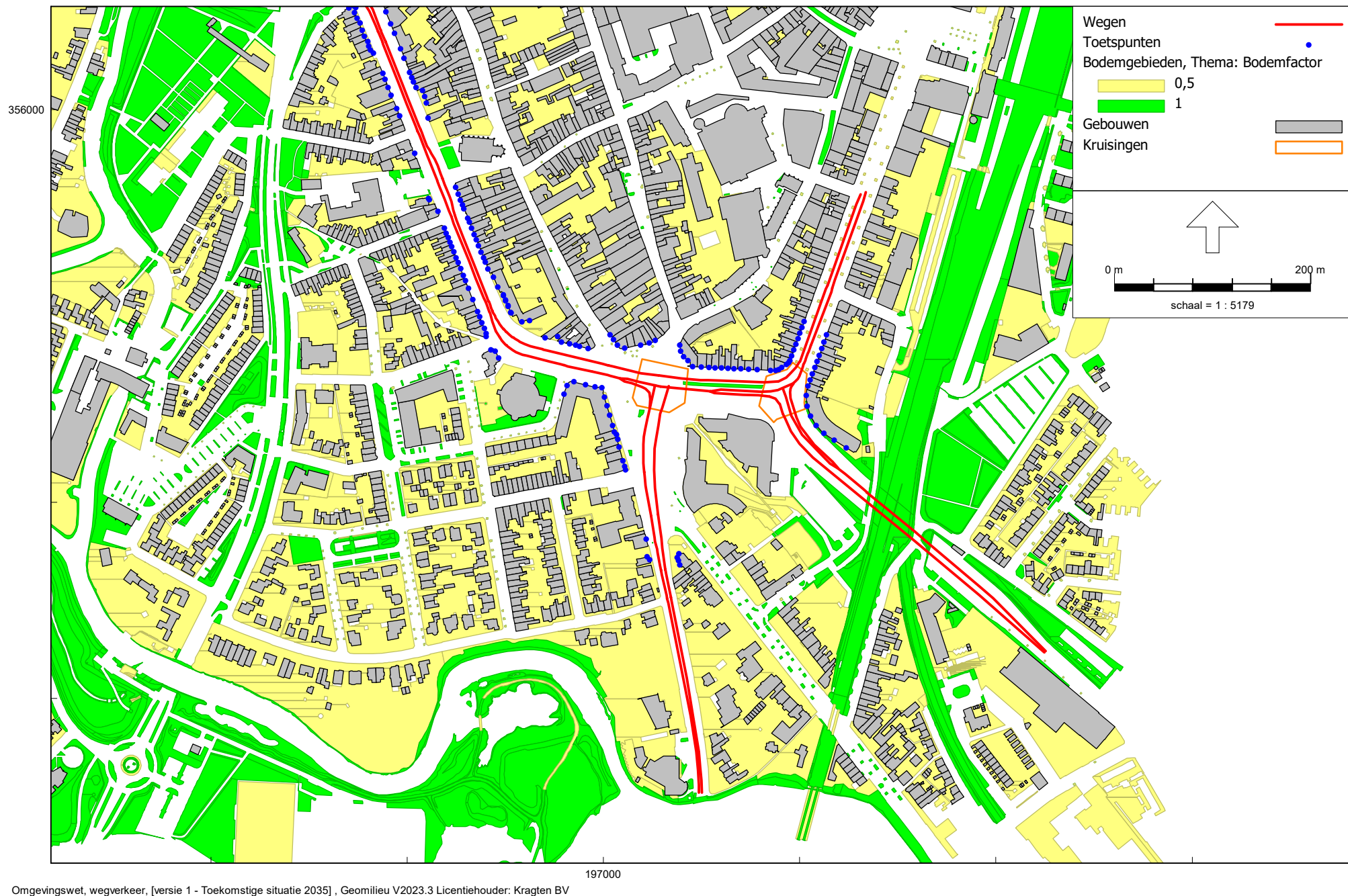
Figuur 17: Grafische weergave rekenmodel bodemgebieden toekomstige situatie 2035
