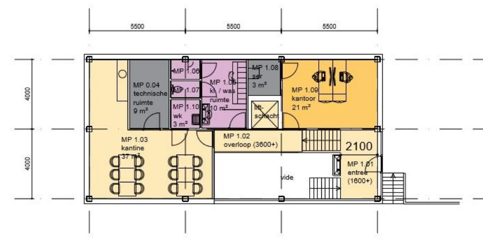
MP - verdieping 112 m² bvo
