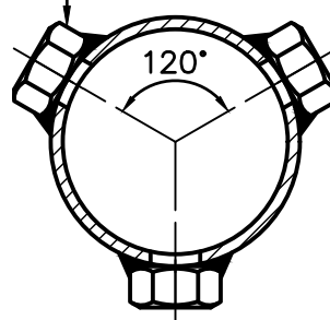
A-A (1:2)
