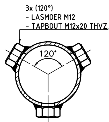
A-A (1:2)
