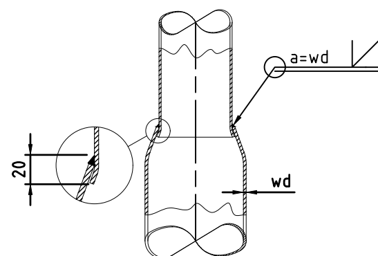
DETAIL VERLOOP
