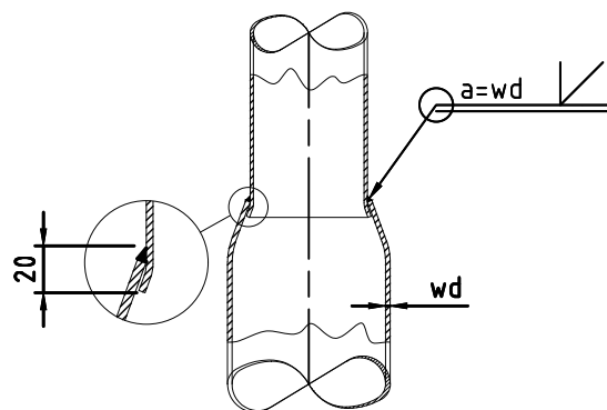
DETAIL VERLOOP
