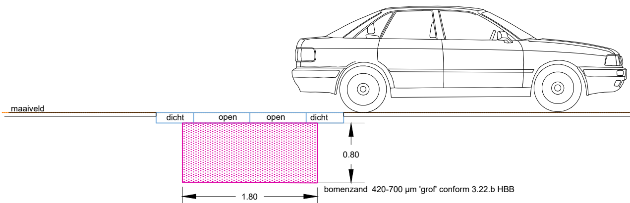
Profiel 2 schaal 1:50 Parkeren middenberm Parkeren bestaande tegels 300x300 nieuwe verharding SoliDrain 125-50x62,5 bestaande tegels 300x300
