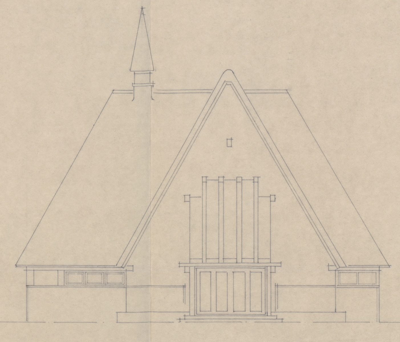
ZIJGEVEL
