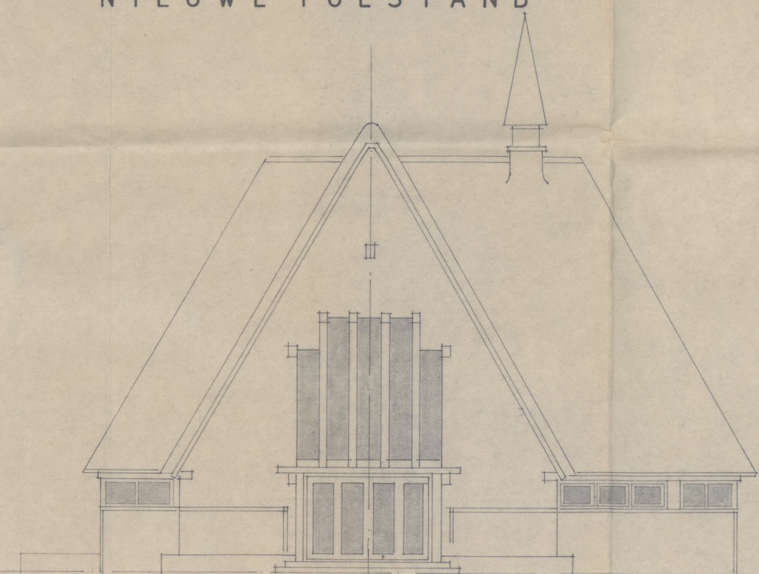
ZIJGEVEL
