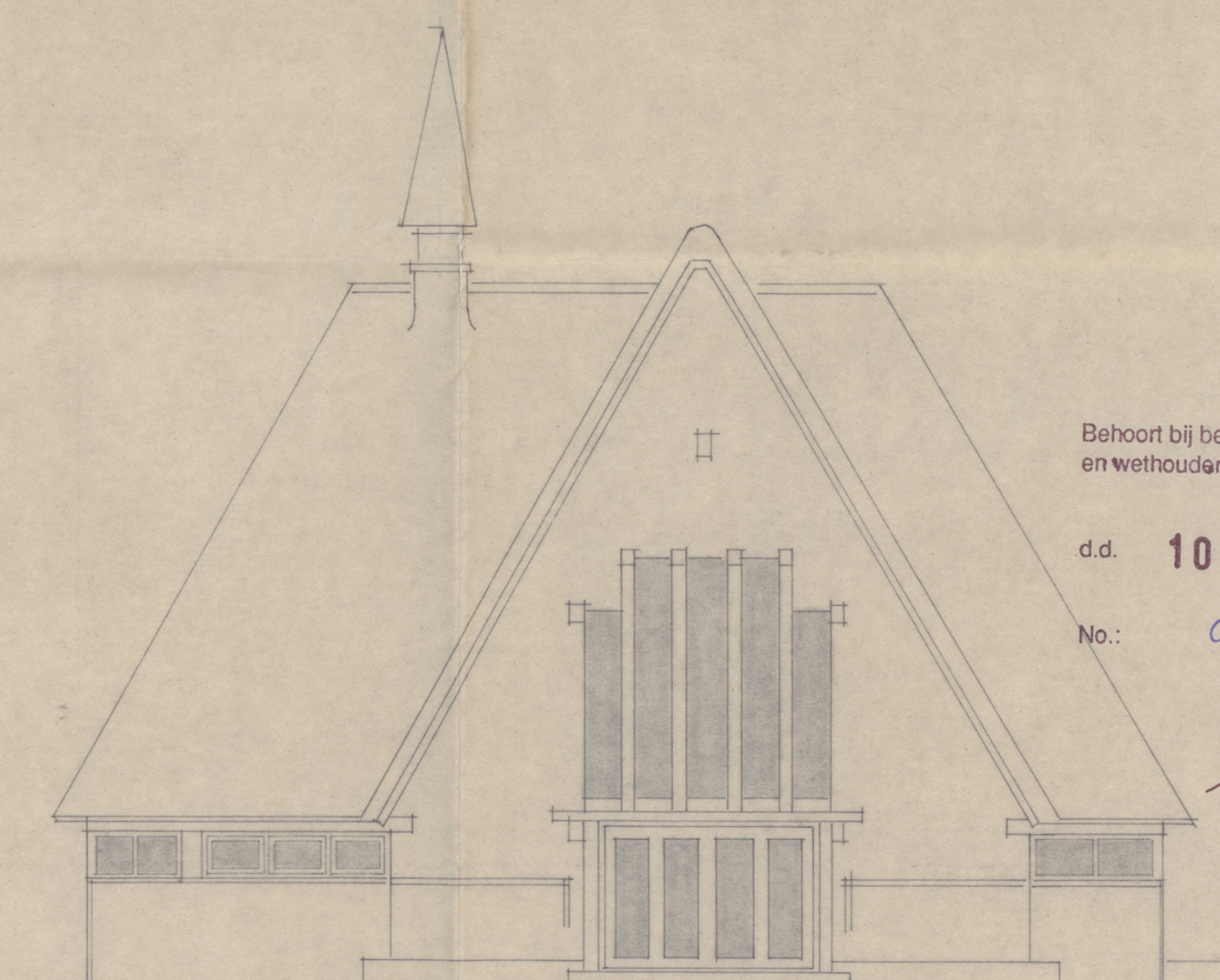
ZIJGEVEL
