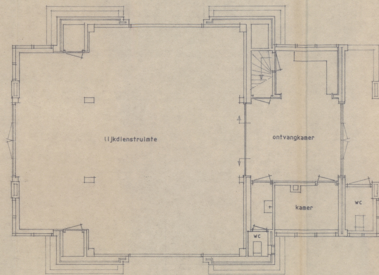
PLATTEGROND
