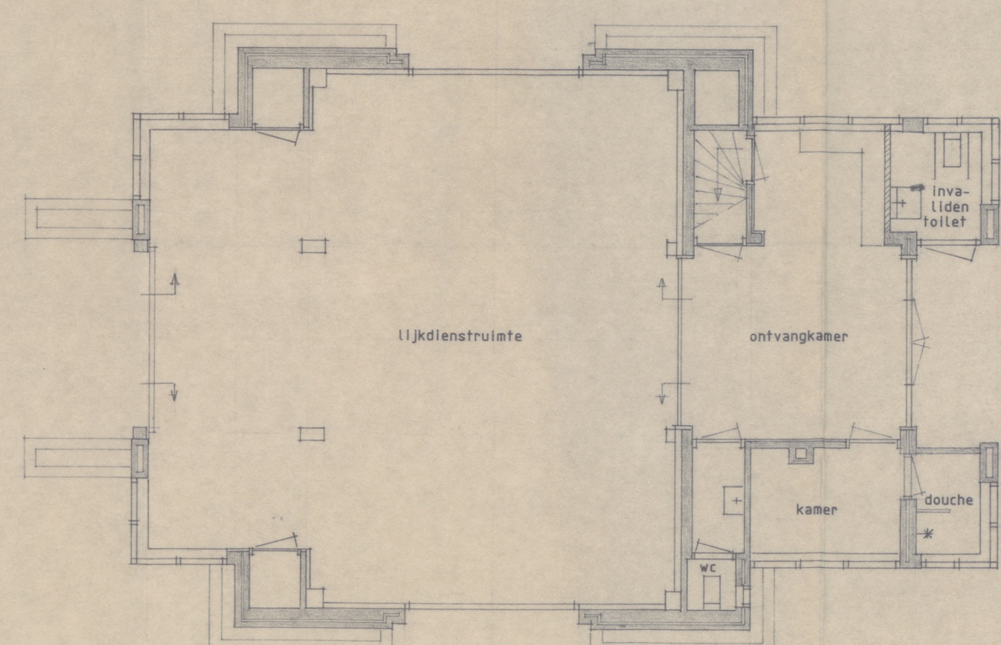
PLATTEGROND
