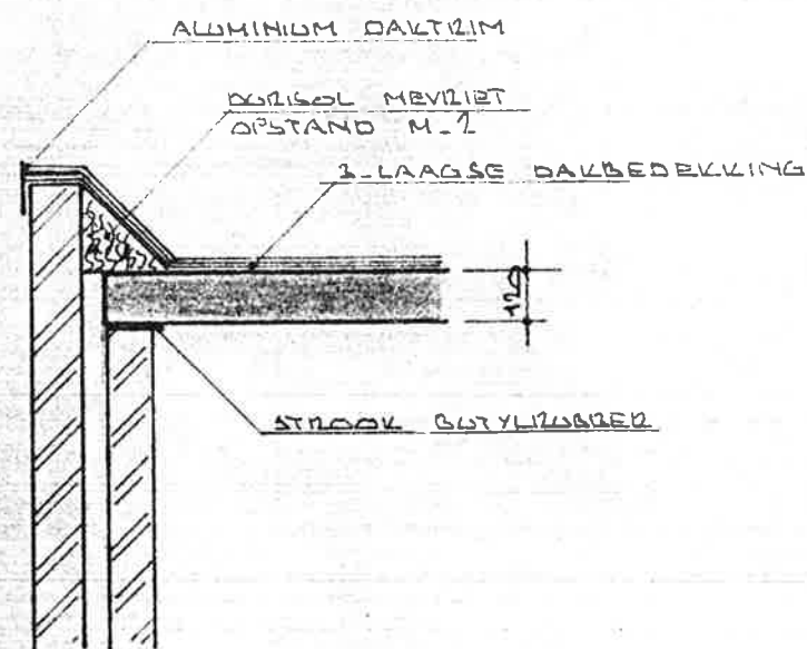
DOORSNEDE B-B
