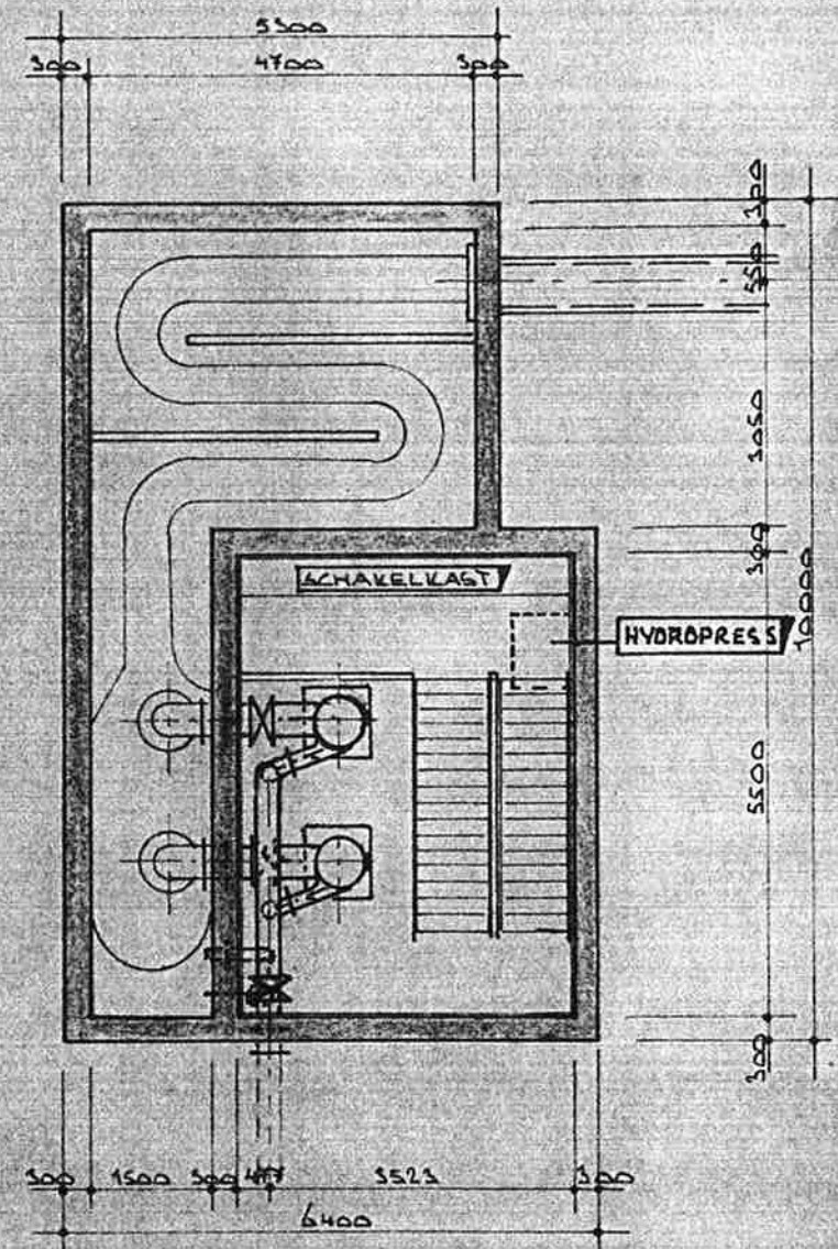
HORIZONTALE DOORSNEDE
