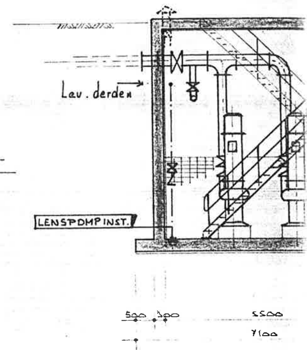
DOORSNEDE
