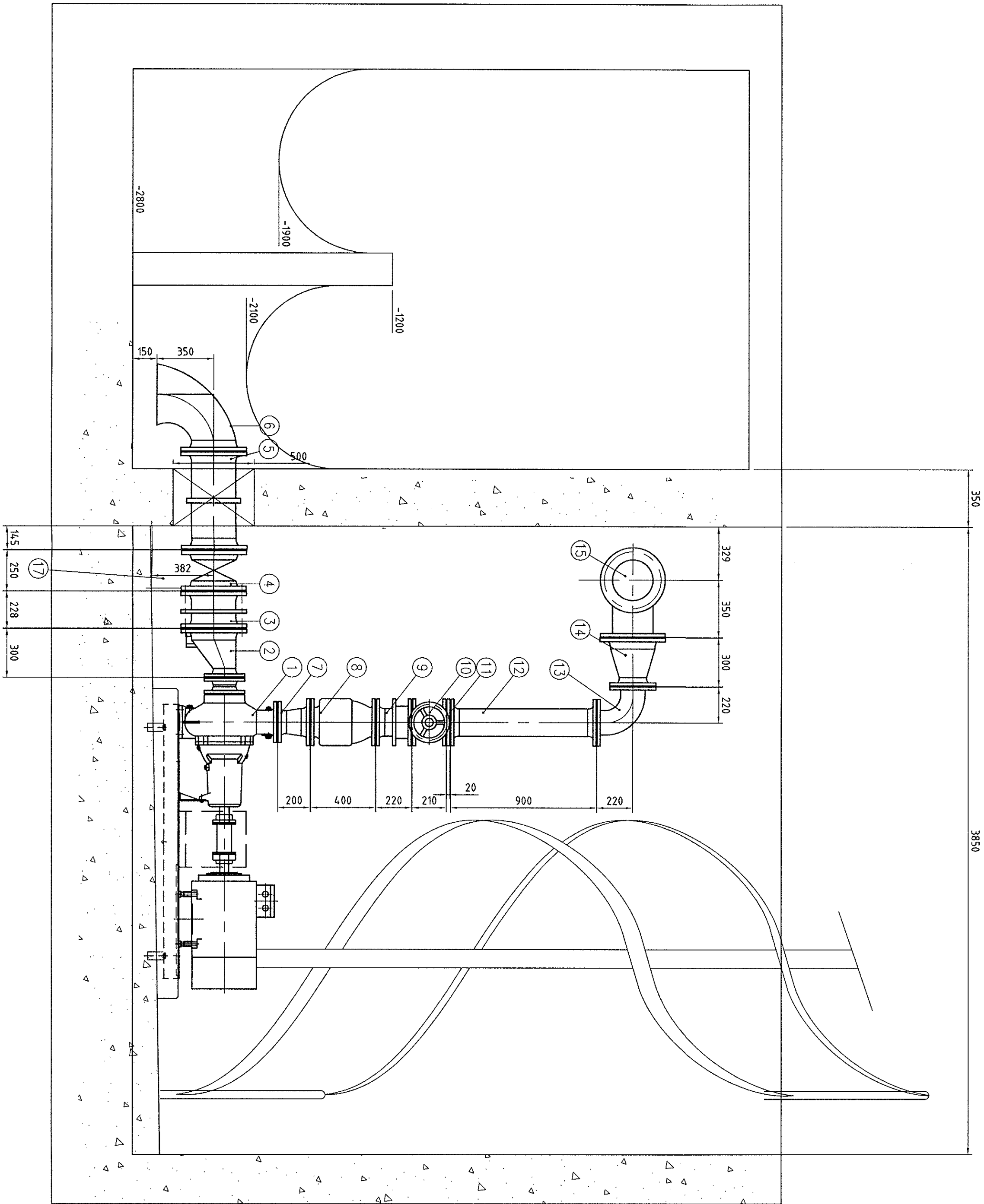
DOORSNEDE B-B
