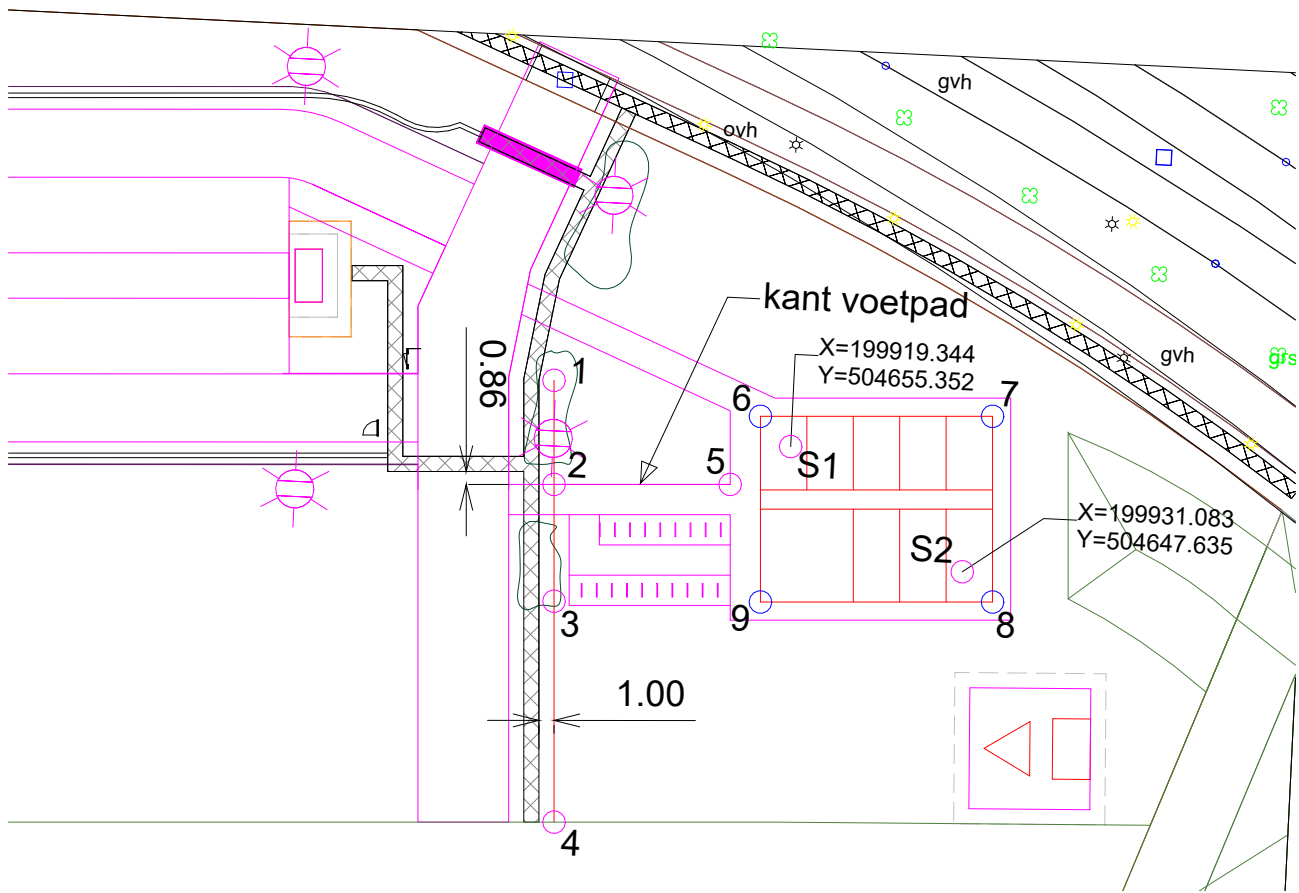
Situatie 1:500
