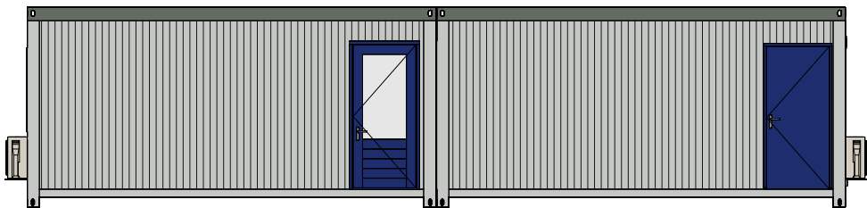
Linkerzijaanzicht 1:100
