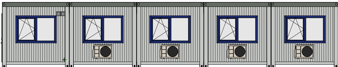
Vooraanzicht 1:100
