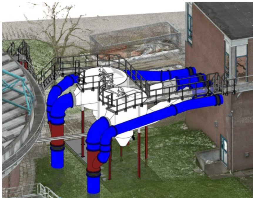
Figuur 2 3D aanzicht van de nieuwe zandvangers tussen het roostergoedgebouw en voorbezinktank 2
