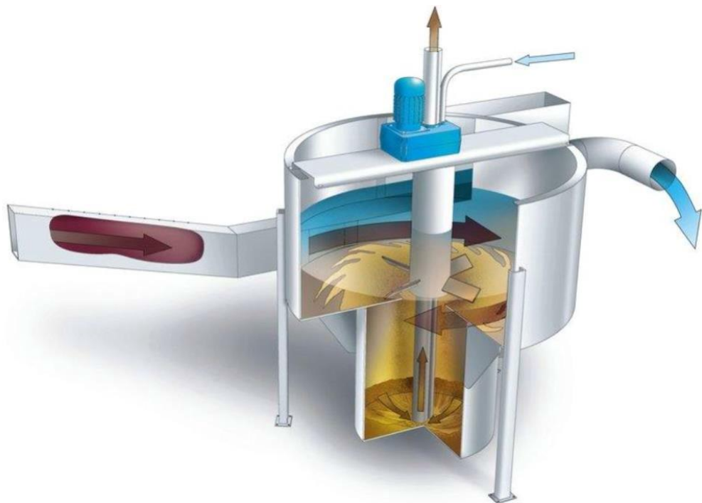
Figuur 1 3D weergave van een Vortex zandvanger
