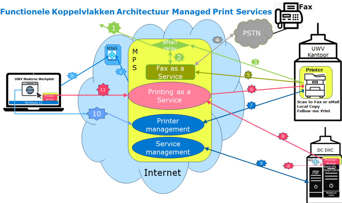
Figuur 2: Functionele koppelvlakken architectuur Managed Print Services
