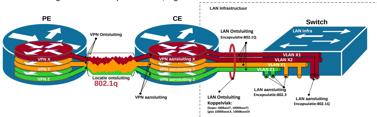
Figuur 42: LAN infrastructuur ODC
