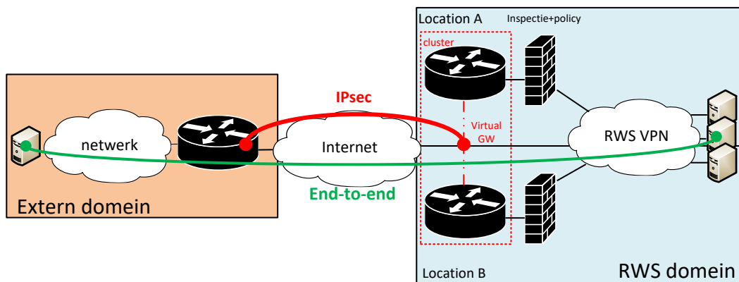
Figuur 35 - IPsec
