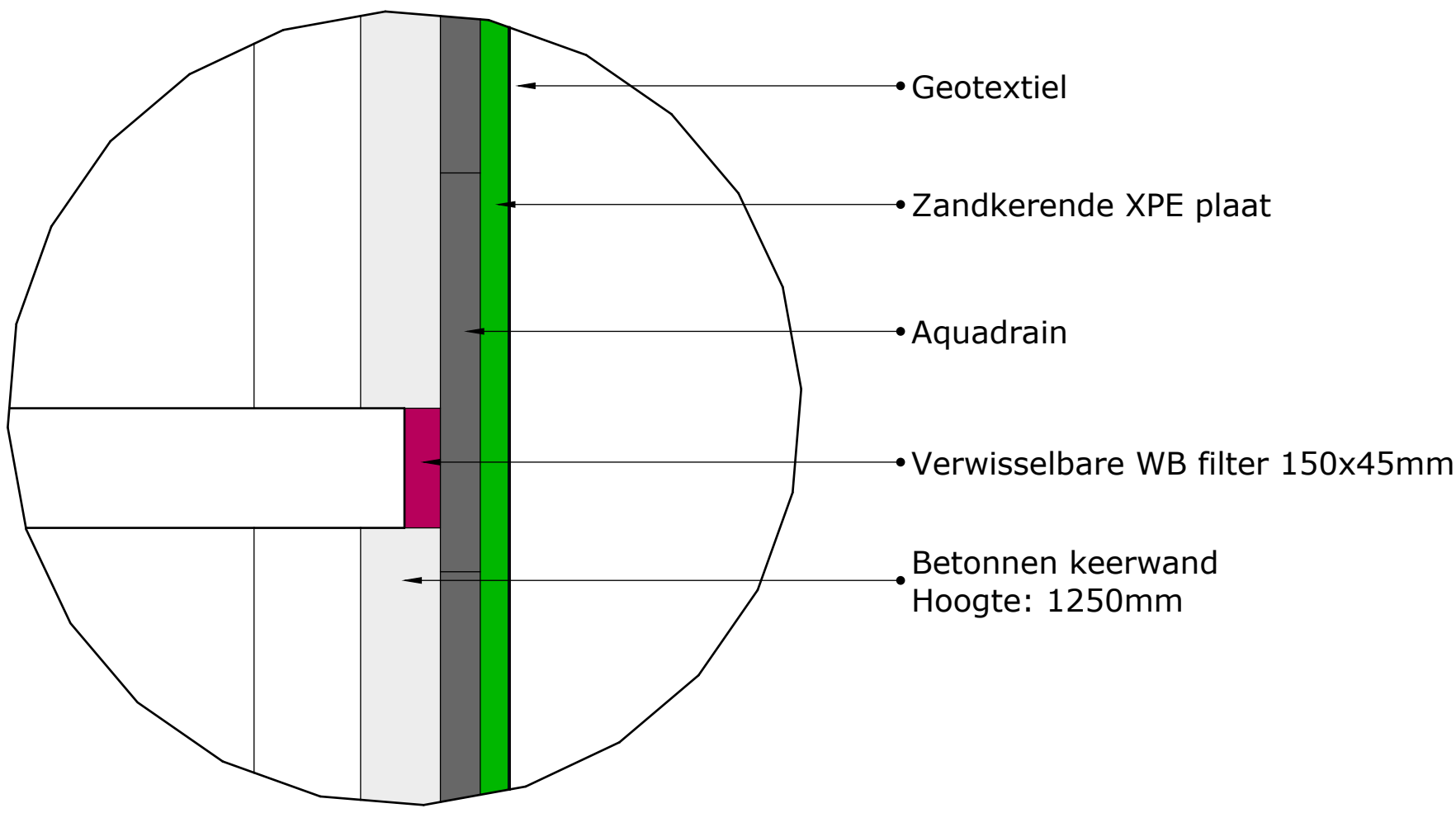
Detail afbeelding
