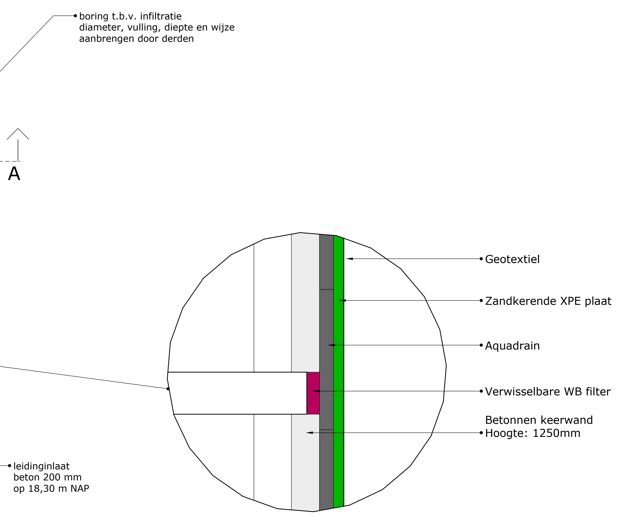
DETAIL-AFBEELDING
