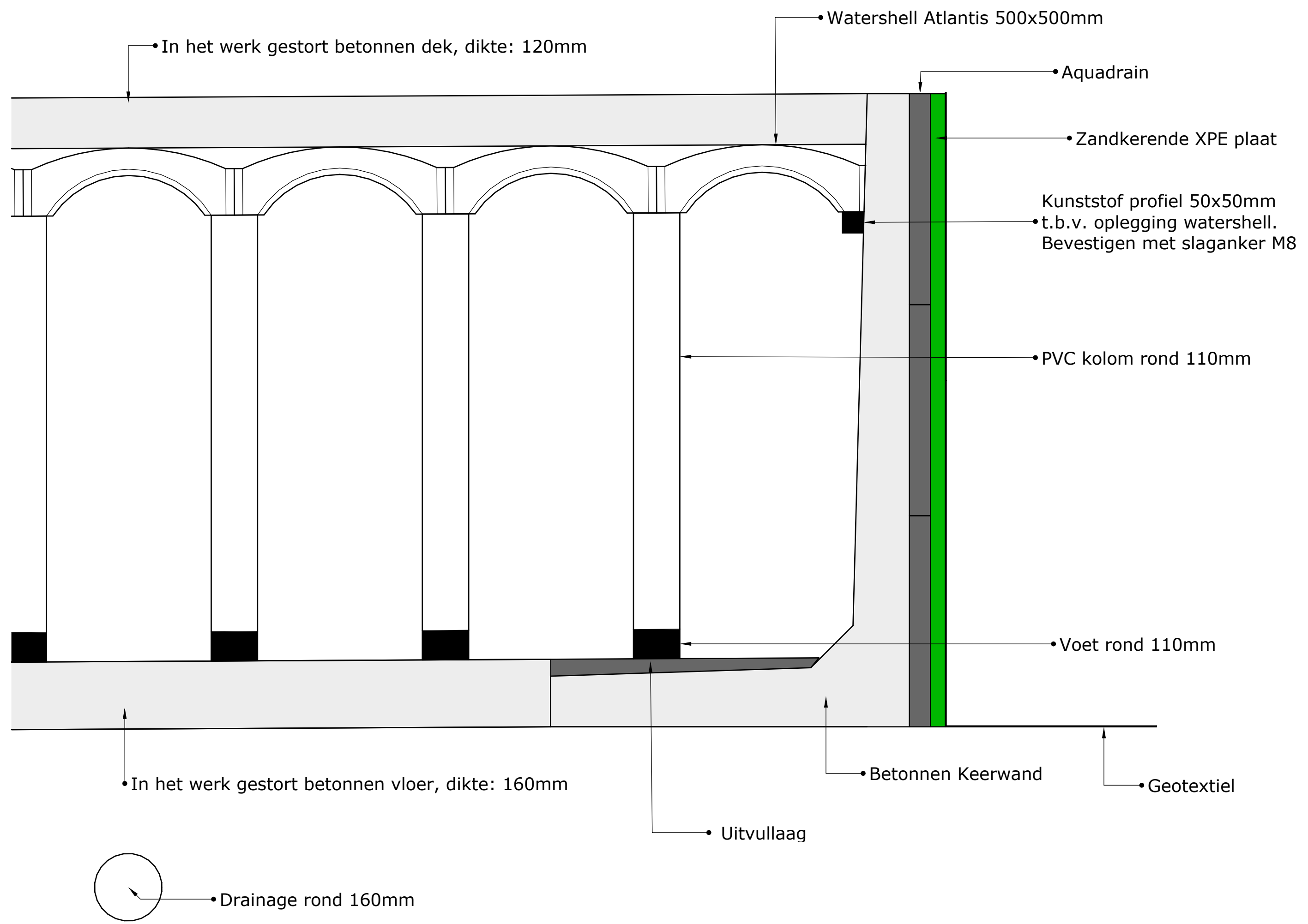
DETAIL-AFBEELDING
