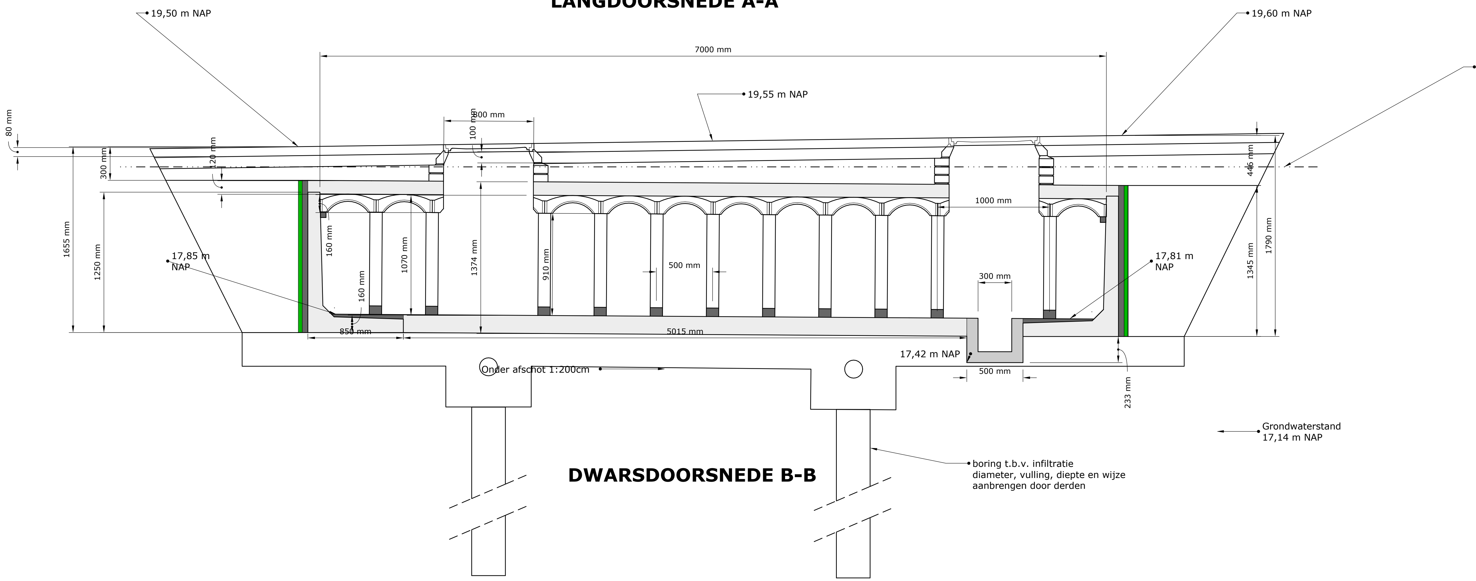
LANGDOORSNEDE A-A
