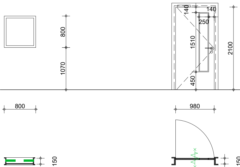
BI 2.03 Binnenkozijn met vast glas Aantal: 1 stuks
