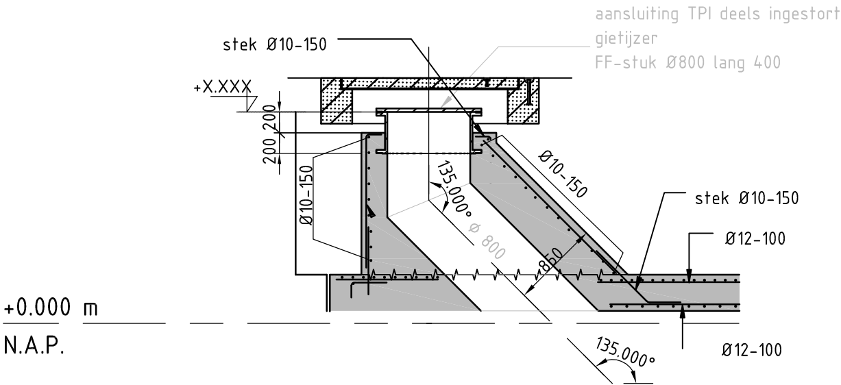
DOORSNEDE schaal: 1:50
