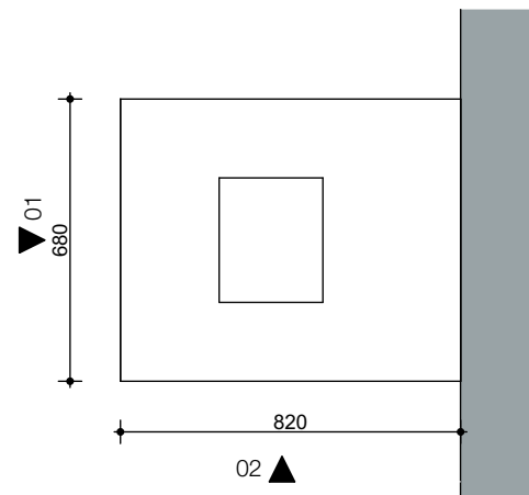
Bovenaanzicht
