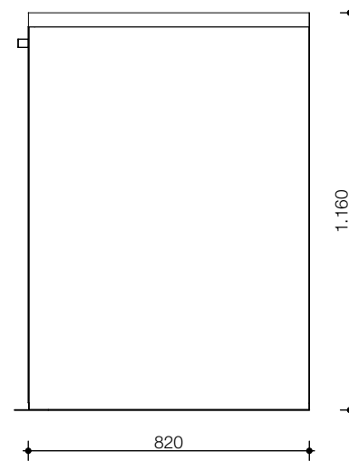
Aanzicht 02
