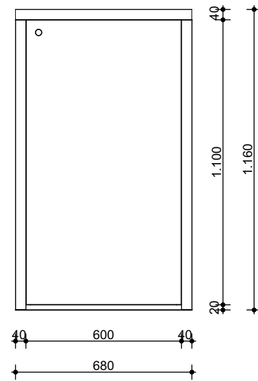
Aanzicht 01
