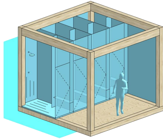
Douchegroep met 4 douche-/kleedhokjes +/- 16m 2
