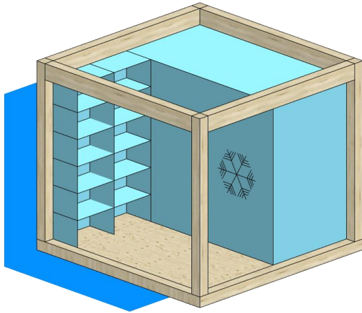
Koelcel met koel/vries/fust +/- 16m 2
